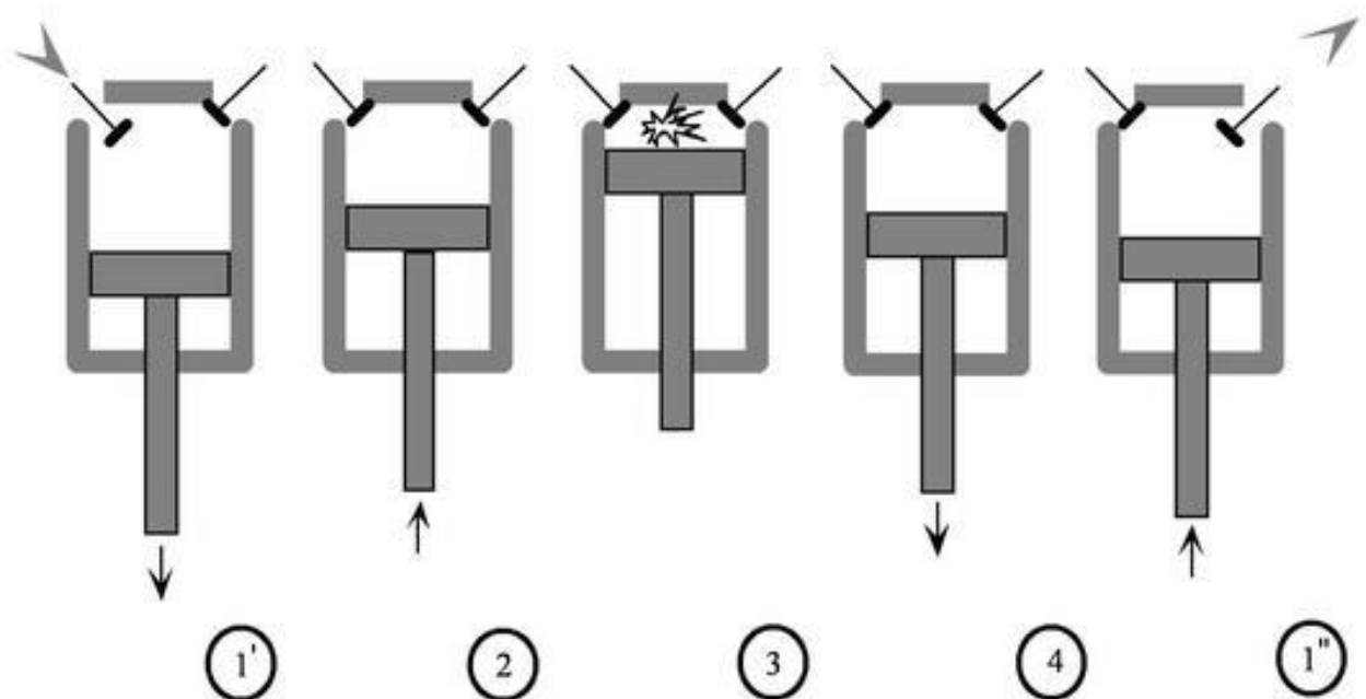
Рис. 2.5. Поршень і клапани в чотиритактному двигуні внутрішнього згорання
