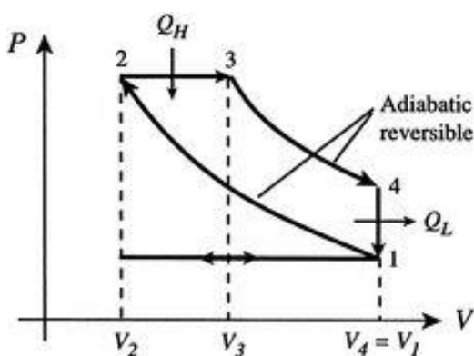
Рис. 2.4. Цикл Дизеля
