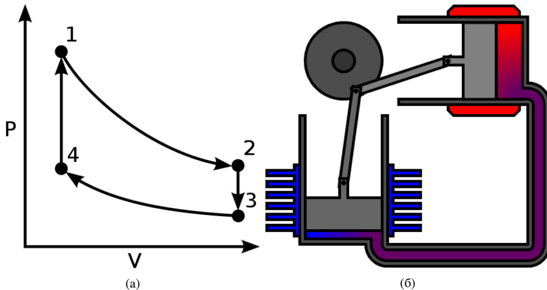
Рис. 1.13. Цикл (а) та Двигун (б) Стирлінга
