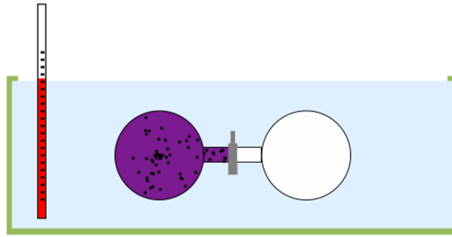
Рис. 1.5. Дослід Гей-Люсака по розширенню газу в вакуум
