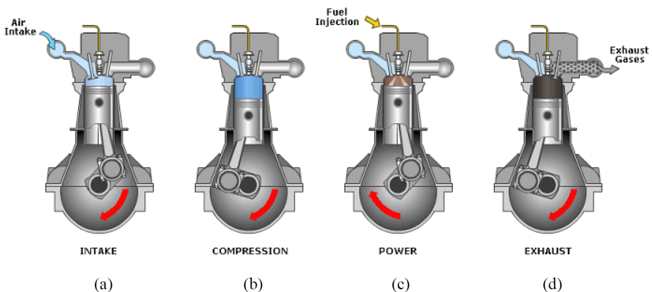
Рис. 1.12. Цикл роботи дизельного двигуна
