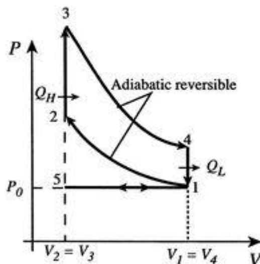
Рис. 1.9. Цикл Отто роботи бензинового двигуна
