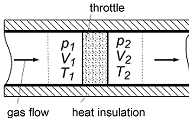
Рис. 1.6. Протікання газу через пористу перегородку в тепло-ізольованій трубці
