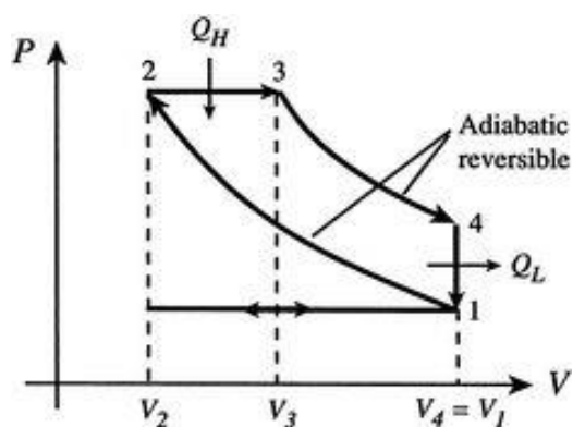
Рис. 1.10. Цикл Дизеля
