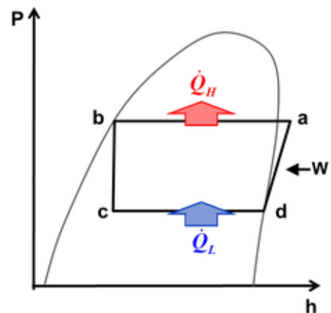
Рис. 1.14. Цикл роботи теплового насоса
