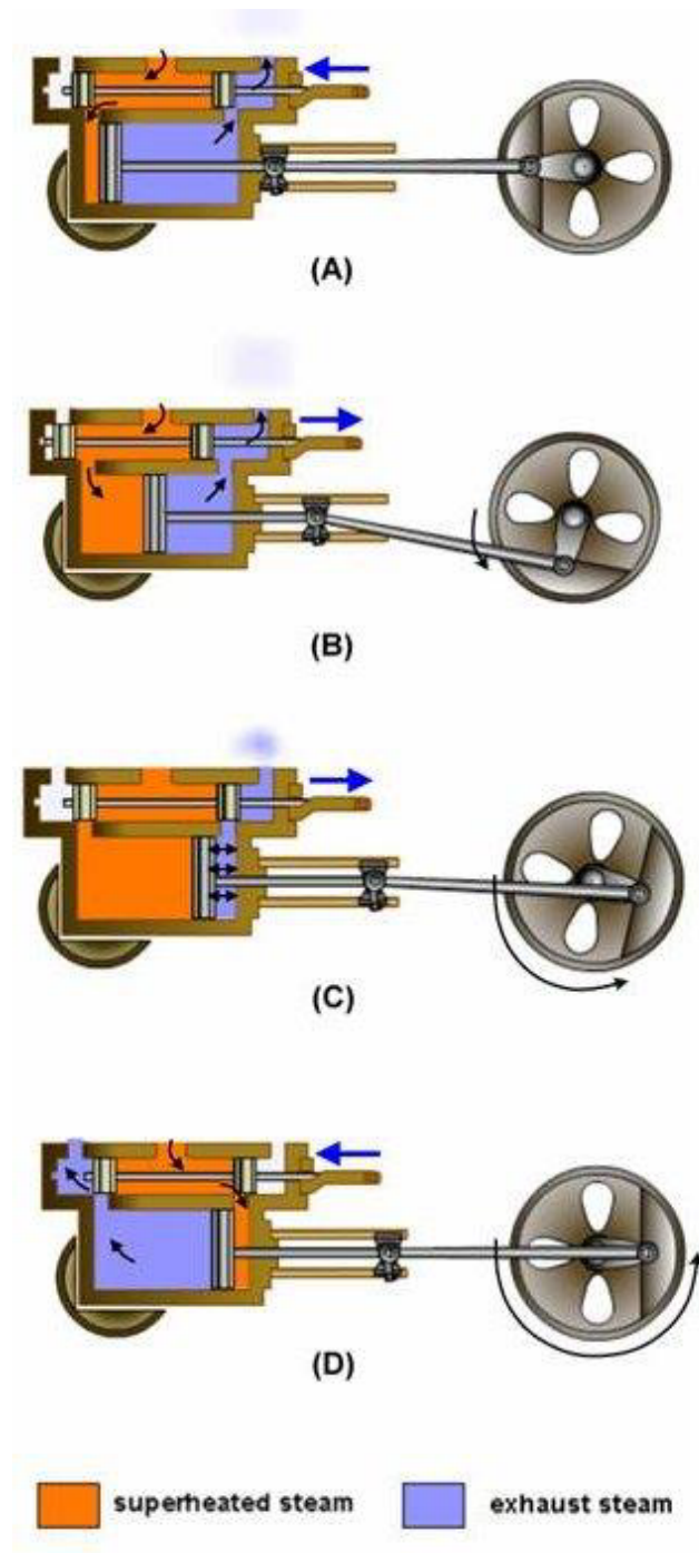
Рис. 1.8. Робота двотактної парової машини.
