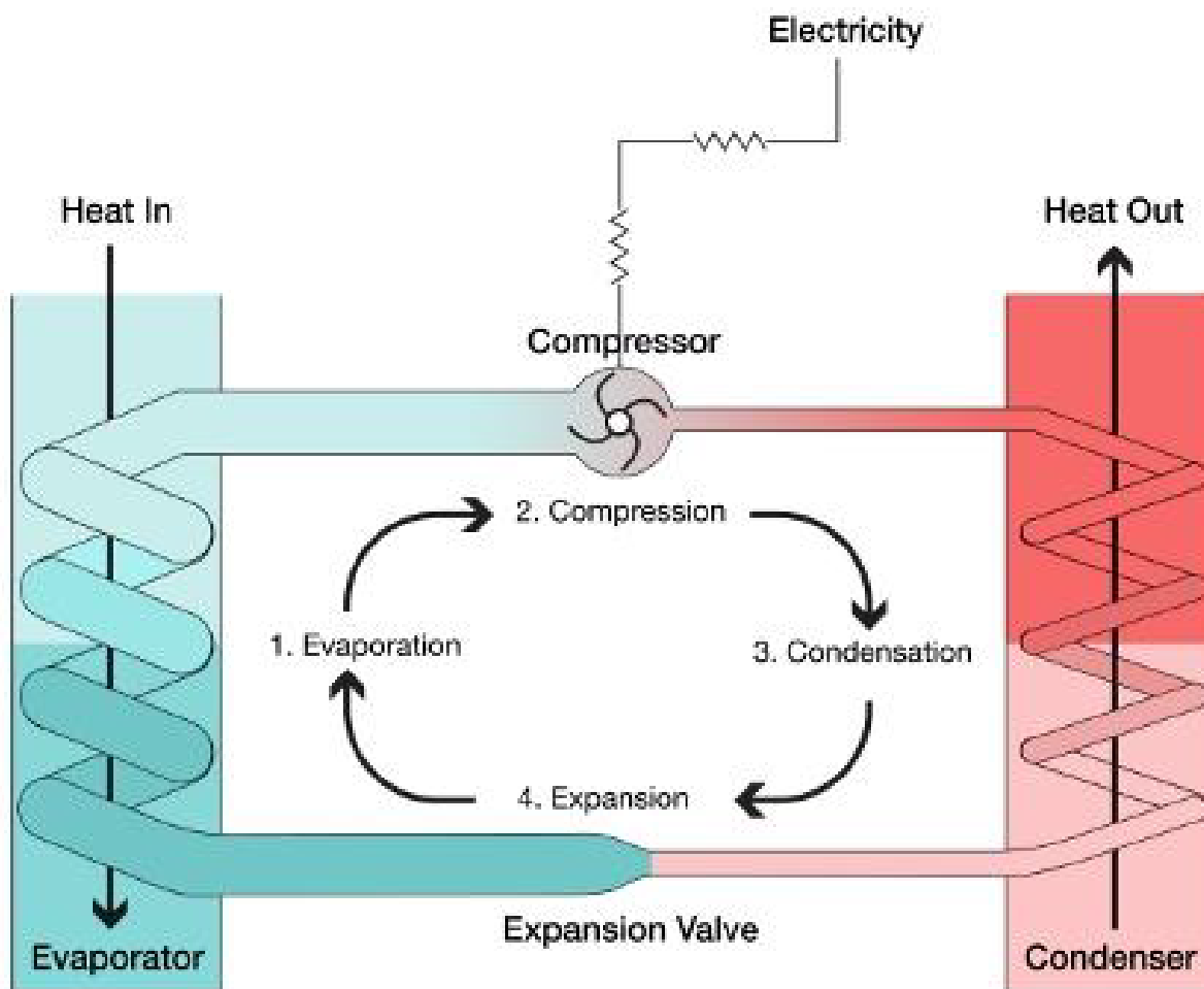
Рис. 1.15. Схема роботи теплового насосу
