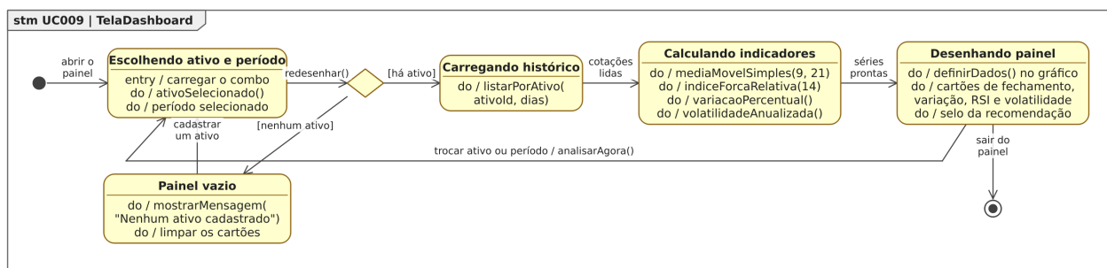
Figura 74: Figura 74. Diagrama de Estados da classe TelaDashboard para o [UC009].
