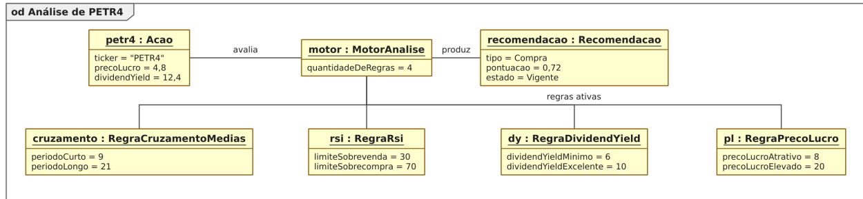
Figura 18: Figura 18. Diagrama de objetos da análise de um ativo.
