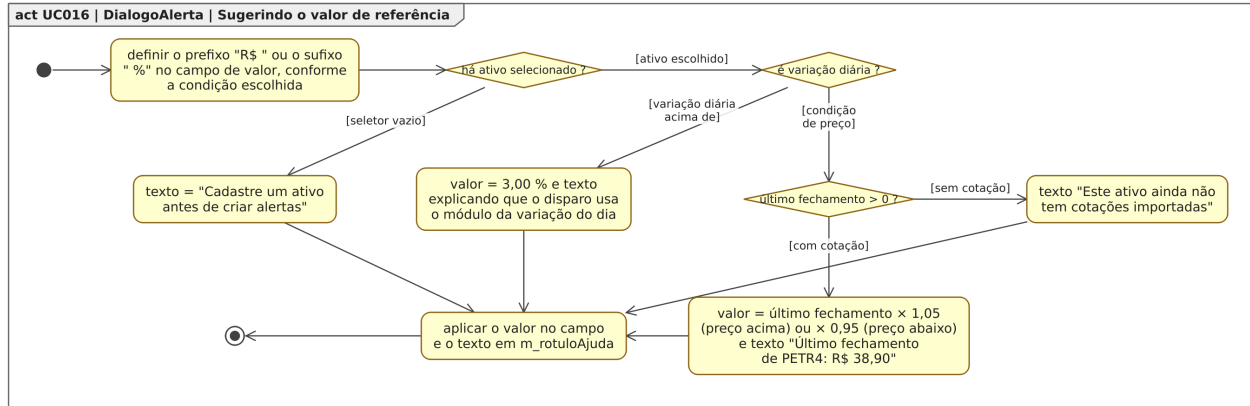
Figura 130: Figura 130. Diagrama de Atividades para o estado “Sugerindo o valor de referência”, dentro do Diagrama de Estados para a classe DialogoAlerta em [UC016].
