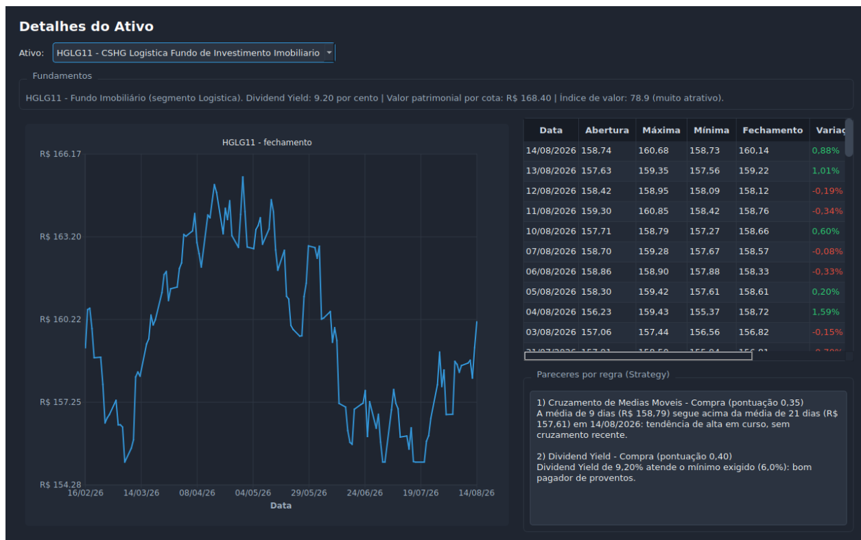
Figura 6: Tela de detalhes do ativo, com fundamentos, histórico e reavaliação regra a regra.
