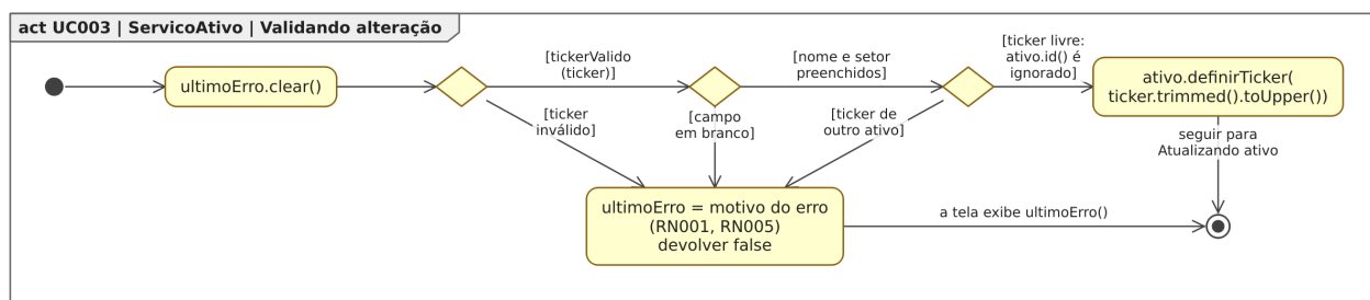
Figura 102: Figura 102. Diagrama de Atividades para o estado “Validando alteração”, dentro do Diagrama de Estados para a classe ServicoAtivo em [UC003].
