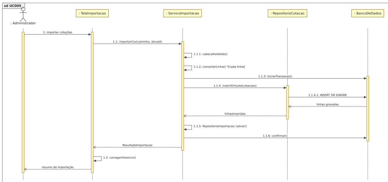
Figura 24: Figura 24. Diagrama de sequência para o [UC005].
