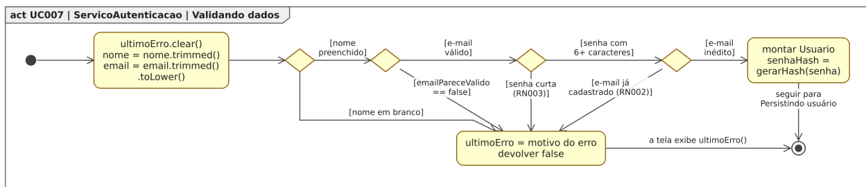
Figura 111: Figura 111. Diagrama de Atividades para o estado “Validando dados”, dentro do Diagrama de Estados para a classe ServicoAutenticacao em [UC007].
