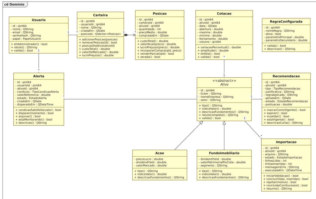
Figura 15: Figura 15. Diagrama de classes do domínio do sistema.
