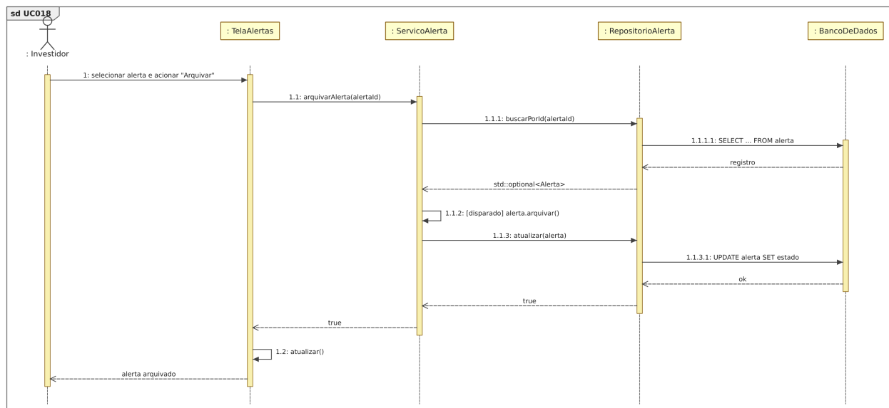
Figura 37: Figura 37. Diagrama de sequência para o [UC018].
