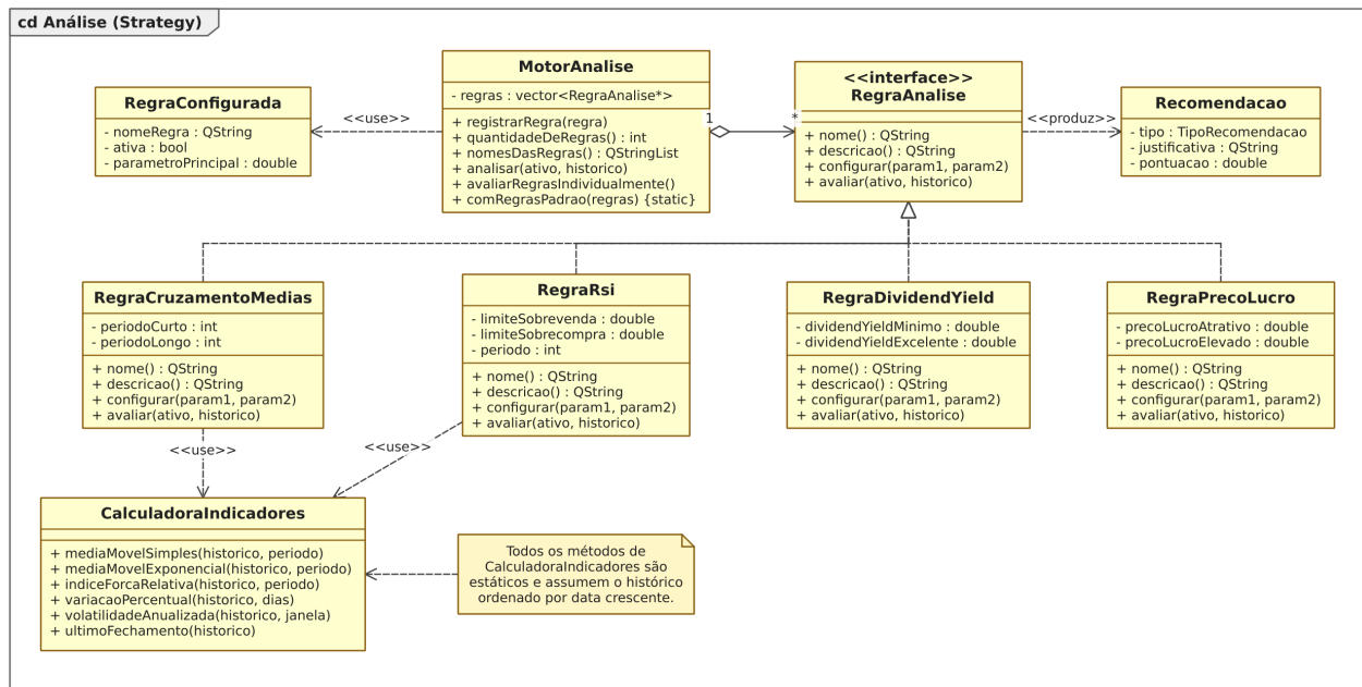
Figura 16: Figura 16. Diagrama de classes do núcleo de análise, com o padrão Strategy.
