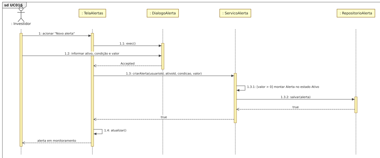
Figura 35: Figura 35. Diagrama de sequência para o [UC016].
