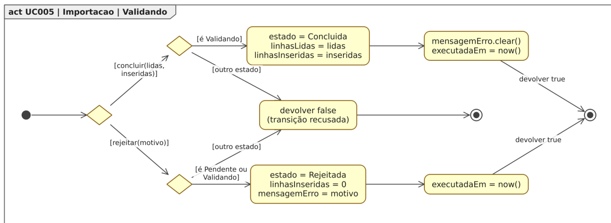
Figura 107: Figura 107. Diagrama de Atividades para o estado “Validando”, dentro do Diagrama de Estados para a classe Importacao em [UC005].
