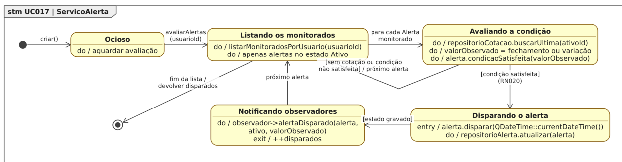
Figura 93: Figura 93. Diagrama de Estados da classe ServicoAlerta para o [UC017].
