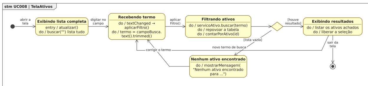
Figura 72: Figura 72. Diagrama de Estados da classe TelaAtivos para o [UC008].
