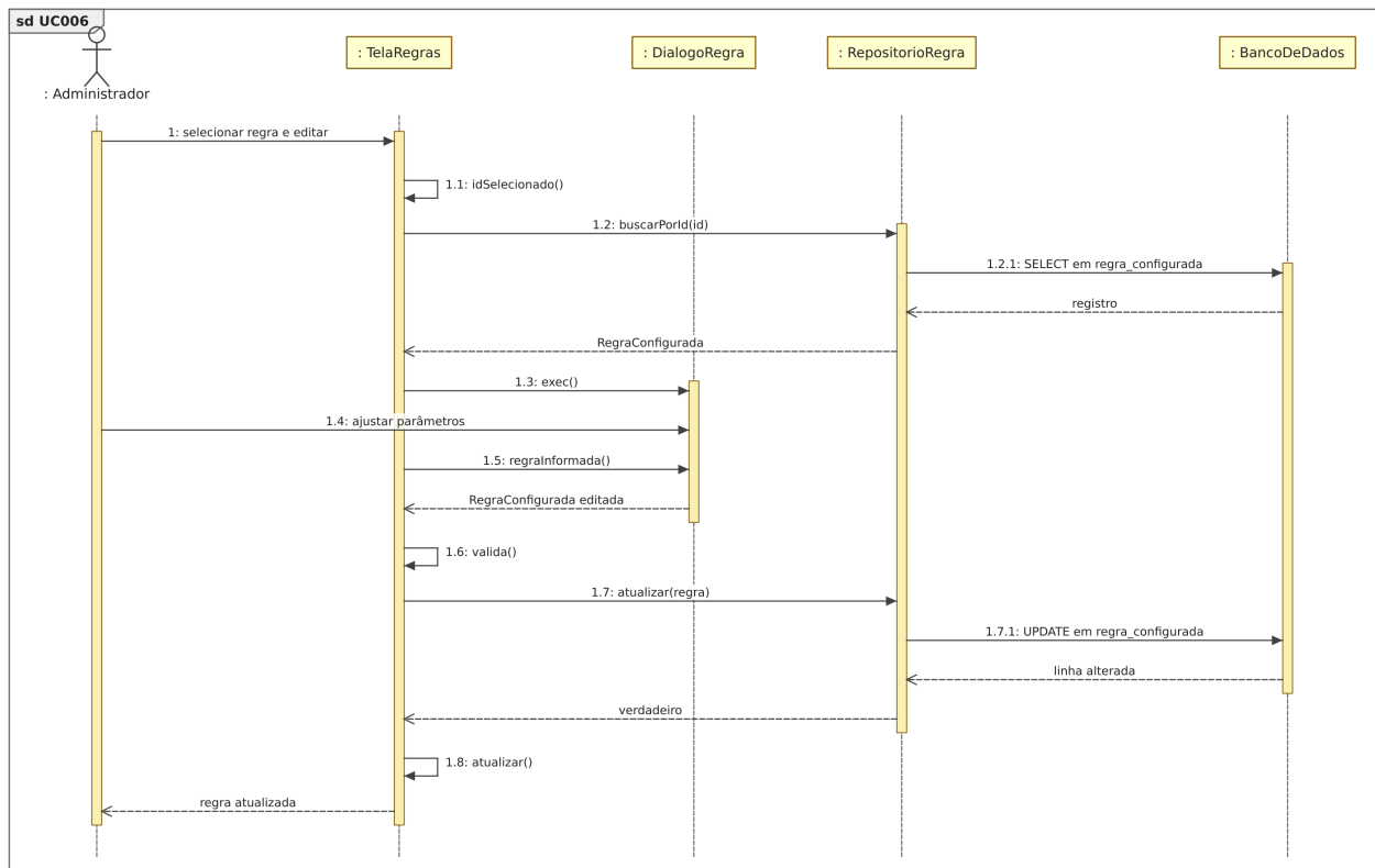
Figura 25: Figura 25. Diagrama de sequência para o [UC006].
