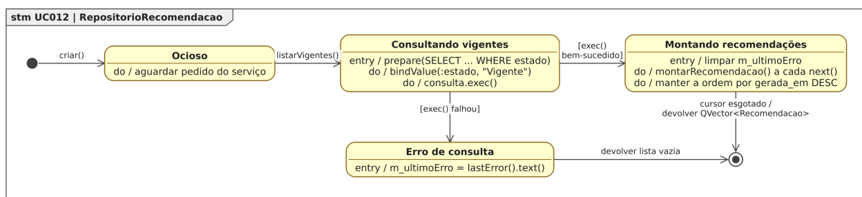
Figura 82: Figura 82. Diagrama de Estados da classe RepositorioRecomendacao para o [UC012].
