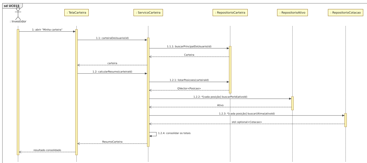
Figura 34: Figura 34. Diagrama de sequência para o [UC015].
