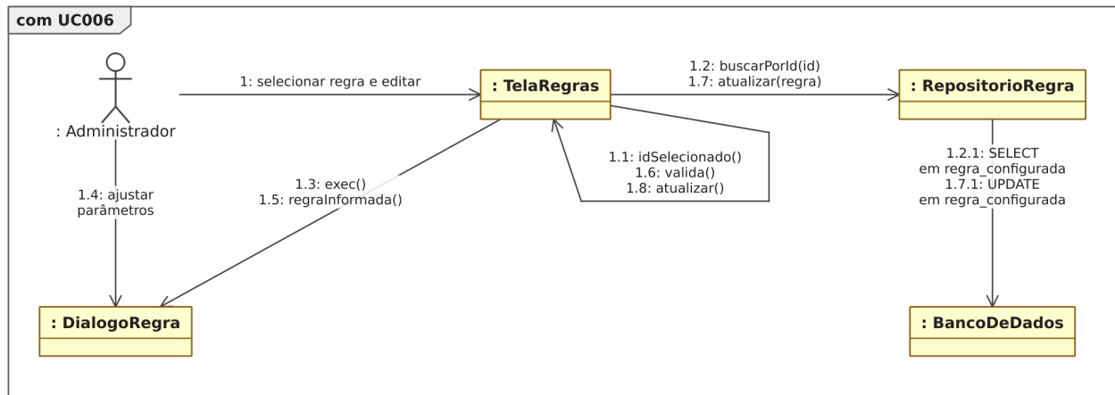
Figura 43: Figura 43. Diagrama de comunicação para o [UC006].
