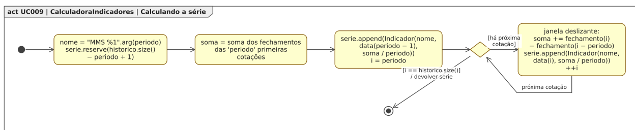
Figura 115: Figura 115. Diagrama de Atividades para o estado “Calculando a série”, dentro do Diagrama de Estados para a classe CalculadoraIndicadores em [UC009].
