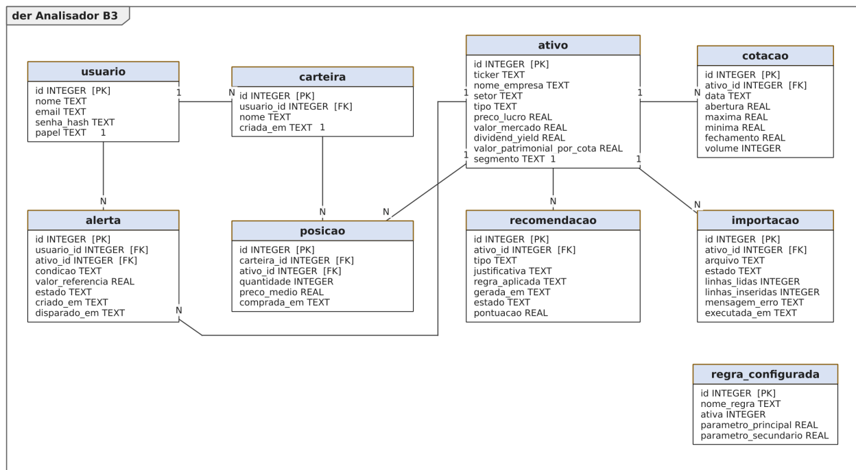
Figura 56: Figura 56. Diagrama Entidade-Relacionamento do banco de dados.
