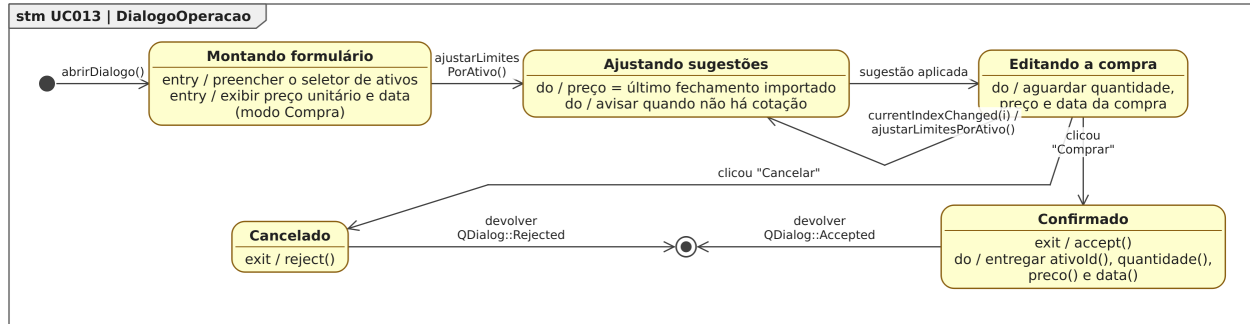
Figura 83: Figura 83. Diagrama de Estados da classe DialogoOperacao para o [UC013].
