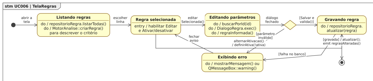
Figura 68: Figura 68. Diagrama de Estados da classe TelaRegras para o [UC006].
