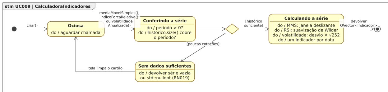
Figura 75: Figura 75. Diagrama de Estados da classe CalculadoraIndicadores para o [UC009].
