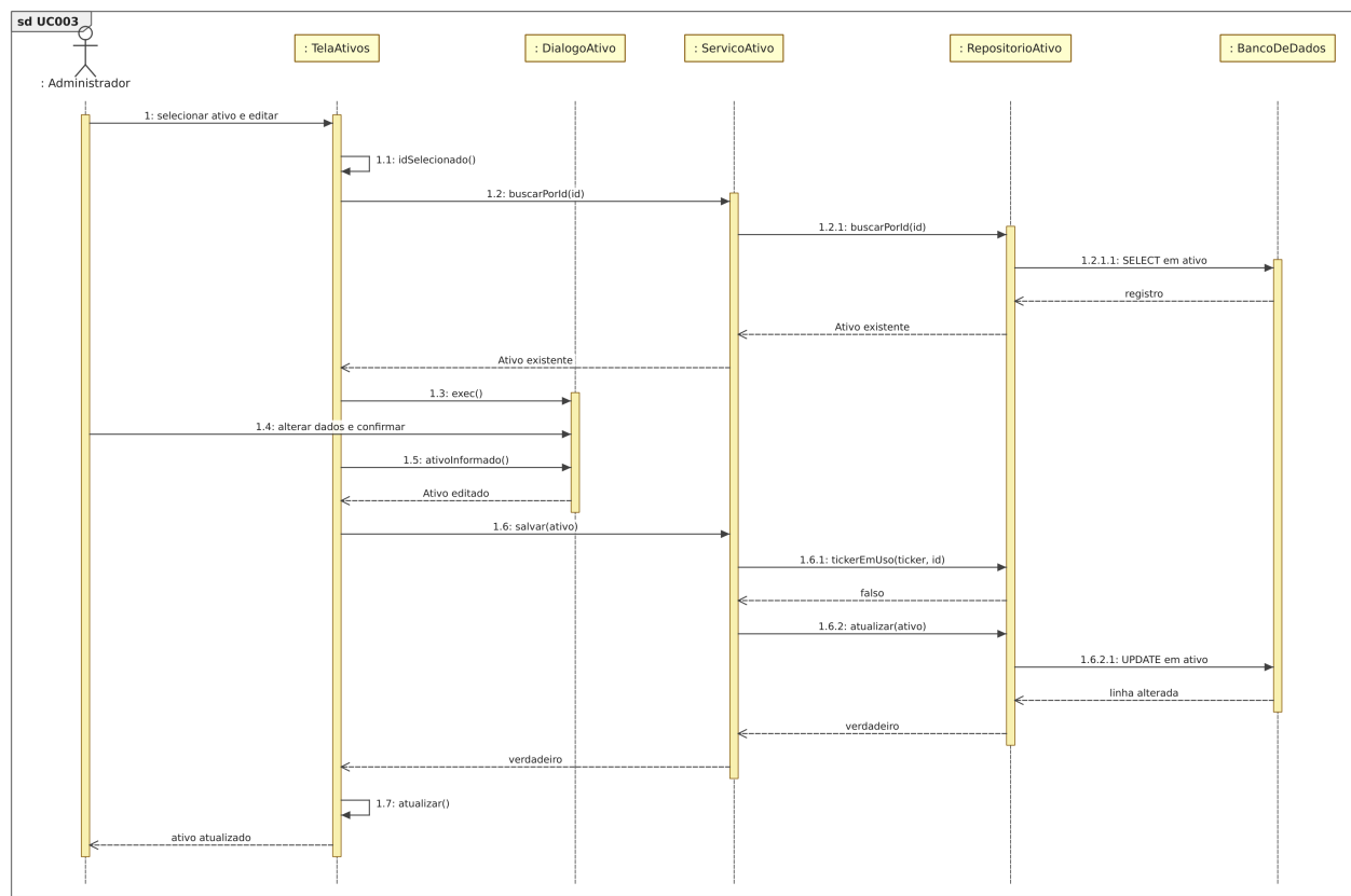
Figura 22: Figura 22. Diagrama de sequência para o [UC003].
