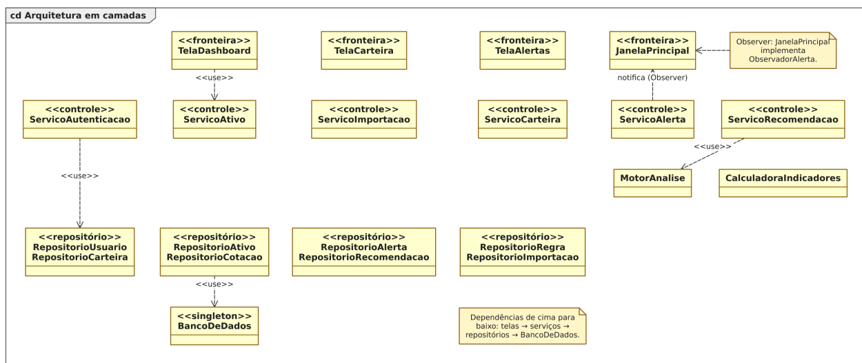
Figura 17: Figura 17. Diagrama de classes da arquitetura em camadas.
