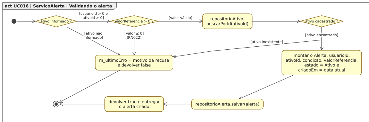
Figura 131: Figura 131. Diagrama de Atividades para o estado “Validando o alerta”, dentro do Diagrama de Estados para a classe ServicoAlerta em [UC016].
