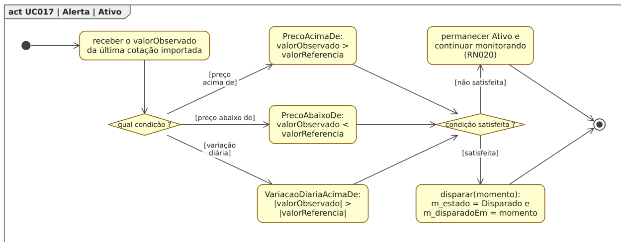
Figura 134: Figura 134. Diagrama de Atividades para o estado “Ativo”, dentro do Diagrama de Estados para a classe Alerta em [UC017].
