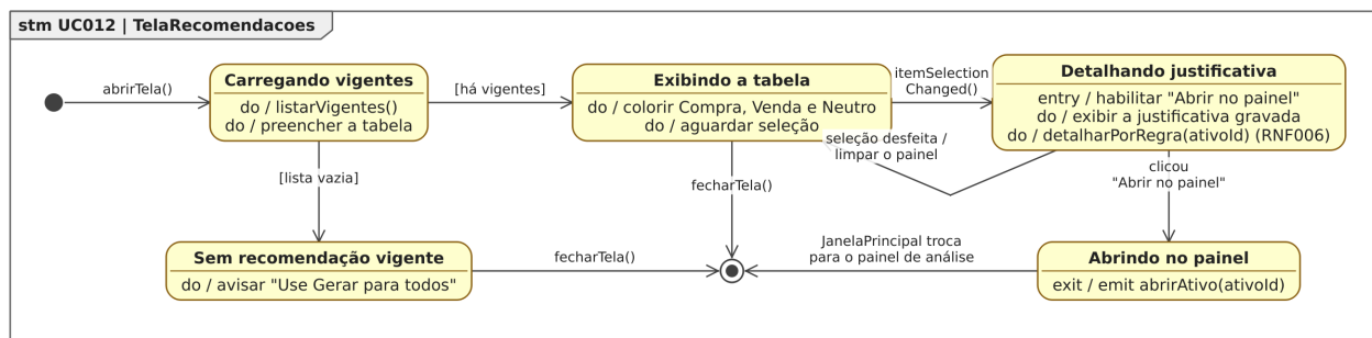
Figura 81: Figura 81. Diagrama de Estados da classe TelaRecomendacoes para o [UC012].
