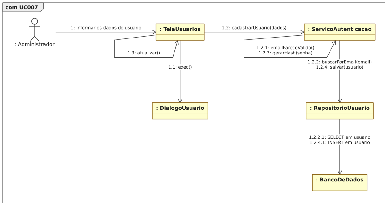
Figura 44: Figura 44. Diagrama de comunicação para o [UC007].
