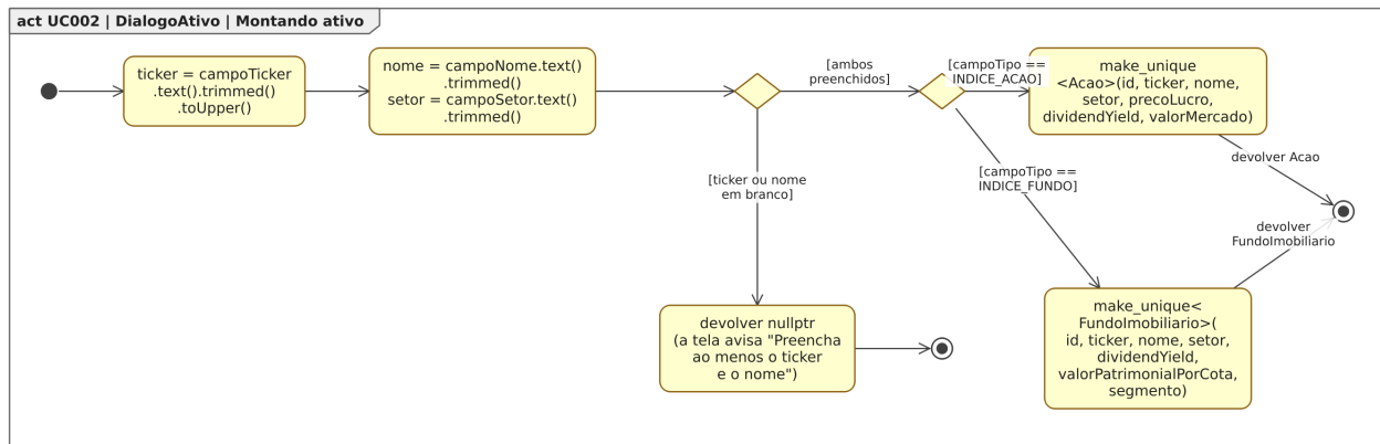
Figura 99: Figura 99. Diagrama de Atividades para o estado “Montando ativo”, dentro do Diagrama de Estados para a classe DialogoAtivo em [UC002].
