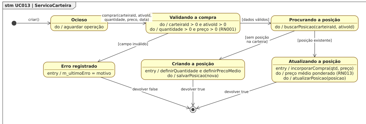
Figura 84: Figura 84. Diagrama de Estados da classe ServicoCarteira para o [UC013].
