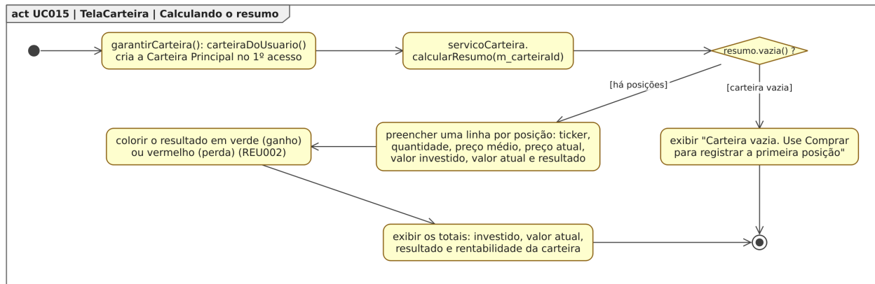
Figura 128: Figura 128. Diagrama de Atividades para o estado “Calculando o resumo”, dentro do Diagrama de Estados para a classe TelaCarteira em [UC015].
