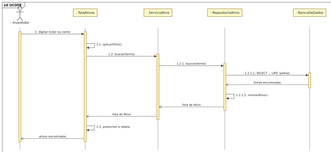
Figura 27: Figura 27. Diagrama de sequência para o [UC008].
