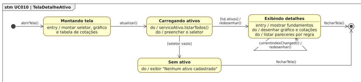
Figura 76: Figura 76. Diagrama de Estados da classe TelaDetalheAtivo para o [UC010].
