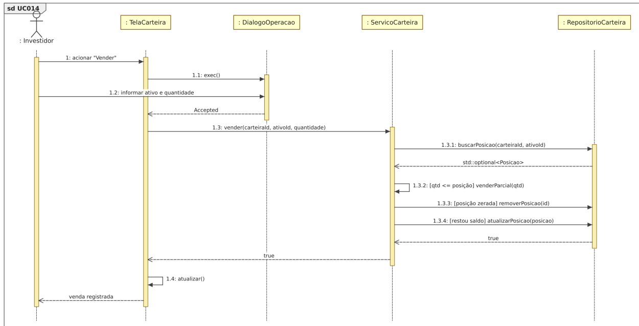
Figura 33: Figura 33. Diagrama de sequência para o [UC014].
