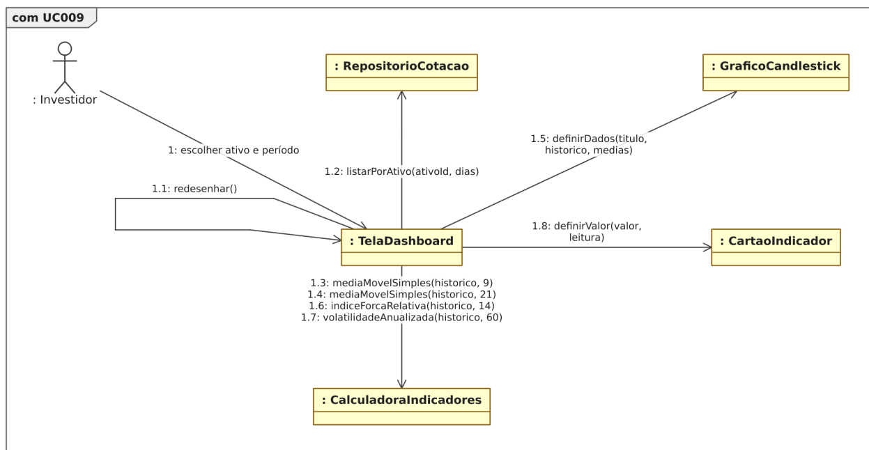
Figura 46: Figura 46. Diagrama de comunicação para o [UC009].
