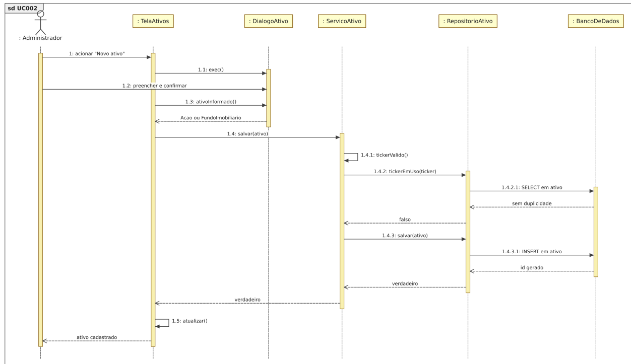
Figura 21: Figura 21. Diagrama de sequência para o [UC002].
