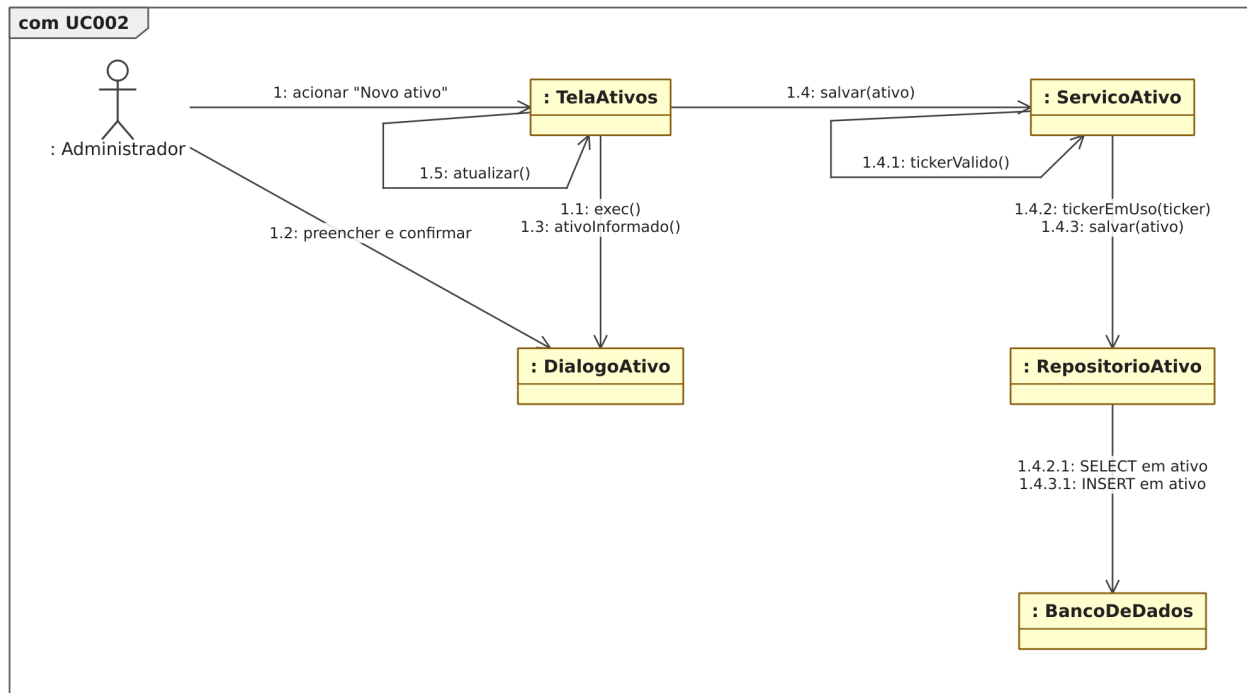
Figura 39: Figura 39. Diagrama de comunicação para o [UC002].
