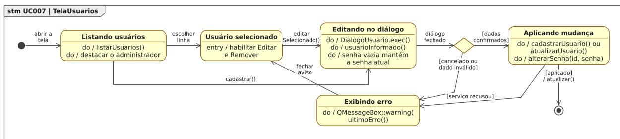
Figura 70: Figura 70. Diagrama de Estados da classe TelaUsuarios para o [UC007].
