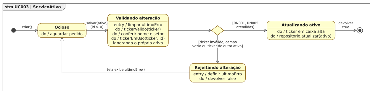
Figura 62: Figura 62. Diagrama de Estados da classe ServicoAtivo para o [UC003].
