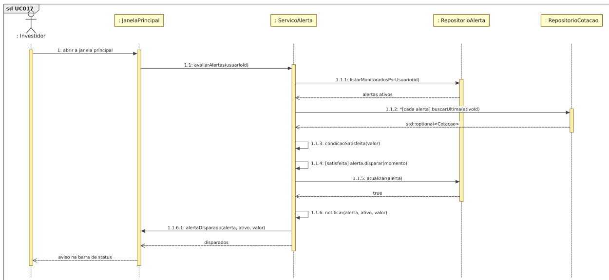
Figura 36: Figura 36. Diagrama de sequência para o [UC017].
