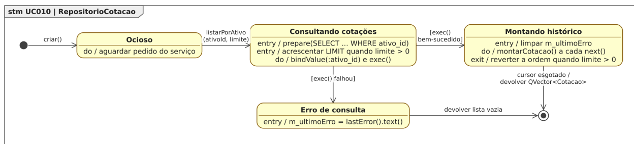
Figura 77: Figura 77. Diagrama de Estados da classe RepositorioCotacao para o [UC010].
