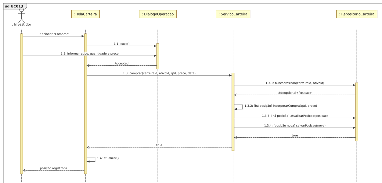
Figura 32: Figura 32. Diagrama de sequência para o [UC013].
