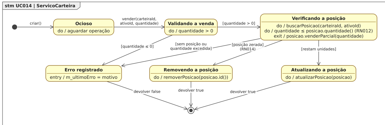
Figura 86: Figura 86. Diagrama de Estados da classe ServicoCarteira para o [UC014].
