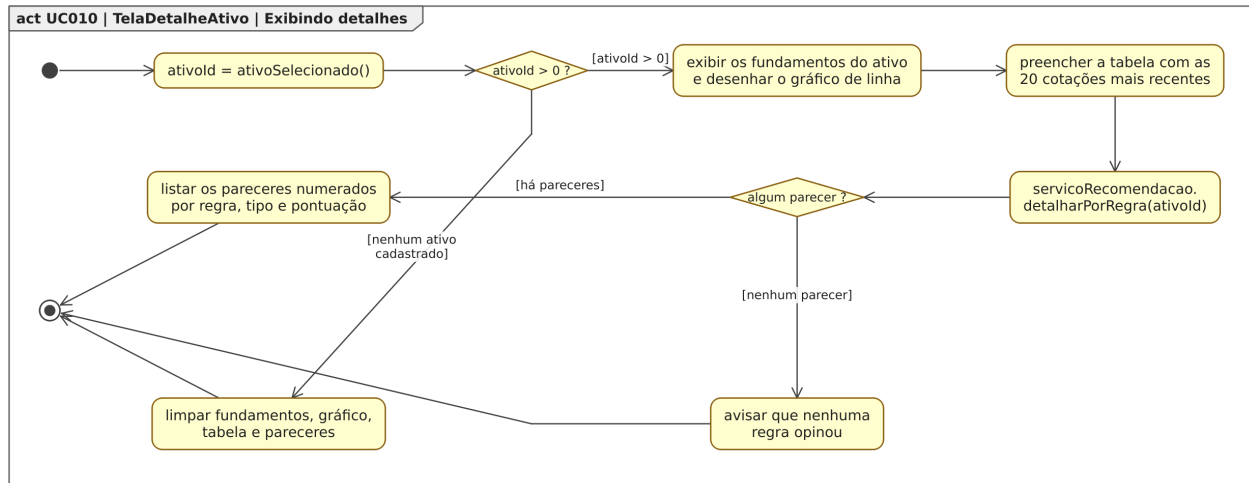
Figura 116: Figura 116. Diagrama de Atividades para o estado “Exibindo detalhes”, dentro do Diagrama de Estados para a classe TelaDetalheAtivo em [UC010].
