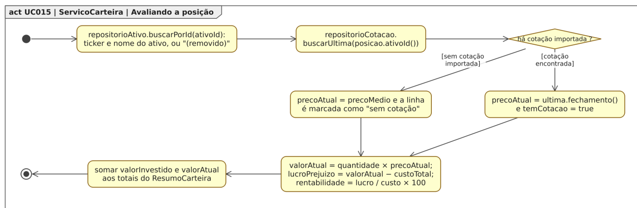
Figura 129: Figura 129. Diagrama de Atividades para o estado “Avaliando a posição”, dentro do Diagrama de Estados para a classe ServicoCarteira em [UC015].
