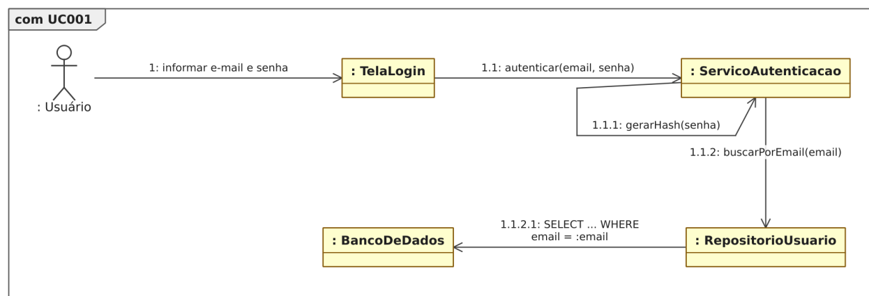
Figura 38: Figura 38. Diagrama de comunicação para o [UC001].
