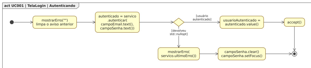
Figura 97: Figura 97. Diagrama de Atividades para o estado “Autenticando”, dentro do Diagrama de Estados para a classe TelaLogin em [UC001].
