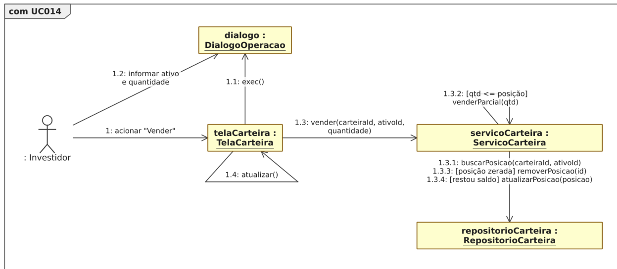
Figura 51: Figura 51. Diagrama de comunicação para o [UC014].
