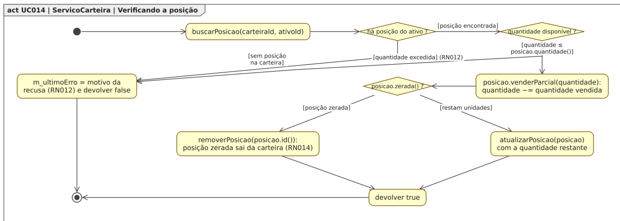
Figura 126: Figura 126. Diagrama de Atividades para o estado “Verificando a posição”, dentro do Diagrama de Estados para a classe ServicoCarteira em [UC014].
