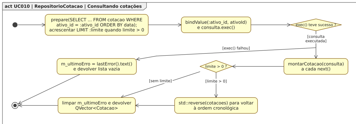
Figura 117: Figura 117. Diagrama de Atividades para o estado “Consultando cotações”, dentro do Diagrama de Estados para a classe RepositorioCotacao em [UC010].
