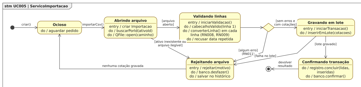
Figura 66: Figura 66. Diagrama de Estados da classe ServicoImportacao para o [UC005].
