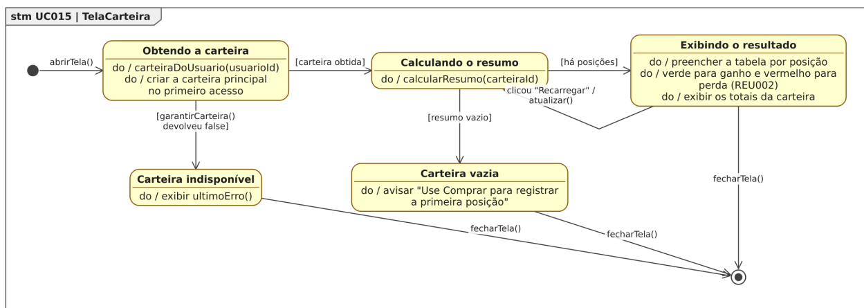
Figura 88: Figura 88. Diagrama de Estados da classe TelaCarteira para o [UC015].
