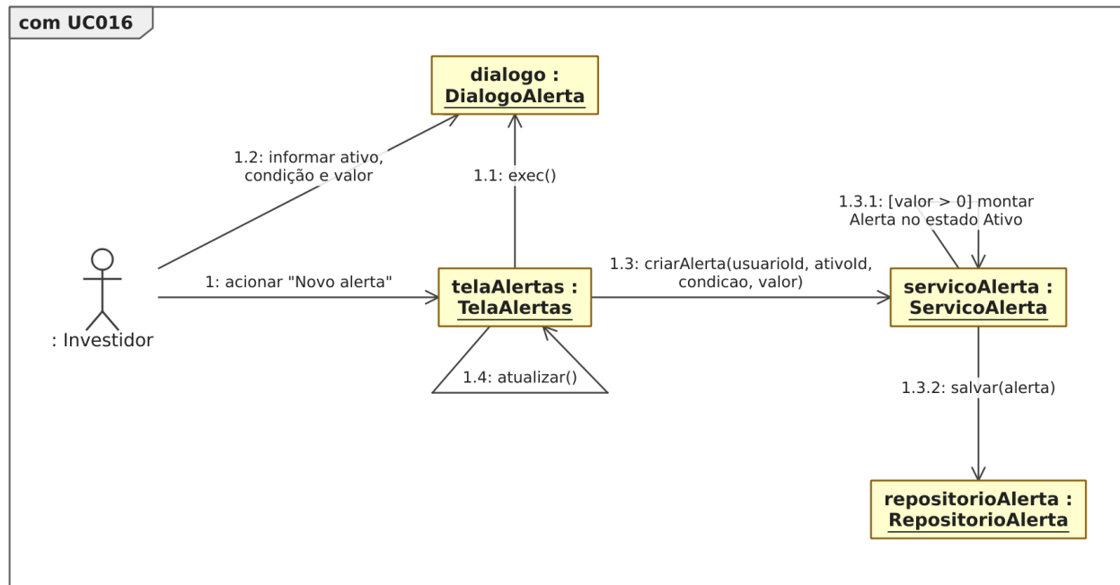
Figura 53: Figura 53. Diagrama de comunicação para o [UC016].
