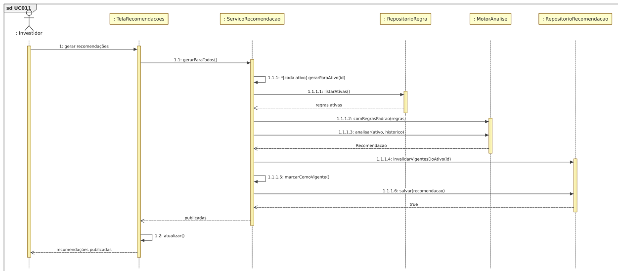
Figura 30: Figura 30. Diagrama de sequência para o [UC011].
