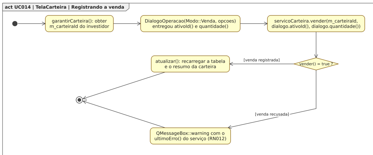
Figura 125: Figura 125. Diagrama de Atividades para o estado “Registrando a venda”, dentro do Diagrama de Estados para a classe TelaCarteira em [UC014].
