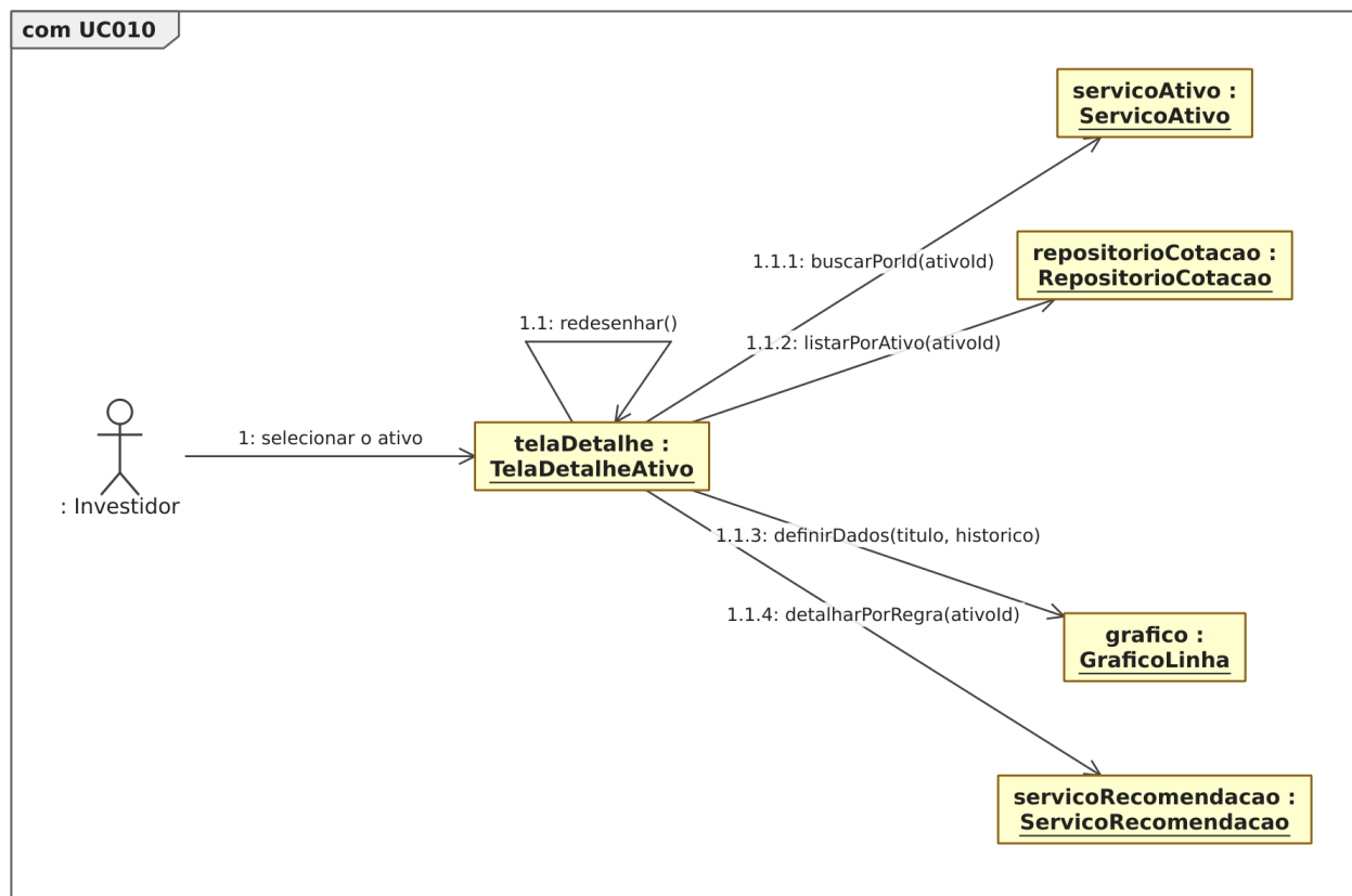
Figura 47: Figura 47. Diagrama de comunicação para o [UC010].
