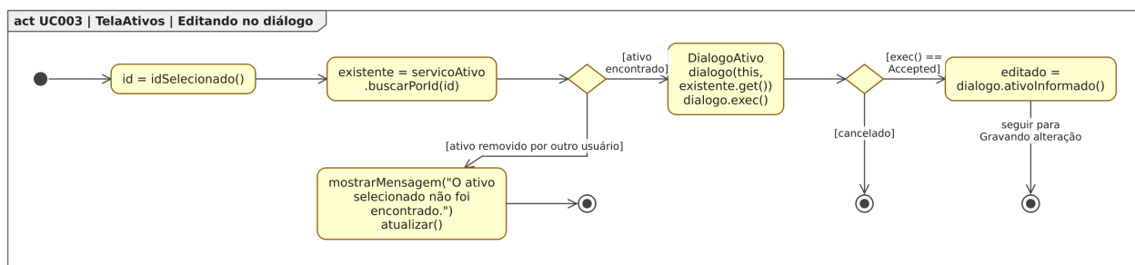
Figura 101: Figura 101. Diagrama de Atividades para o estado “Editando no diálogo”, dentro do Diagrama de Estados para a classe TelaAtivos em [UC003].
