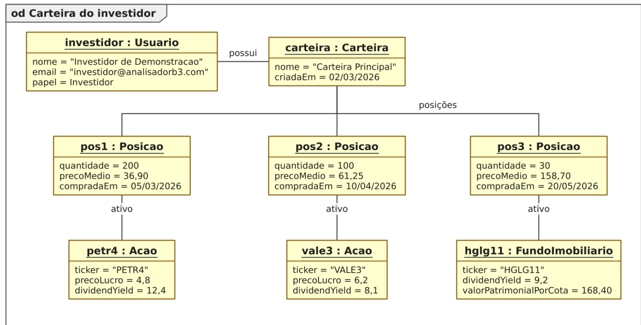
Figura 19: Figura 19. Diagrama de objetos da carteira do investidor.
