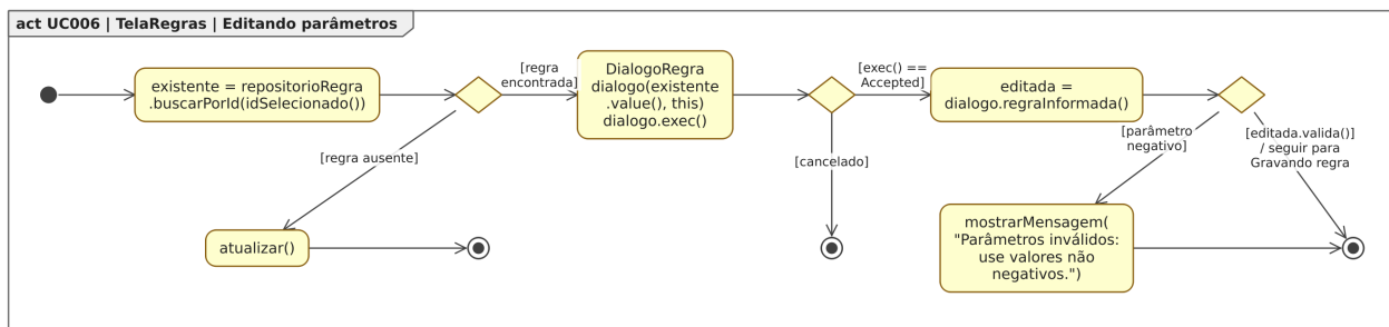
Figura 108: Figura 108. Diagrama de Atividades para o estado “Editando parâmetros”, dentro do Diagrama de Estados para a classe TelaRegras em [UC006].
