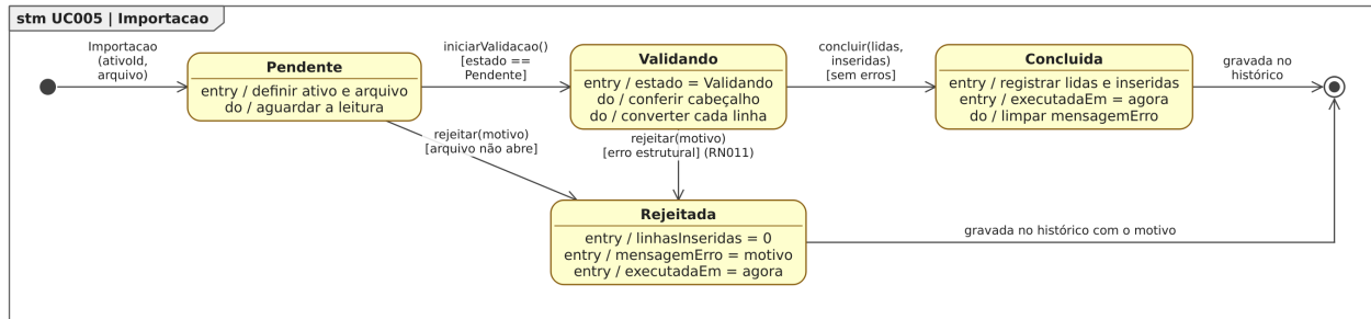
Figura 67: Figura 67. Diagrama de Estados da classe Importacao para o [UC005].
