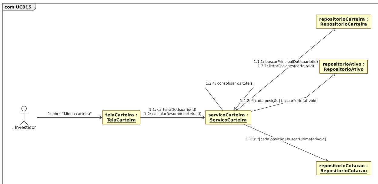
Figura 52: Figura 52. Diagrama de comunicação para o [UC015].
