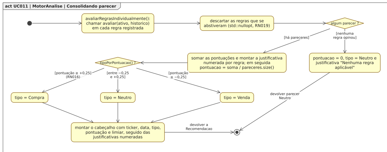
Figura 119: Figura 119. Diagrama de Atividades para o estado “Consolidando parecer”, dentro do Diagrama de Estados para a classe MotorAnalise em [UC011].
