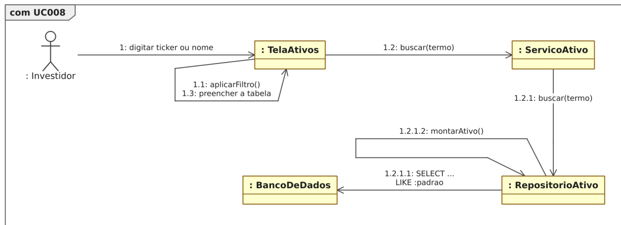
Figura 45: Figura 45. Diagrama de comunicação para o [UC008].
