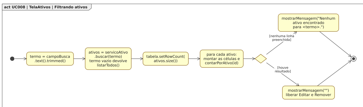
Figura 112: Figura 112. Diagrama de Atividades para o estado “Filtrando ativos”, dentro do Diagrama de Estados para a classe TelaAtivos em [UC008].
