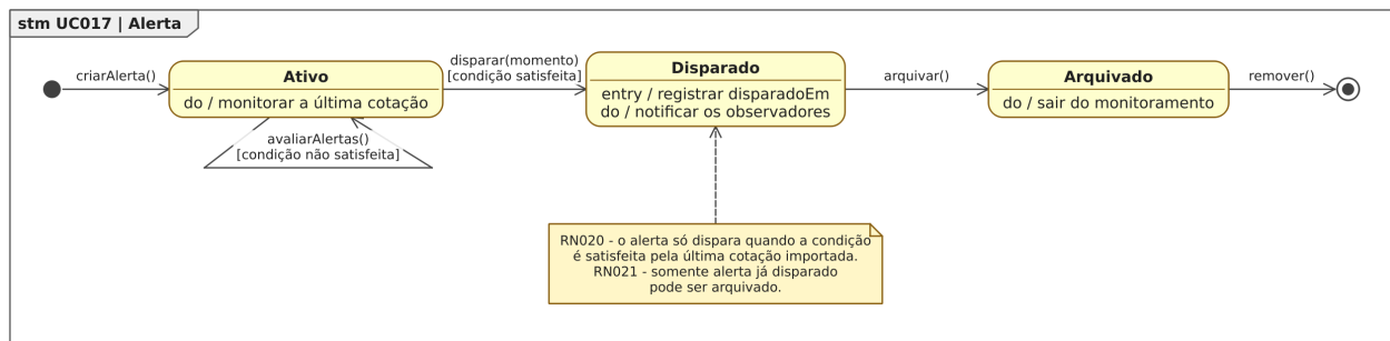
Figura 94: Figura 94. Diagrama de Estados da classe Alerta para o [UC017].
