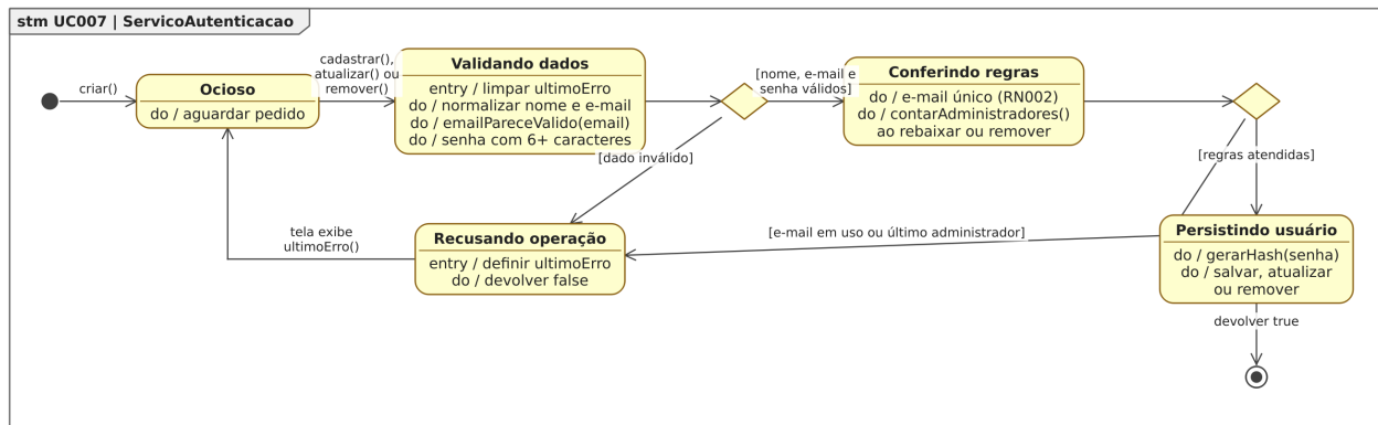
Figura 71: Figura 71. Diagrama de Estados da classe ServicoAutenticacao para o [UC007].
