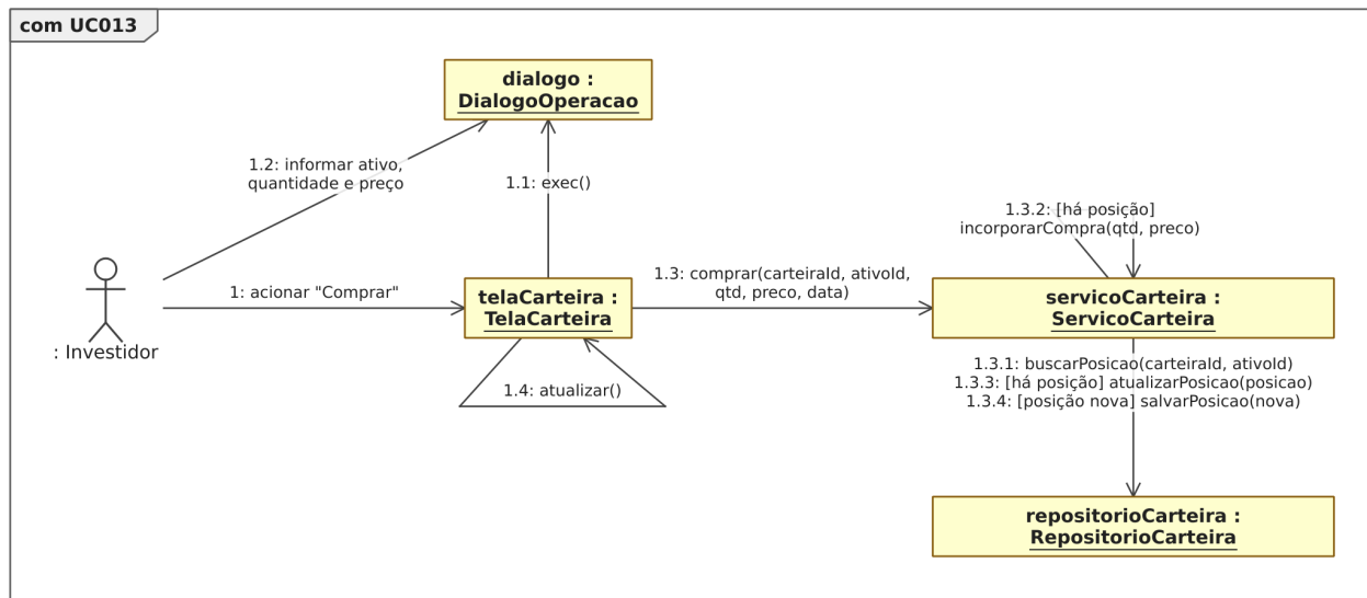
Figura 50: Figura 50. Diagrama de comunicação para o [UC013].
