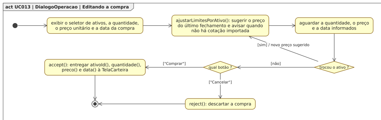
Figura 123: Figura 123. Diagrama de Atividades para o estado “Editando a compra”, dentro do Diagrama de Estados para a classe DialogoOperacao em [UC013].
