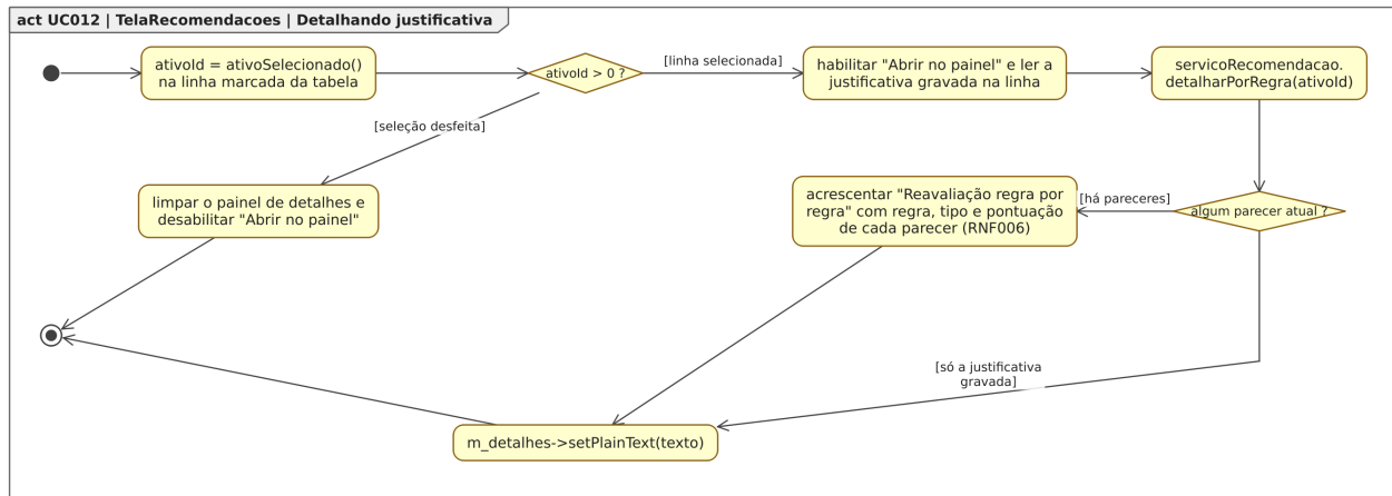
Figura 121: Figura 121. Diagrama de Atividades para o estado “Detalhando justificativa”, dentro do Diagrama de Estados para a classe TelaRecomendacoes em [UC012].
