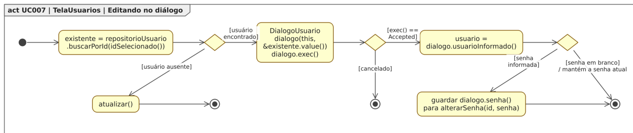
Figura 110: Figura 110. Diagrama de Atividades para o estado “Editando no diálogo”, dentro do Diagrama de Estados para a classe TelaUsuarios em [UC007].
