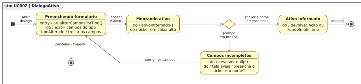
Figura 59: Figura 59. Diagrama de Estados da classe DialogoAtivo para o [UC002].
