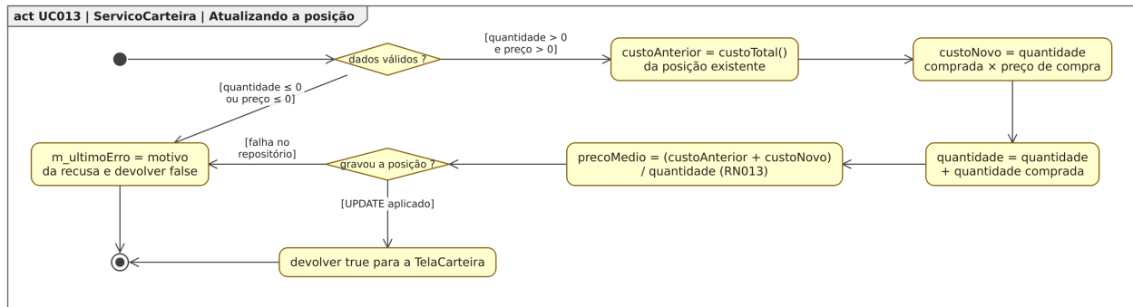
Figura 124: Figura 124. Diagrama de Atividades para o estado “Atualizando a posição”, dentro do Diagrama de Estados para a classe ServicoCarteira em [UC013].
