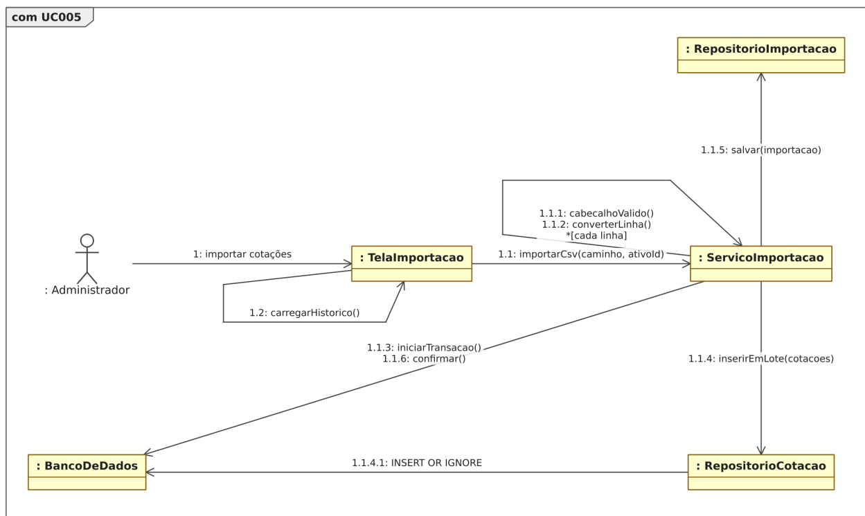
Figura 42: Figura 42. Diagrama de comunicação para o [UC005].
