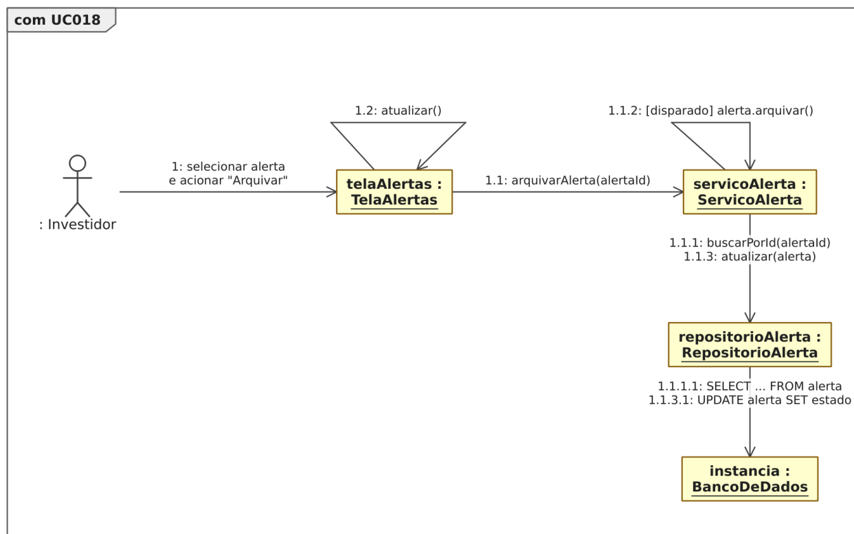
Figura 55: Figura 55. Diagrama de comunicação para o [UC018].
