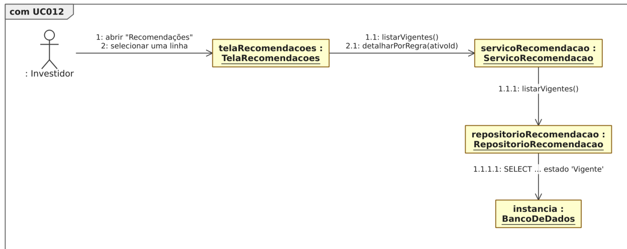
Figura 49: Figura 49. Diagrama de comunicação para o [UC012].
