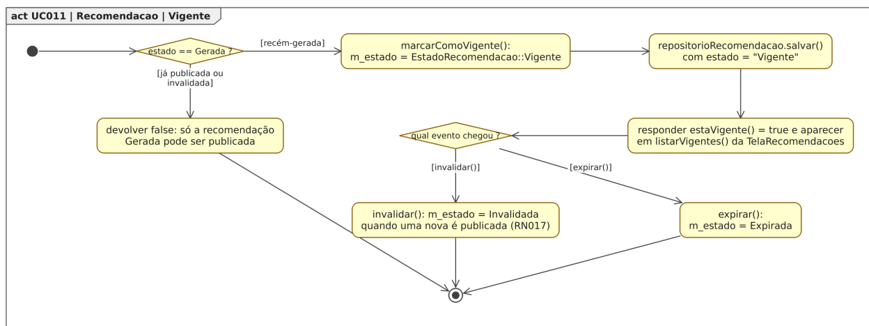
Figura 120: Figura 120. Diagrama de Atividades para o estado “Vigente”, dentro do Diagrama de Estados para a classe Recomendacao em [UC011].
