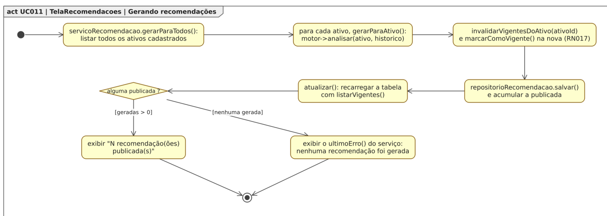
Figura 118: Figura 118. Diagrama de Atividades para o estado “Gerando recomendações”, dentro do Diagrama de Estados para a classe TelaRecomendacoes em [UC011].
