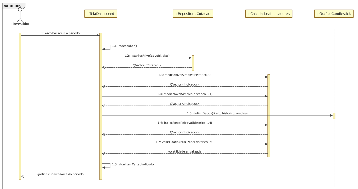
Figura 28: Figura 28. Diagrama de sequência para o [UC009].
