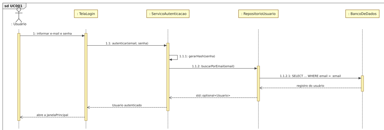
Figura 20: Figura 20. Diagrama de sequência para o [UC001].
