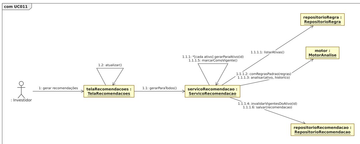
Figura 48: Figura 48. Diagrama de comunicação para o [UC011].
