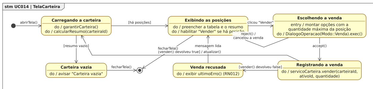
Figura 85: Figura 85. Diagrama de Estados da classe TelaCarteira para o [UC014].
