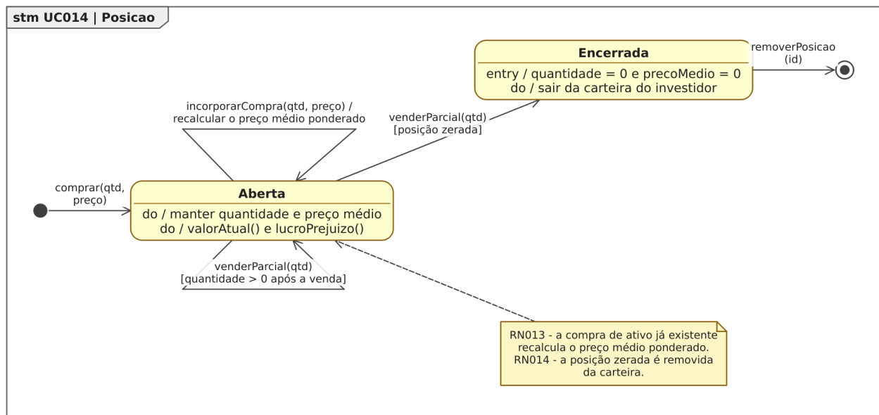
Figura 87: Figura 87. Diagrama de Estados da classe Posicao para o [UC014].
