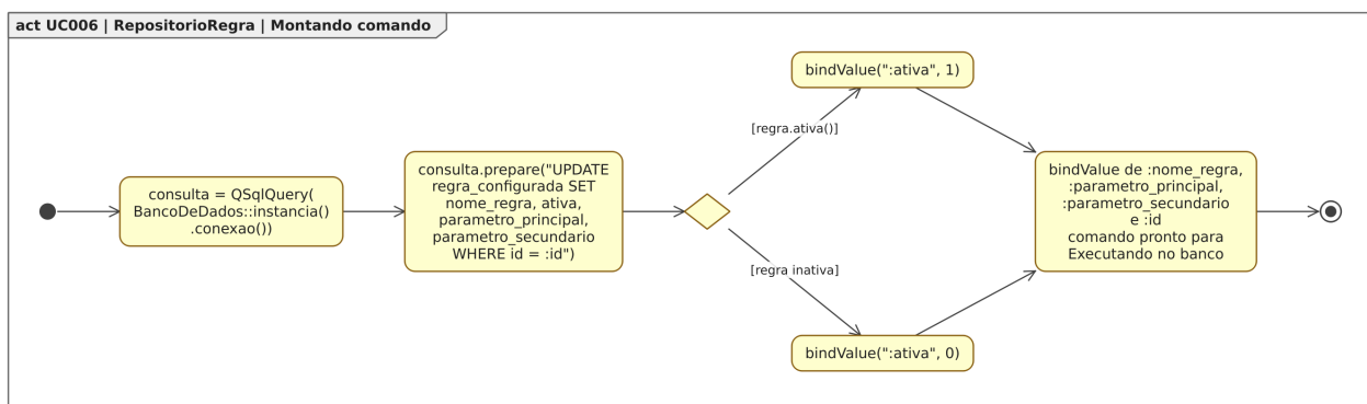
Figura 109: Figura 109. Diagrama de Atividades para o estado “Montando comando”, dentro do Diagrama de Estados para a classe RepositorioRegra em [UC006].
