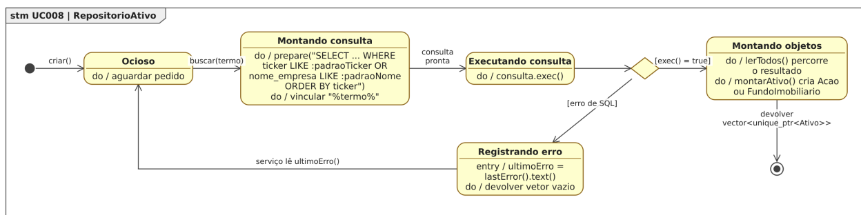
Figura 73: Figura 73. Diagrama de Estados da classe RepositorioAtivo para o [UC008].
