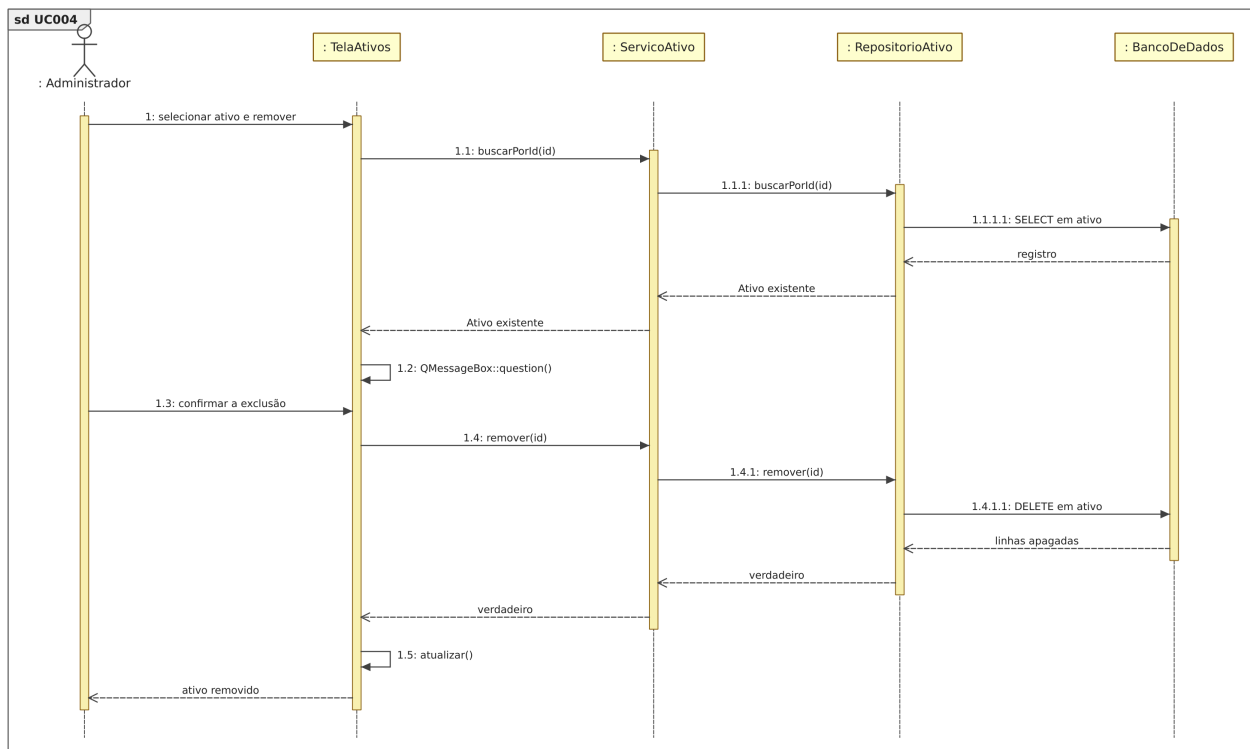
Figura 23: Figura 23. Diagrama de sequência para o [UC004].
