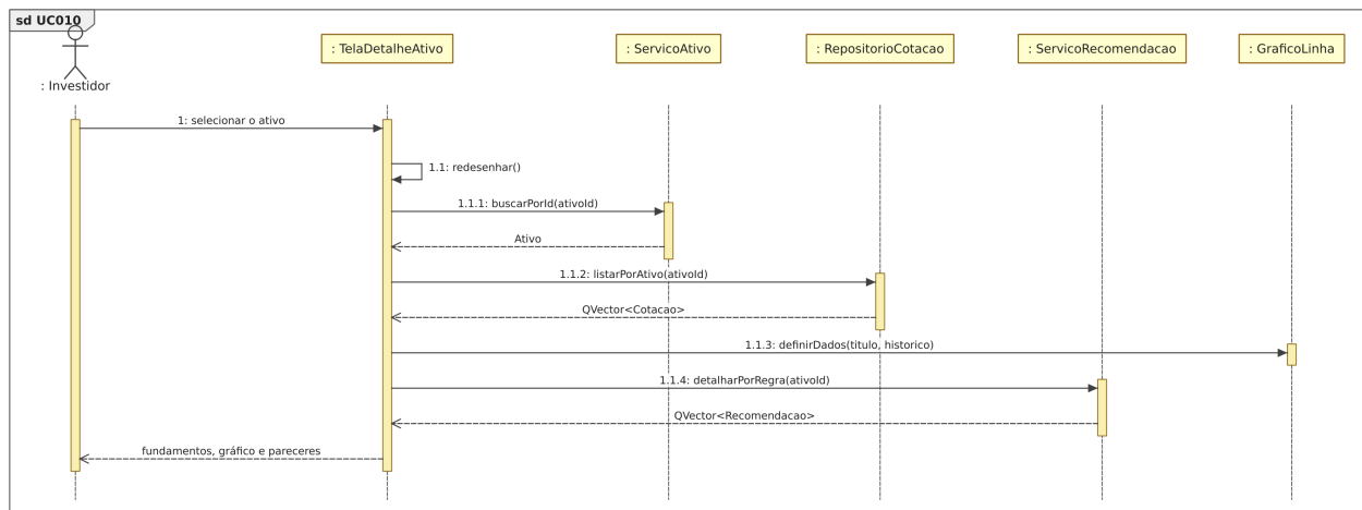
Figura 29: Figura 29. Diagrama de sequência para o [UC010].
