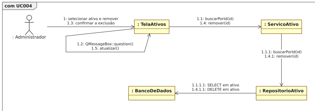
Figura 41: Figura 41. Diagrama de comunicação para o [UC004].
