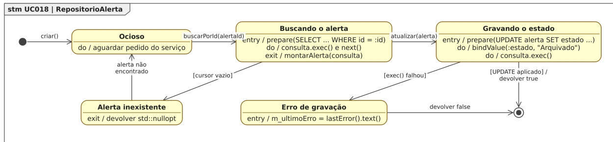
Figura 96: Figura 96. Diagrama de Estados da classe RepositorioAlerta para o [UC018].
