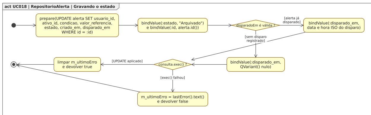
Figura 136: Figura 136. Diagrama de Atividades para o estado “Gravando o estado”, dentro do Diagrama de Estados para a classe RepositorioAlerta em [UC018].
