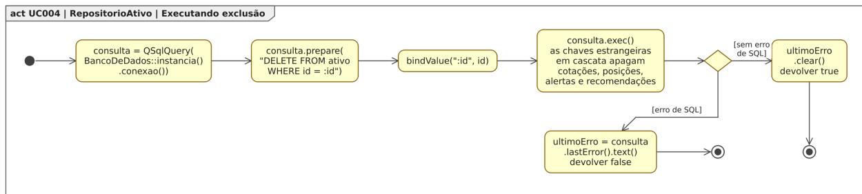
Figura 104: Figura 104. Diagrama de Atividades para o estado “Executando exclusão”, dentro do Diagrama de Estados para a classe RepositorioAtivo em [UC004].
