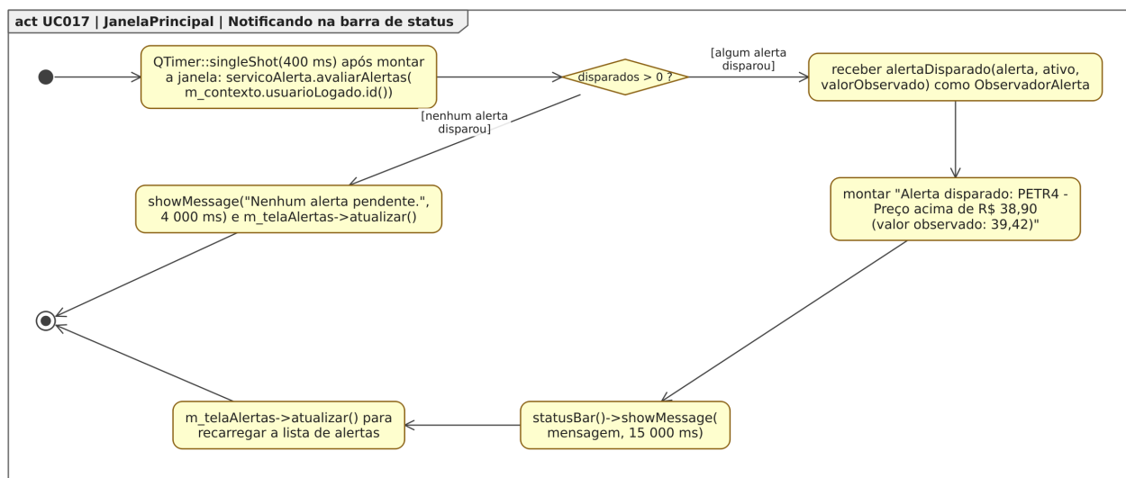
Figura 132: Figura 132. Diagrama de Atividades para o estado “Notificando na barra de status”, dentro do Diagrama de Estados para a classe JanelaPrincipal em [UC017].
