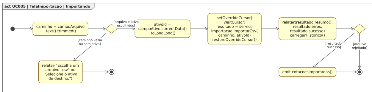
Figura 105: Figura 105. Diagrama de Atividades para o estado “Importando”, dentro do Diagrama de Estados para a classe TelaImportacao em [UC005].
