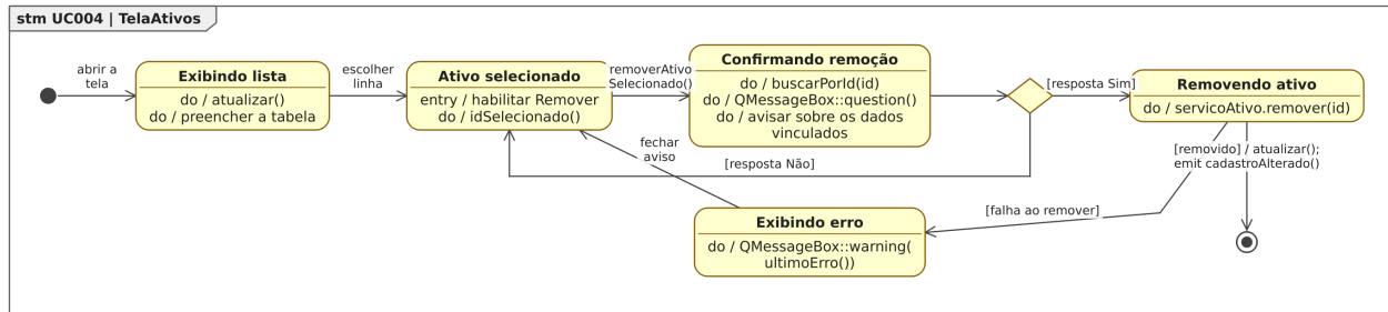
Figura 63: Figura 63. Diagrama de Estados da classe TelaAtivos para o [UC004].
