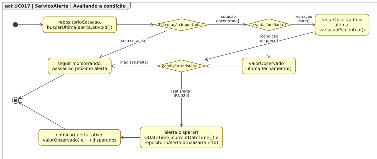
Figura 133: Figura 133. Diagrama de Atividades para o estado “Avaliando a condição”, dentro do Diagrama de Estados para a classe ServiçoAlerta em [UC017].
