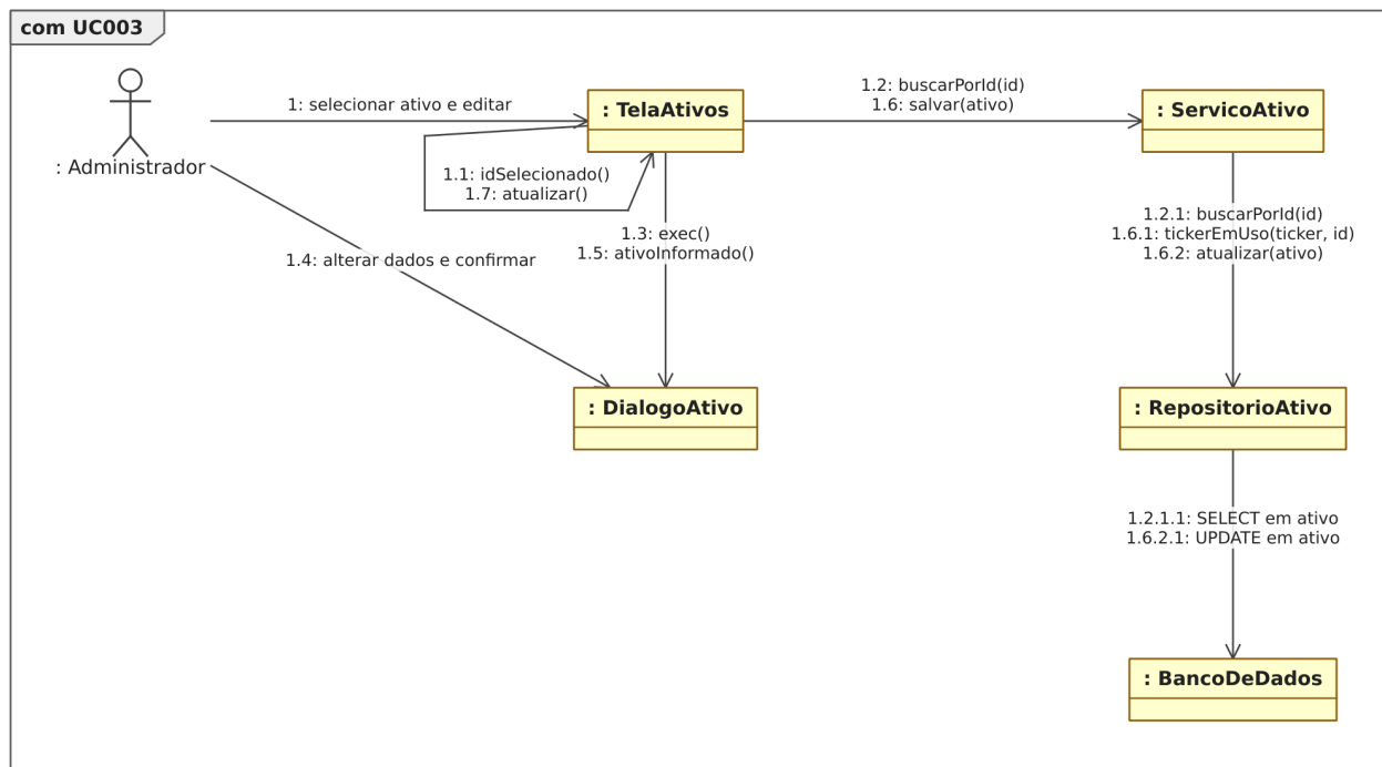
Figura 40: Figura 40. Diagrama de comunicação para o [UC003].
