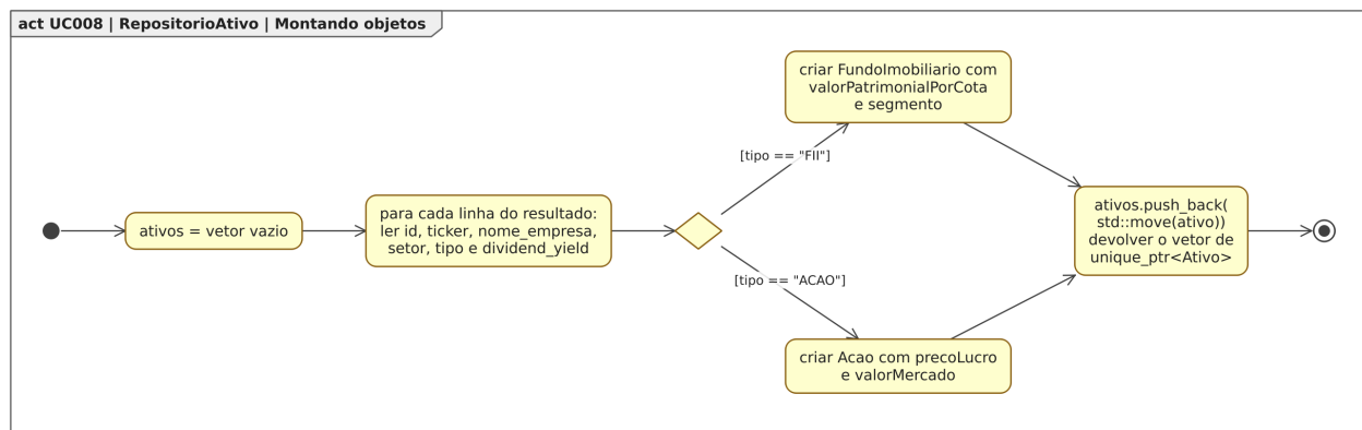
Figura 113: Figura 113. Diagrama de Atividades para o estado “Montando objetos”, dentro do Diagrama de Estados para a classe RepositorioAtivo em [UC008].
