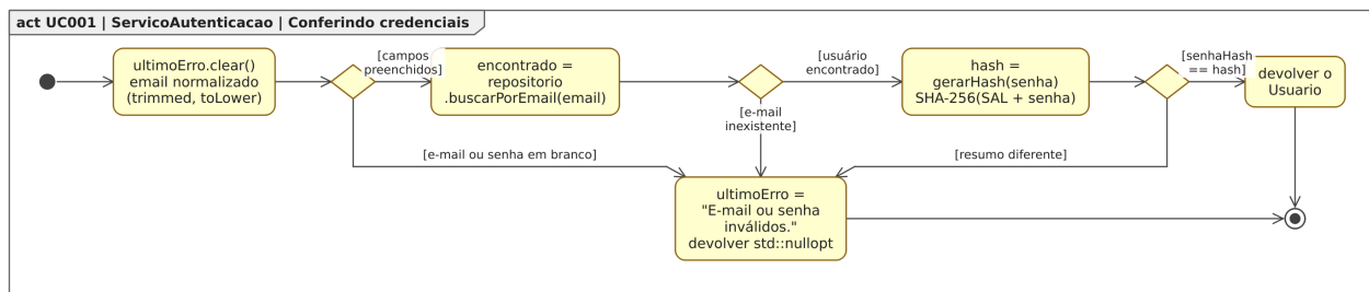
Figura 98: Figura 98. Diagrama de Atividades para o estado “Conferindo credenciais”, dentro do Diagrama de Estados para a classe ServicoAutenticacao em [UC001].
