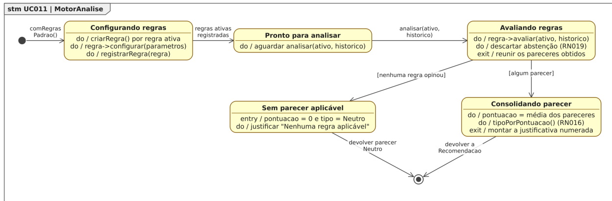
Figura 79: Figura 79. Diagrama de Estados da classe MotorAnalise para o [UC011].
