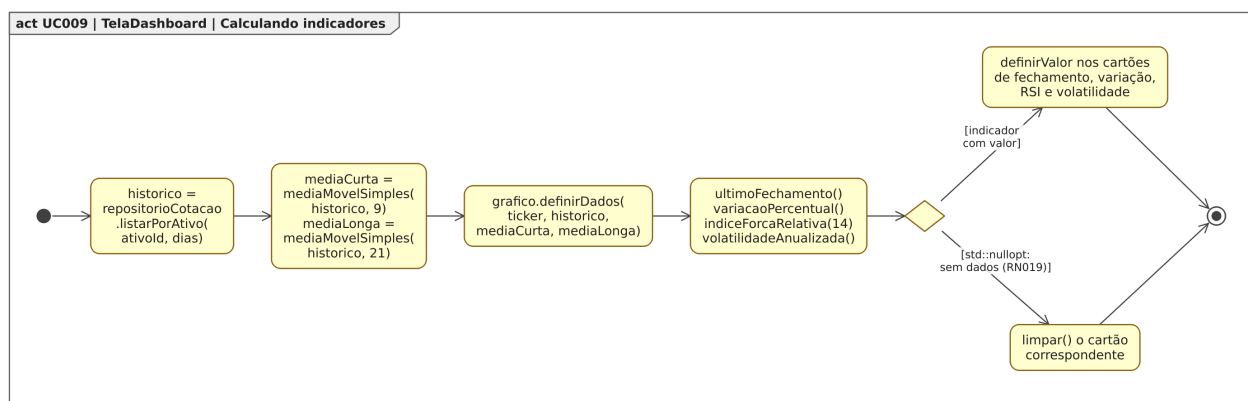
Figura 114: Figura 114. Diagrama de Atividades para o estado “Calculando indicadores”, dentro do Diagrama de Estados para a classe TelaDashboard em [UC009].
