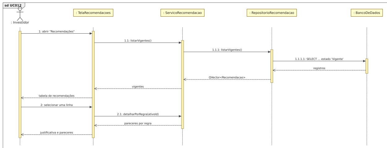
Figura 31: Figura 31. Diagrama de sequência para o [UC012].
