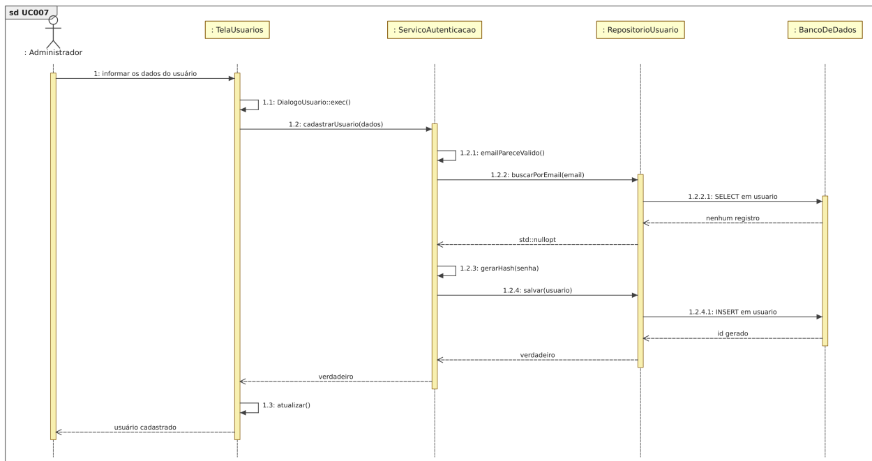
Figura 26: Figura 26. Diagrama de sequência para o [UC007].
