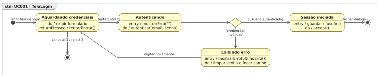
Figura 57: Figura 57. Diagrama de Estados da classe TelaLogin para o [UC001].
