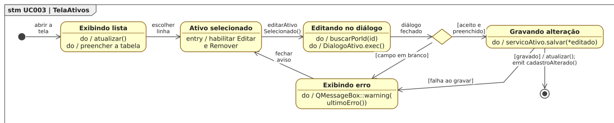
Figura 61: Figura 61. Diagrama de Estados da classe TelaAtivos para o [UC003].
