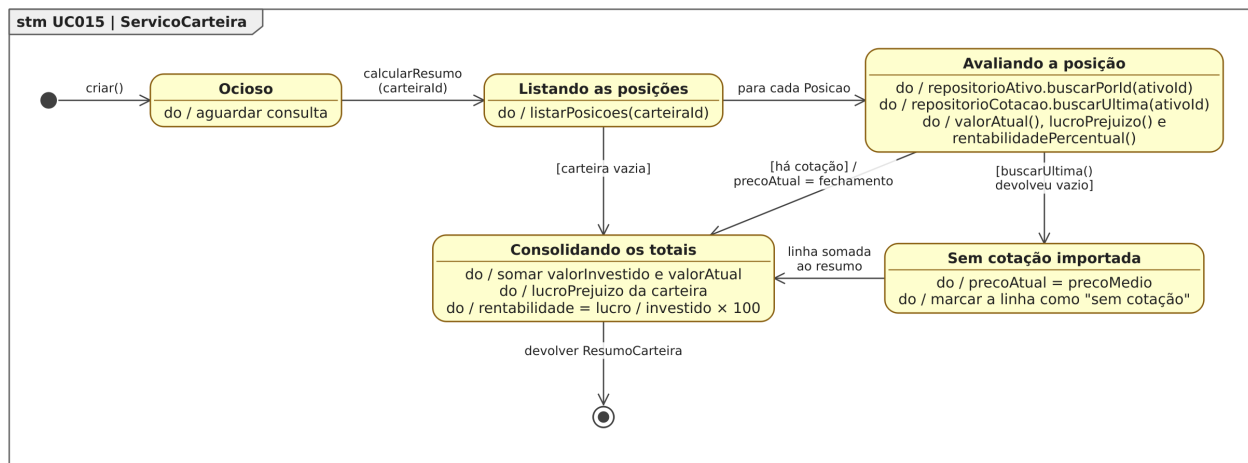
Figura 89: Figura 89. Diagrama de Estados da classe ServicoCarteira para o [UC015].
