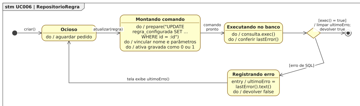
Figura 69: Figura 69. Diagrama de Estados da classe RepositorioRegra para o [UC006].
