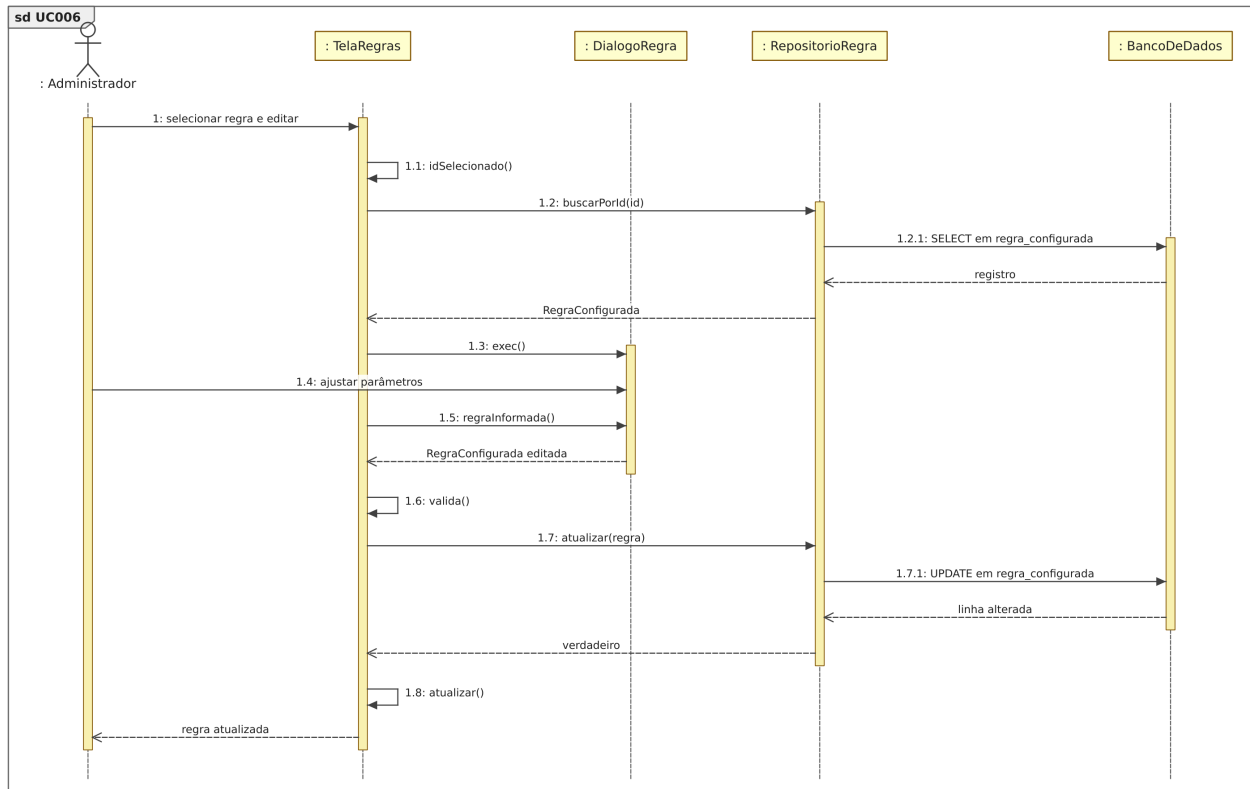
Figura 25. Diagrama de sequência para o [UC006].
