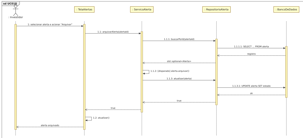
Figura 37. Diagrama de sequência para o [UC018].
