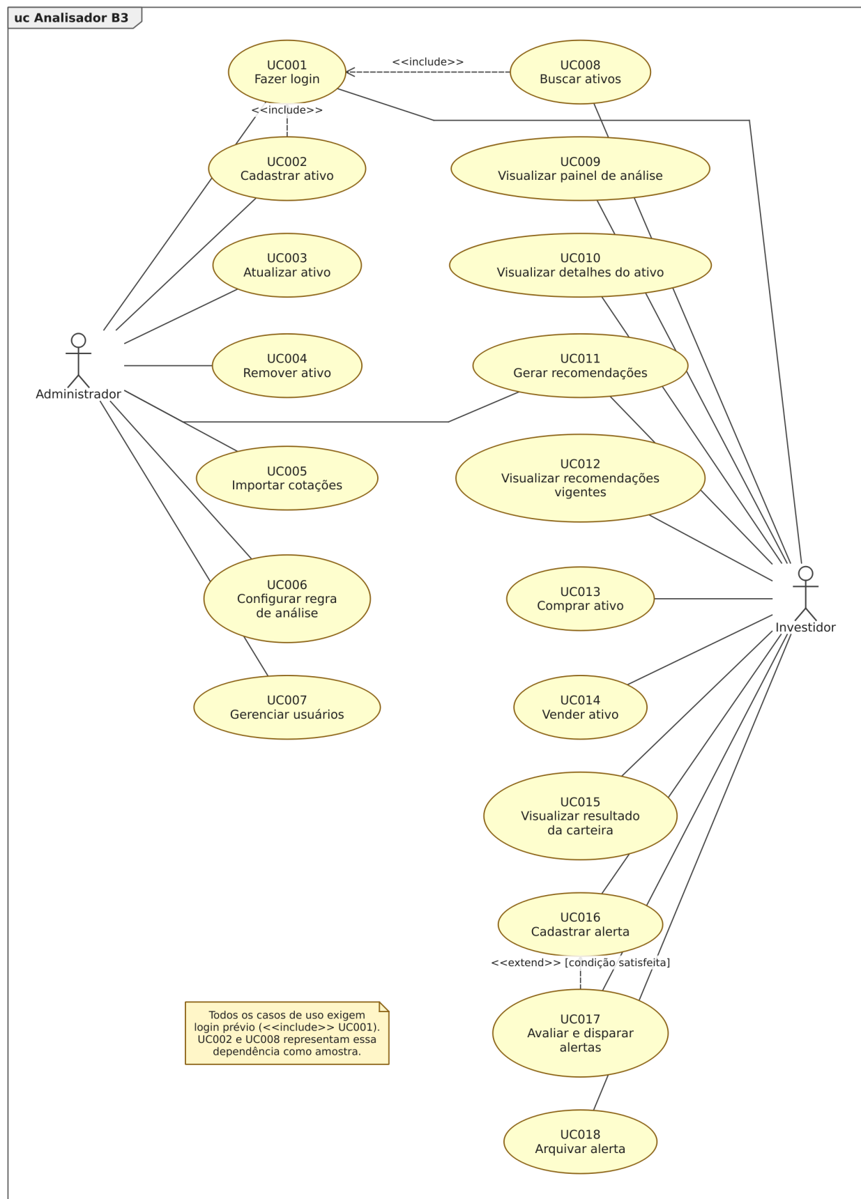
Figura 14. Diagrama de casos de uso.
