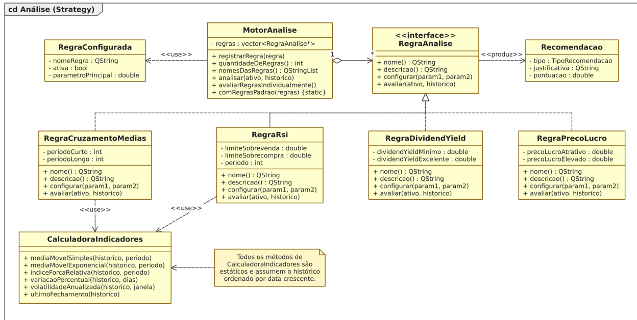
Figura 16. Diagrama de classes do núcleo de análise, com o padrão Strategy.
