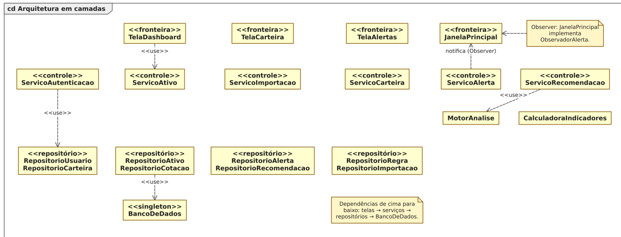
Figura 17. Diagrama de classes da arquitetura em camadas.
