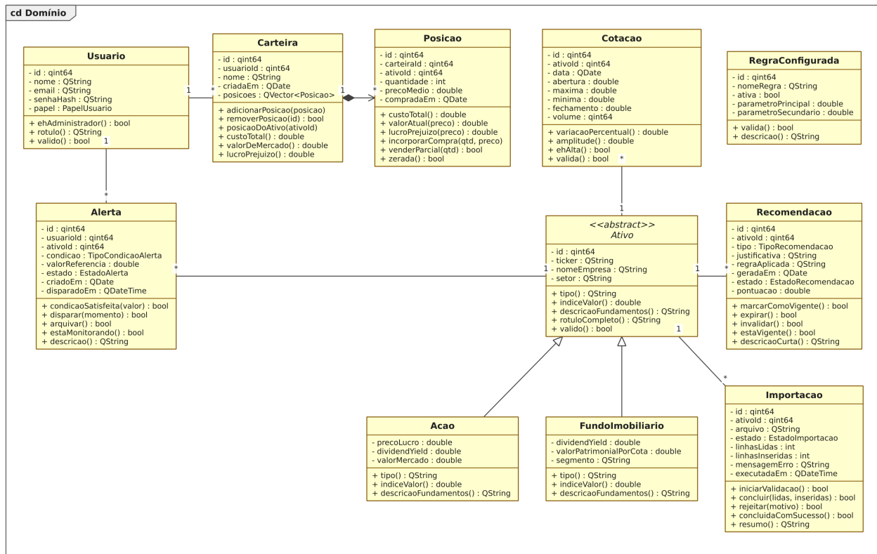
Figura 15. Diagrama de classes do domínio do sistema.
