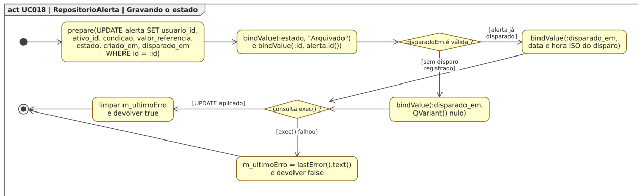
Figura 136. Diagrama de Atividades para o estado “Gravando o estado”, dentro do Diagrama de Estados para a classe RepositorioAlerta em [UC018].
