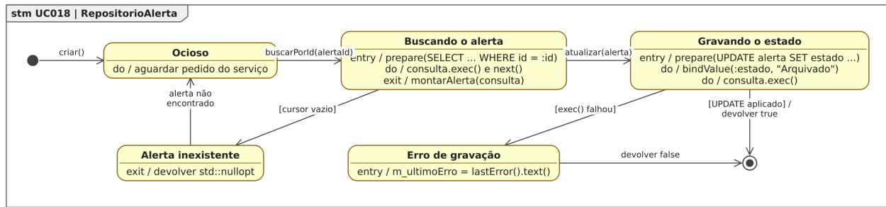
Figura 96. Diagrama de Estados da classe RepositorioAlerta para o [UC018].
