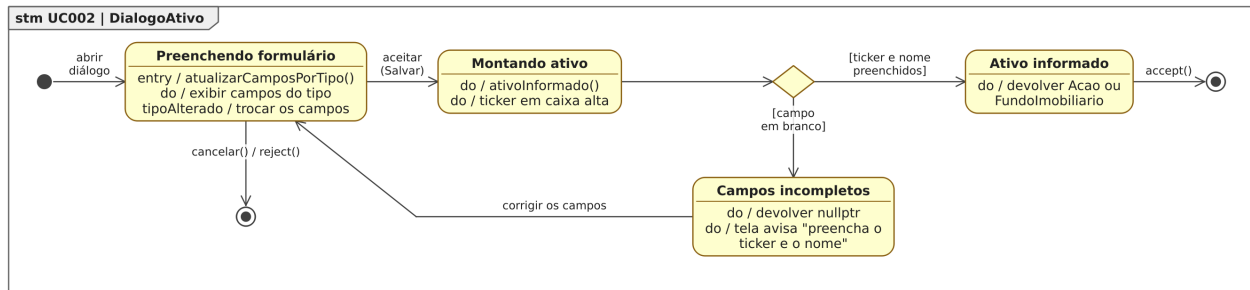
Figura 59. Diagrama de Estados da classe DialogoAtivo para o [UC002].
