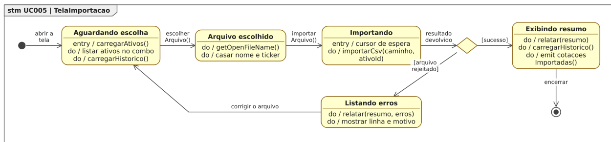
Figura 65. Diagrama de Estados da classe TelaImportacao para o [UC005].
