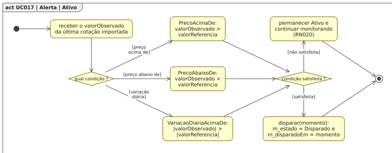
Figura 134. Diagrama de Atividades para o estado “Ativo”, dentro do Diagrama de Estados para a classe Alerta em [UC017].
