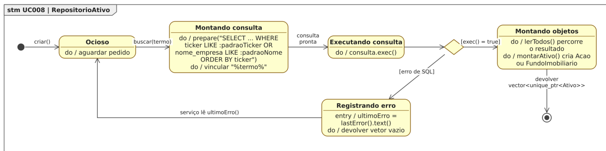
Figura 73. Diagrama de Estados da classe RepositorioAtivo para o [UC008].
