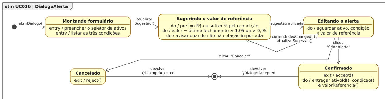
Figura 90. Diagrama de Estados da classe DialogoAlerta para o [UC016].
