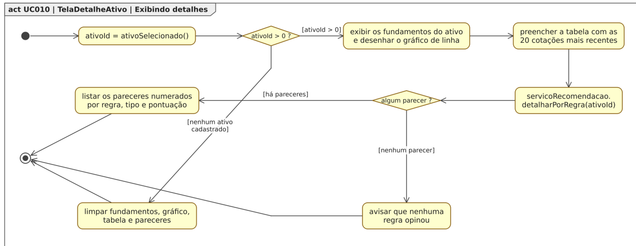
Figura 116. Diagrama de Atividades para o estado “Exibindo detalhes”, dentro do Diagrama de Estados para a classe TelaDetalheAtivo em [UC010].
