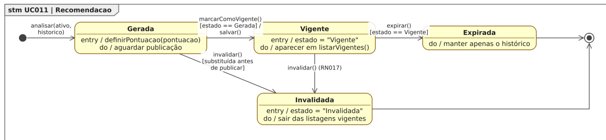
Figura 80. Diagrama de Estados da classe Recomendacao para o [UC011].
