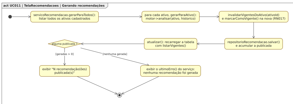
Figura 118. Diagrama de Atividades para o estado “Gerando recomendações”, dentro do Diagrama de Estados para a classe TelaRecomendacoes em [UC011].
