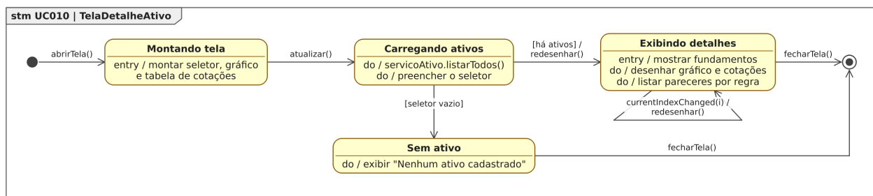
Figura 76. Diagrama de Estados da classe TelaDetalheAtivo para o [UC010].
