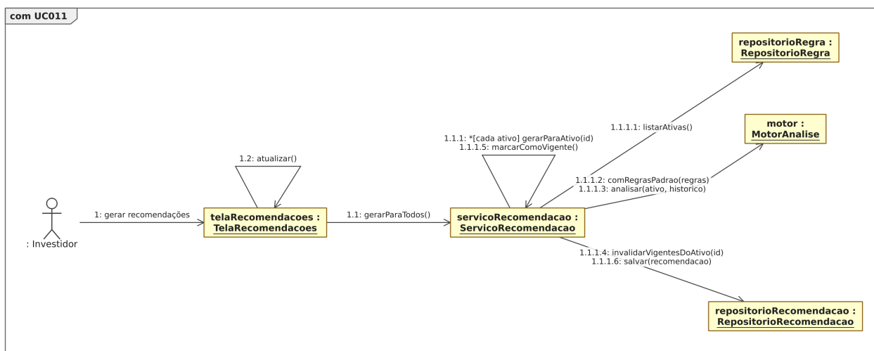
Figura 48. Diagrama de comunicação para o [UC011].
