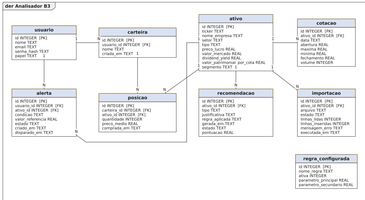
Figura 56. Diagrama Entidade-Relacionamento do banco de dados.
