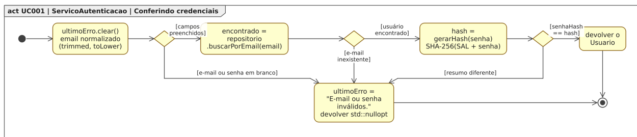
Figura 98. Diagrama de Atividades para o estado “Conferindo credenciais”, dentro do Diagrama de Estados para a classe ServicoAutenticacao em [UC001].
