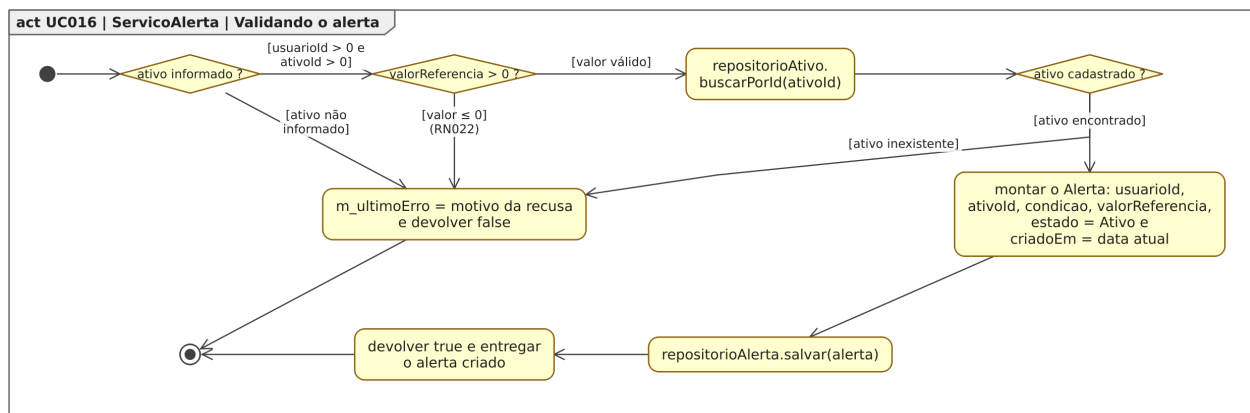
Figura 131. Diagrama de Atividades para o estado “Validando o alerta”, dentro do Diagrama de Estados para a classe ServicoAlerta em [UC016].
