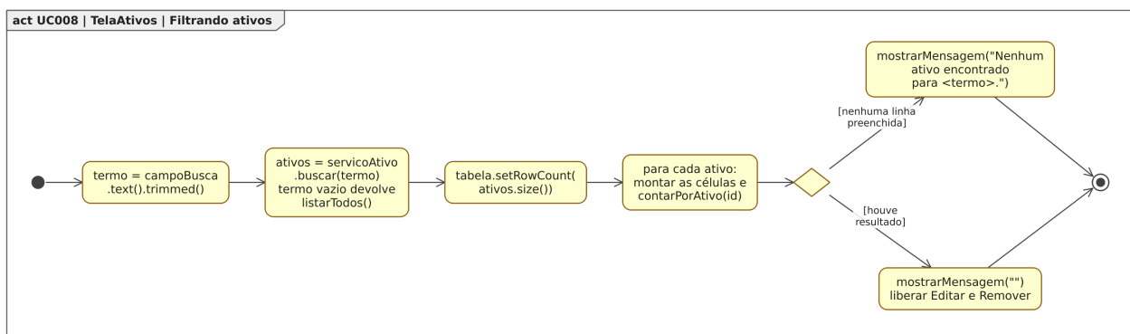
Figura 112. Diagrama de Atividades para o estado “Filtrando ativos”, dentro do Diagrama de Estados para a classe TelaAtivos em [UC008].
