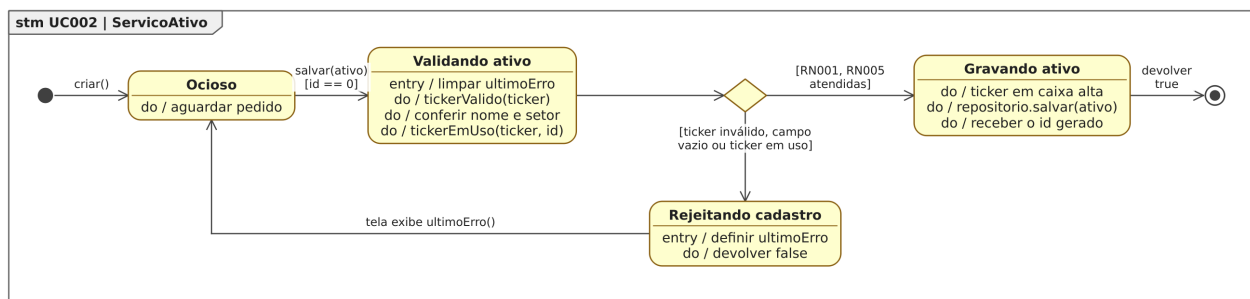
Figura 60. Diagrama de Estados da classe ServicoAtivo para o [UC002].
