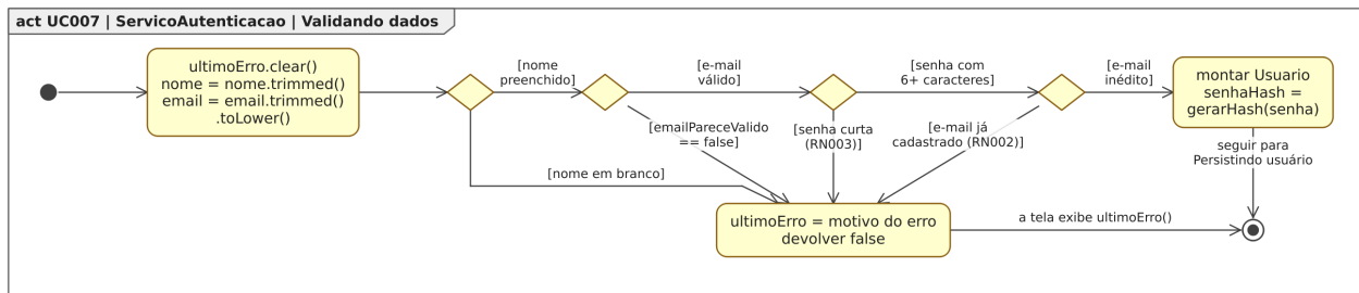
Figura 111. Diagrama de Atividades para o estado “Validando dados”, dentro do Diagrama de Estados para a classe ServicoAutenticacao em [UC007].
