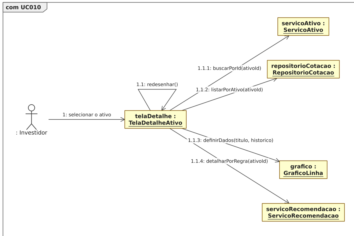
Figura 47. Diagrama de comunicação para o [UC010].
