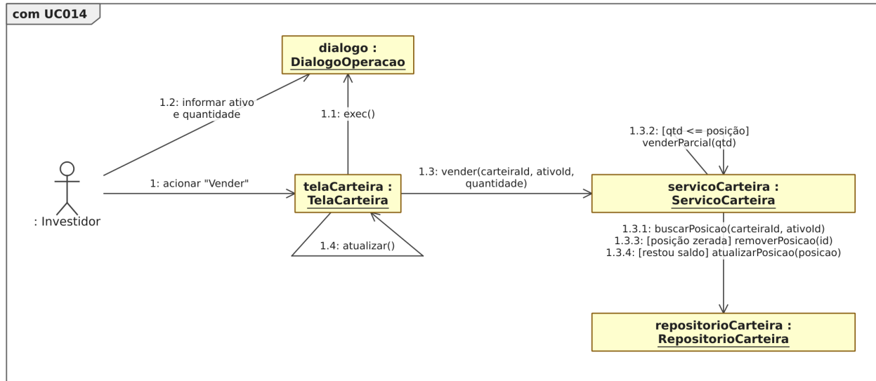
Figura 51. Diagrama de comunicação para o [UC014].
