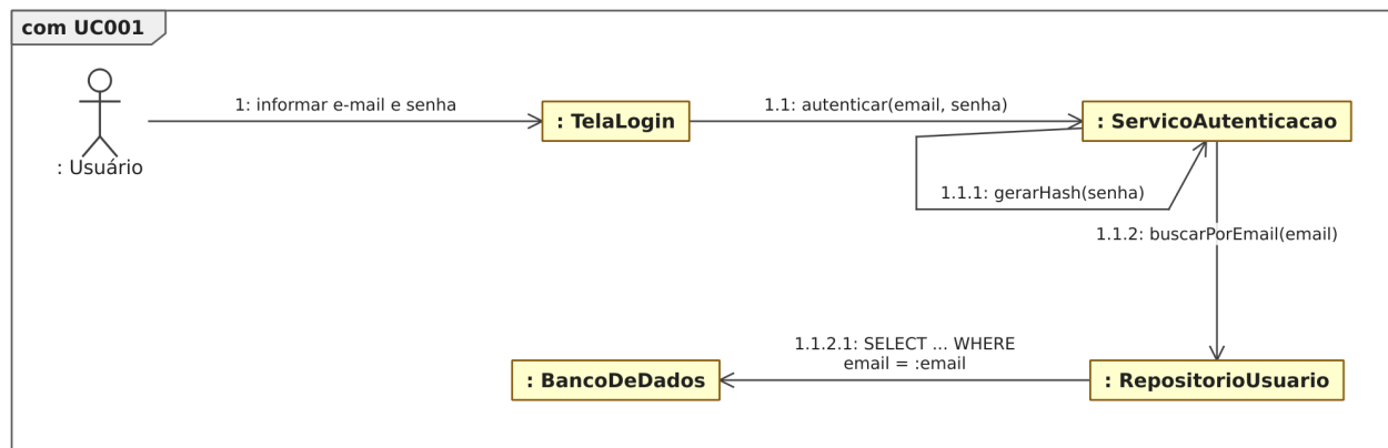
Figura 38. Diagrama de comunicação para o [UC001].
