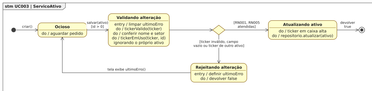
Figura 62. Diagrama de Estados da classe ServicoAtivo para o [UC003].
