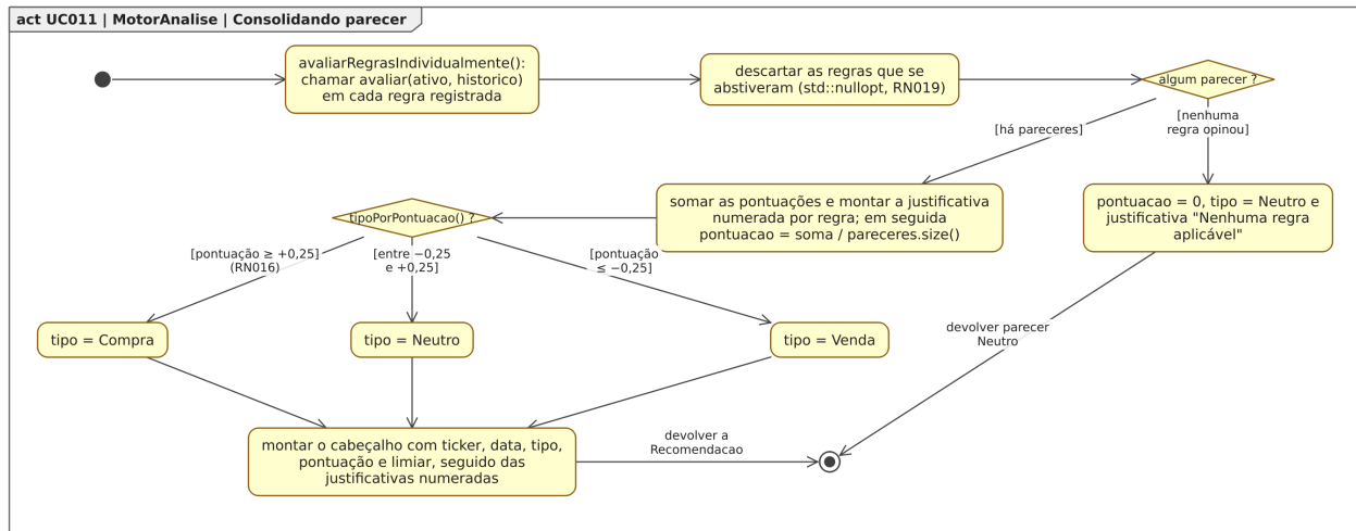
Figura 119. Diagrama de Atividades para o estado “Consolidando parecer”, dentro do Diagrama de Estados para a classe MotorAnalise em [UC011].
