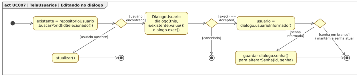
Figura 110. Diagrama de Atividades para o estado “Editando no diálogo”, dentro do Diagrama de Estados para a classe TelaUsuarios em [UC007].
