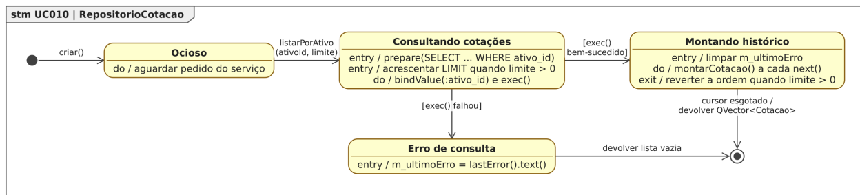
Figura 77. Diagrama de Estados da classe RepositorioCotacao para o [UC010].
