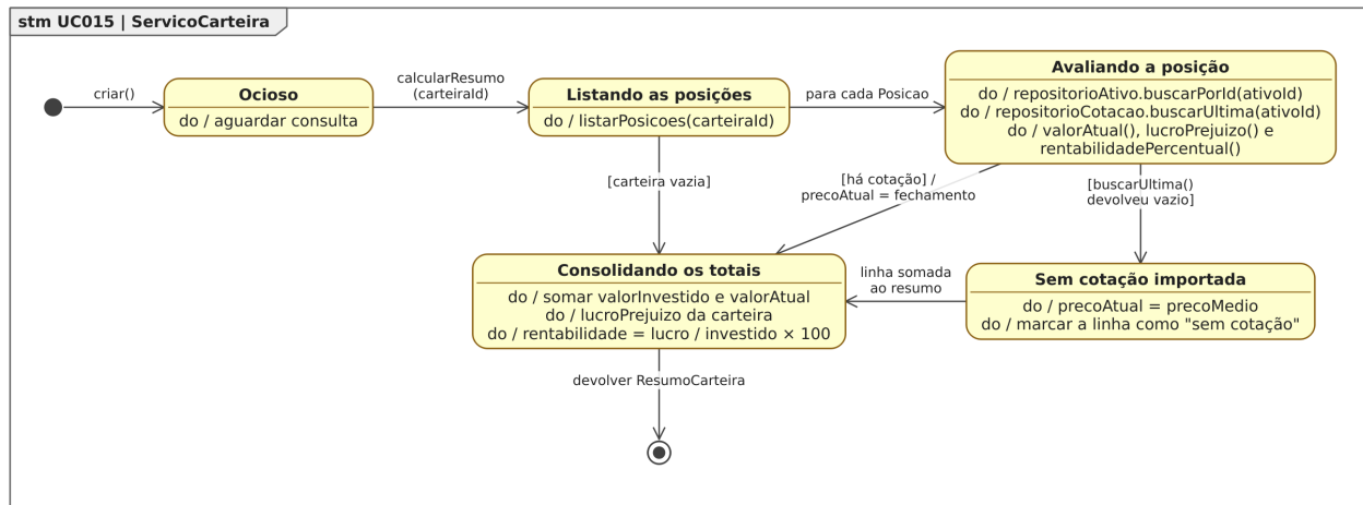
Figura 89. Diagrama de Estados da classe ServicoCarteira para o [UC015].
