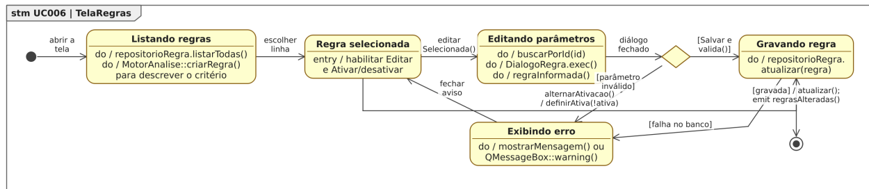
Figura 68. Diagrama de Estados da classe TelaRegras para o [UC006].
