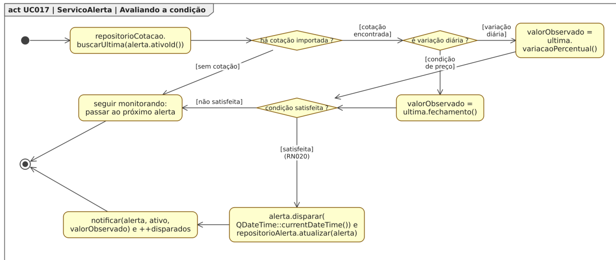
Figura 133. Diagrama de Atividades para o estado “Avaliando a condição”, dentro do Diagrama de Estados para a classe ServicoAlerta em [UC017].
