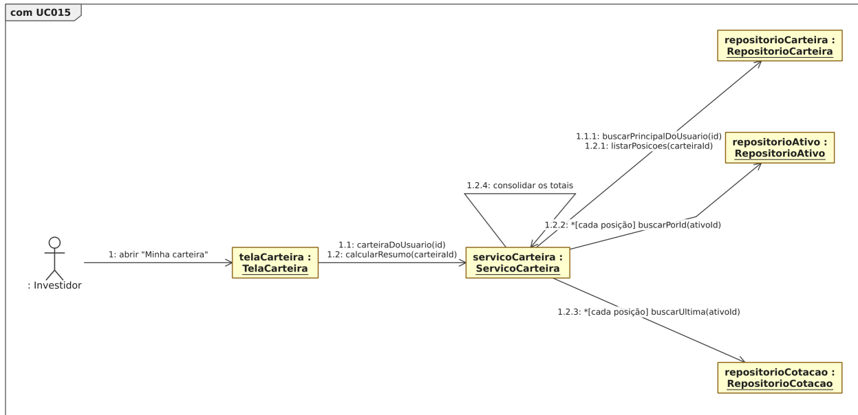
Figura 52. Diagrama de comunicação para o [UC015].
