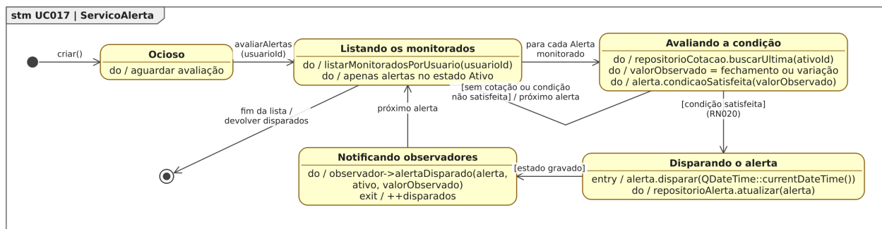
Figura 93. Diagrama de Estados da classe ServicoAlerta para o [UC017].
