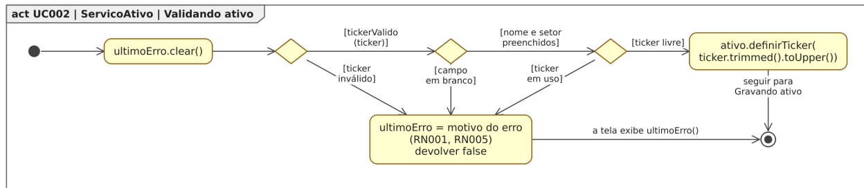
Figura 100. Diagrama de Atividades para o estado “Validando ativo”, dentro do Diagrama de Estados para a classe ServicoAtivo em [UC002].
