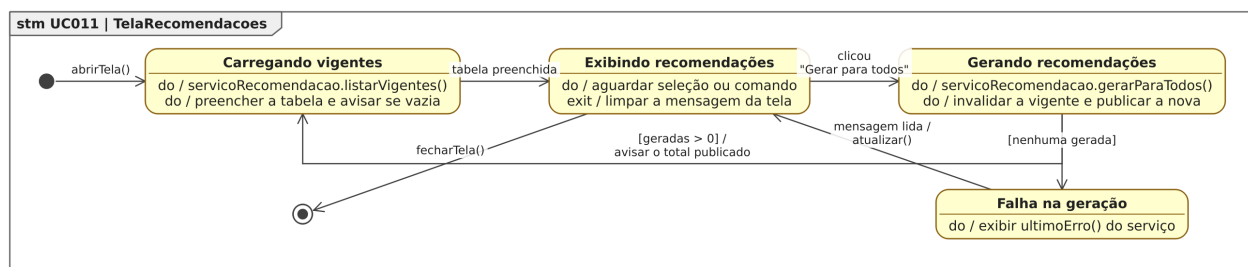
Figura 78. Diagrama de Estados da classe TelaRecomendacoes para o [UC011].
