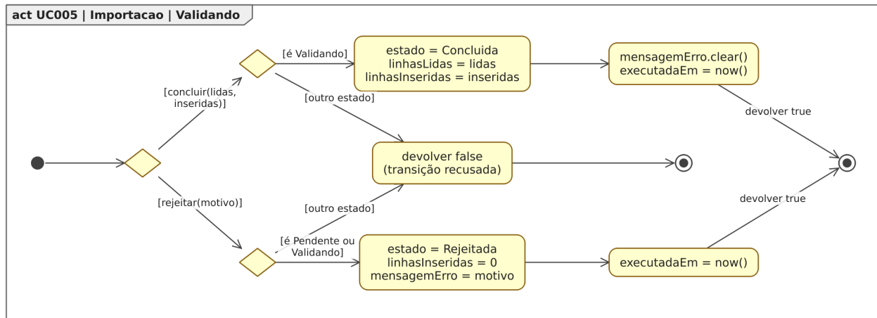
Figura 107. Diagrama de Atividades para o estado “Validando”, dentro do Diagrama de Estados para a classe Importacao em [UC005].
