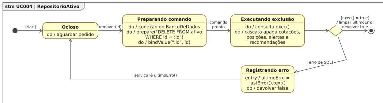
Figura 64. Diagrama de Estados da classe RepositorioAtivo para o [UC004].
