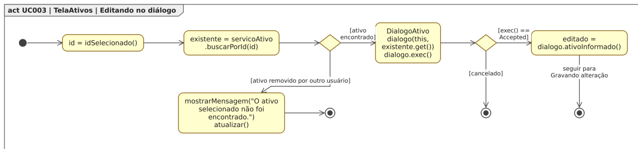
Figura 101. Diagrama de Atividades para o estado “Editando no diálogo”, dentro do Diagrama de Estados para a classe TelaAtivos em [UC003].
