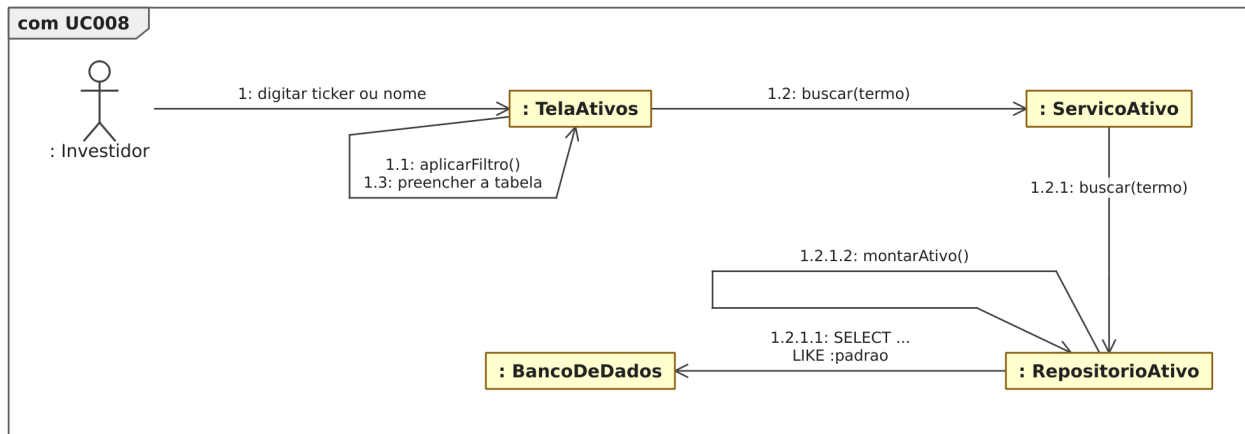
Figura 45. Diagrama de comunicação para o [UC008].
