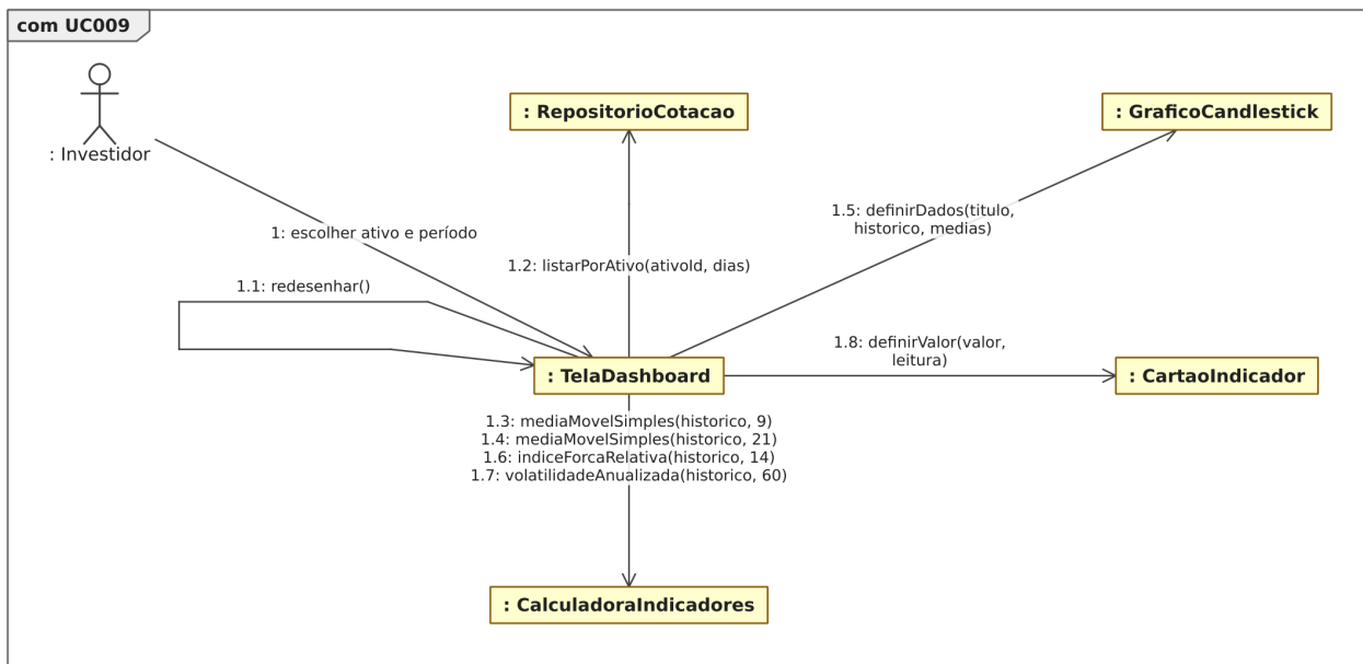
Figura 46. Diagrama de comunicação para o [UC009].
