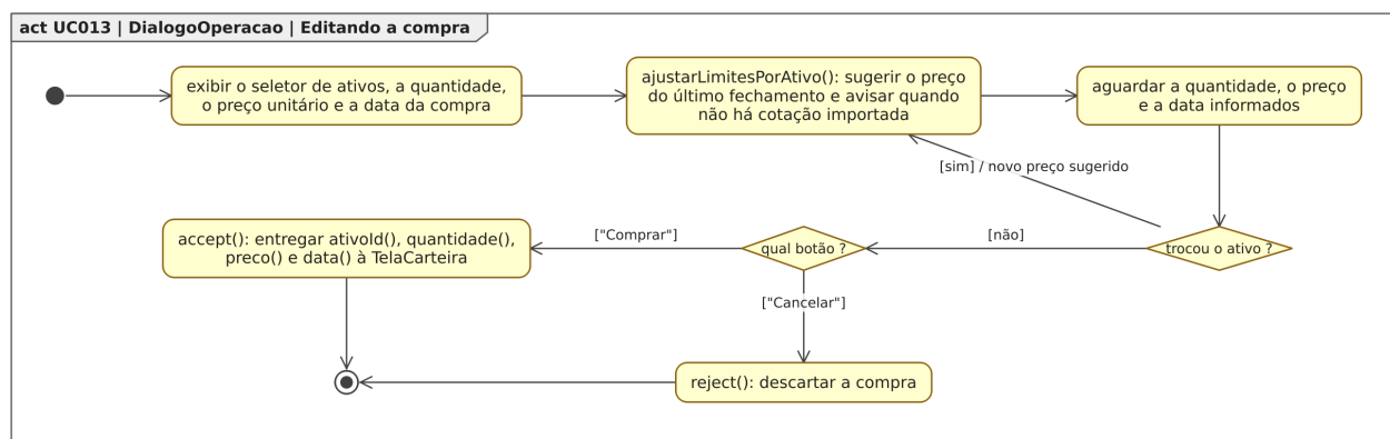
Figura 123. Diagrama de Atividades para o estado “Editando a compra”, dentro do Diagrama de Estados para a classe DialogoOperacao em [UC013].
