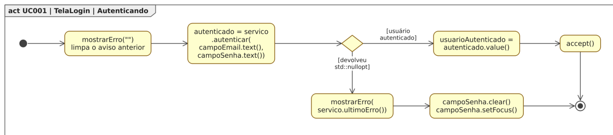
Figura 97. Diagrama de Atividades para o estado “Autenticando”, dentro do Diagrama de Estados para a classe TelaLogin em [UC001].
