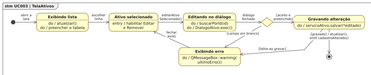
Figura 61. Diagrama de Estados da classe TelaAtivos para o [UC003].
