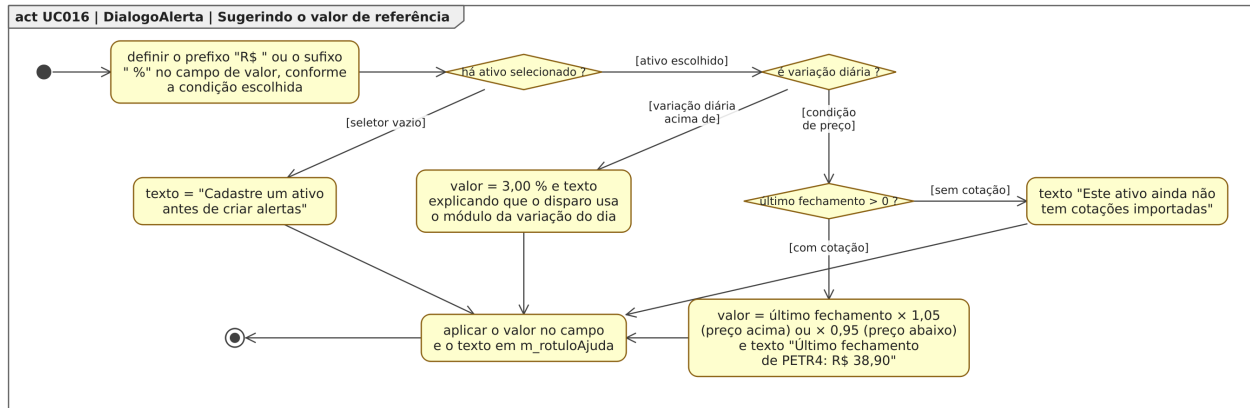
Figura 130. Diagrama de Atividades para o estado “Sugerindo o valor de referência”, dentro do Diagrama de Estados para a classe DialogoAlerta em [UC016].
