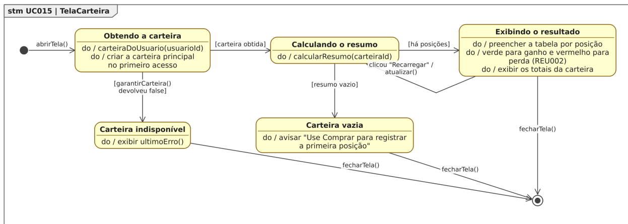
Figura 88. Diagrama de Estados da classe TelaCarteira para o [UC015].
