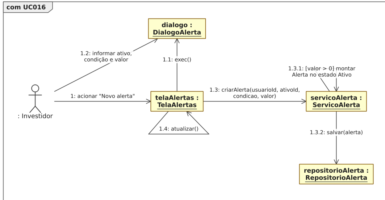
Figura 53. Diagrama de comunicação para o [UC016].
