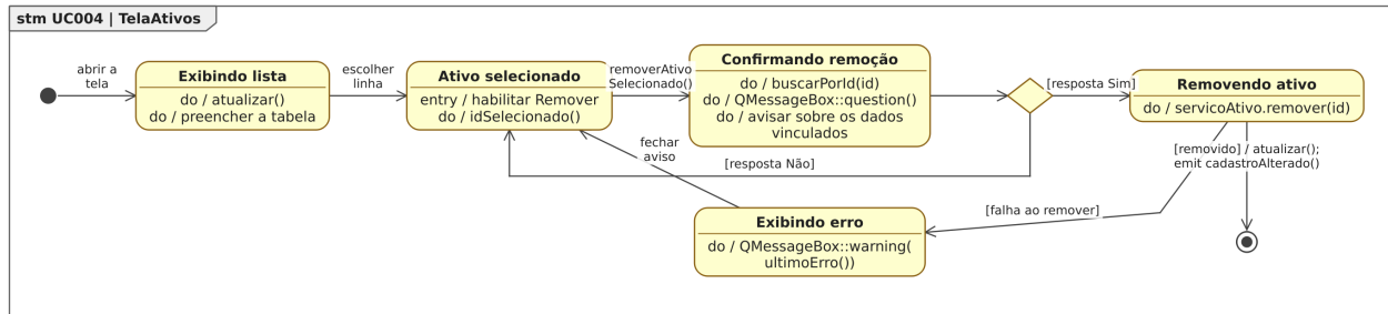
Figura 63. Diagrama de Estados da classe TelaAtivos para o [UC004].
