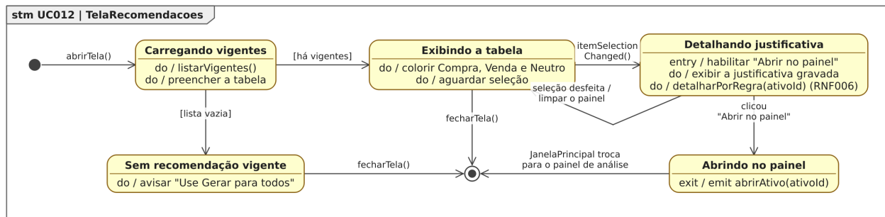
Figura 81. Diagrama de Estados da classe TelaRecomendacoes para o [UC012].
