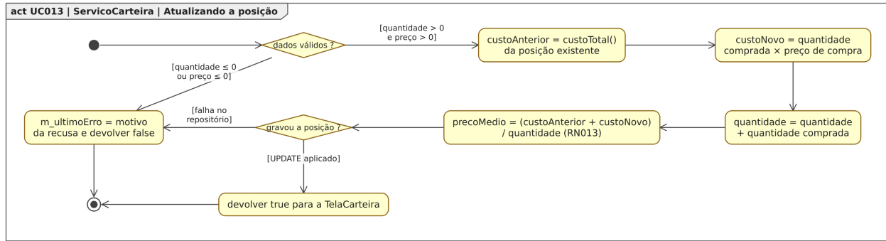
Figura 124. Diagrama de Atividades para o estado “Atualizando a posição”, dentro do Diagrama de Estados para a classe ServicoCarteira em [UC013].
