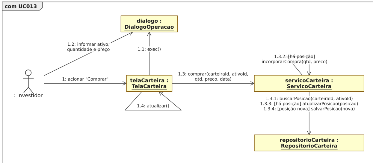
Figura 50. Diagrama de comunicação para o [UC013].
