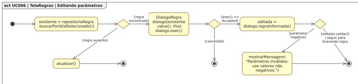
Figura 108. Diagrama de Atividades para o estado “Editando parâmetros”, dentro do Diagrama de Estados para a classe TelaRegras em [UC006].
