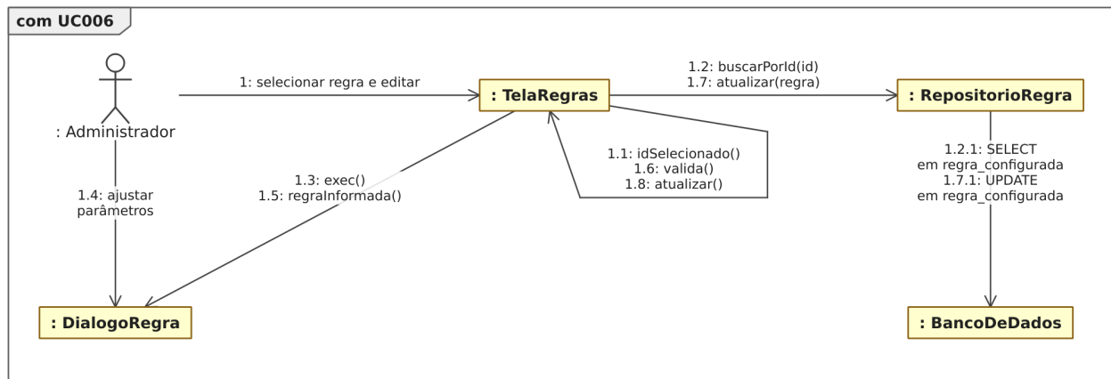
Figura 43. Diagrama de comunicação para o [UC006].
