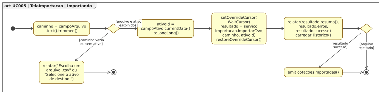
Figura 105. Diagrama de Atividades para o estado “Importando”, dentro do Diagrama de Estados para a classe TelaImportacao em [UC005].
