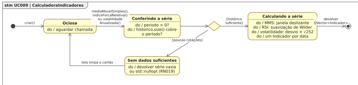
Figura 75. Diagrama de Estados da classe CalculadoraIndicadores para o [UC009].
