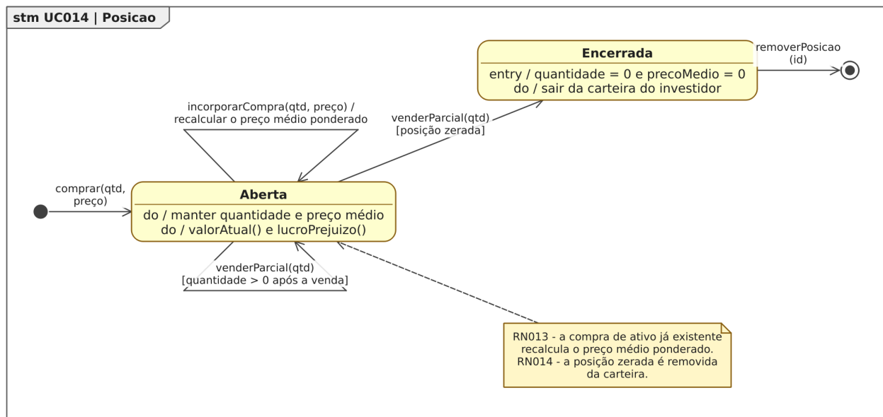
Figura 87. Diagrama de Estados da classe Posicao para o [UC014].
