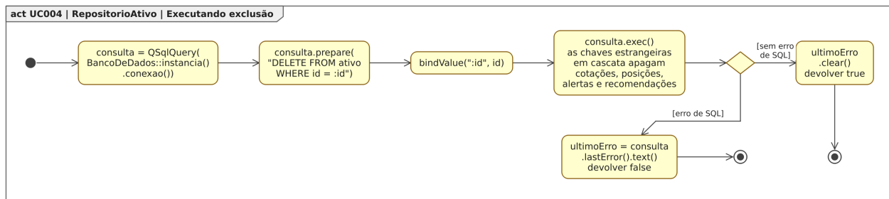
Figura 104. Diagrama de Atividades para o estado “Executando exclusão”, dentro do Diagrama de Estados para a classe RepositorioAtivo em [UC004].
