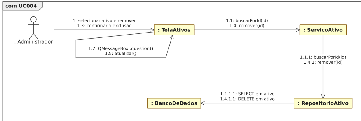
Figura 41. Diagrama de comunicação para o [UC004].
