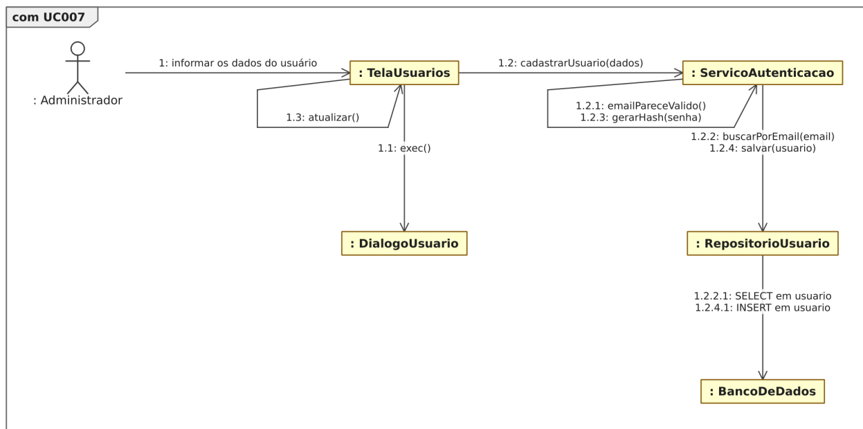
Figura 44. Diagrama de comunicação para o [UC007].
