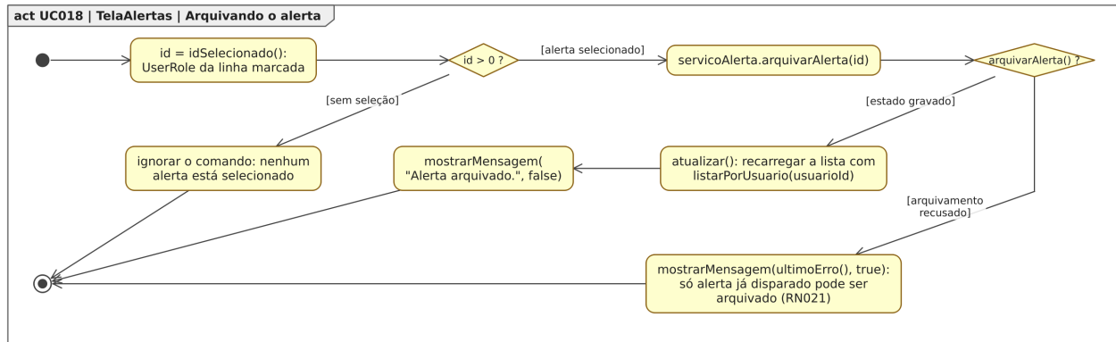
Figura 135. Diagrama de Atividades para o estado “Arquivando o alerta”, dentro do Diagrama de Estados para a classe TelaAlertas em [UC018].
