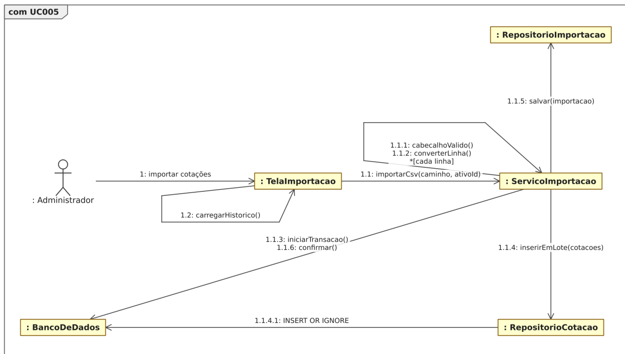
Figura 42. Diagrama de comunicação para o [UC005].
