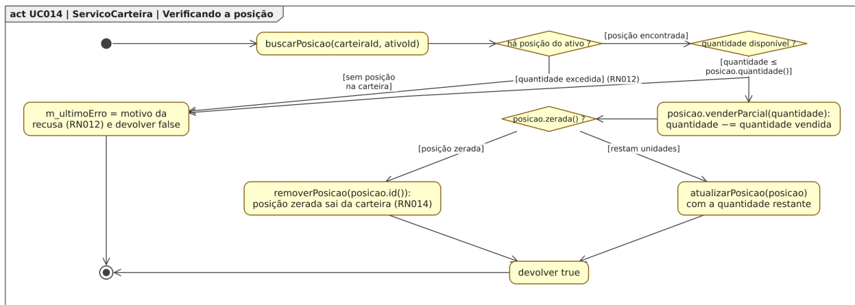
Figura 126. Diagrama de Atividades para o estado “Verificando a posição”, dentro do Diagrama de Estados para a classe ServicoCarteira em [UC014].
