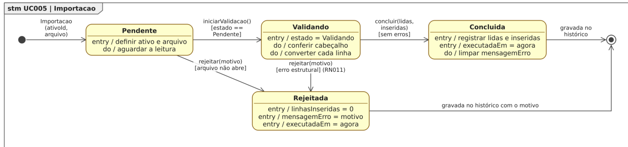
Figura 67. Diagrama de Estados da classe Importacao para o [UC005].
