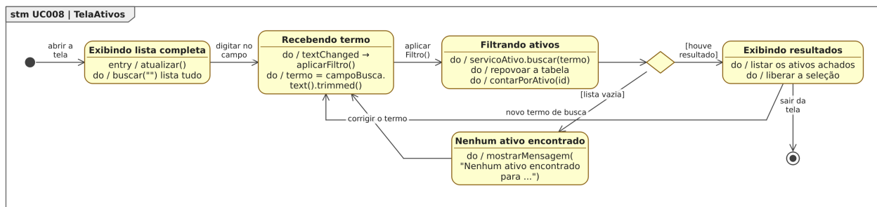
Figura 72. Diagrama de Estados da classe TelaAtivos para o [UC008].
