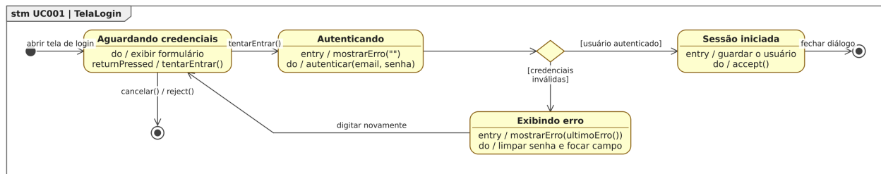
Figura 57. Diagrama de Estados da classe TelaLogin para o [UC001].
