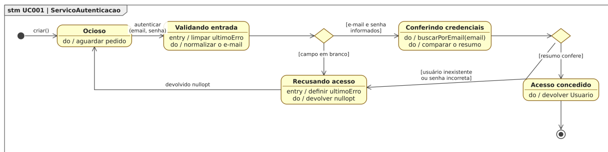
Figura 58. Diagrama de Estados da classe ServicoAutenticacao para o [UC001].
