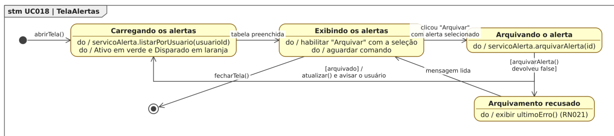
Figura 95. Diagrama de Estados da classe TelaAlertas para o [UC018].
