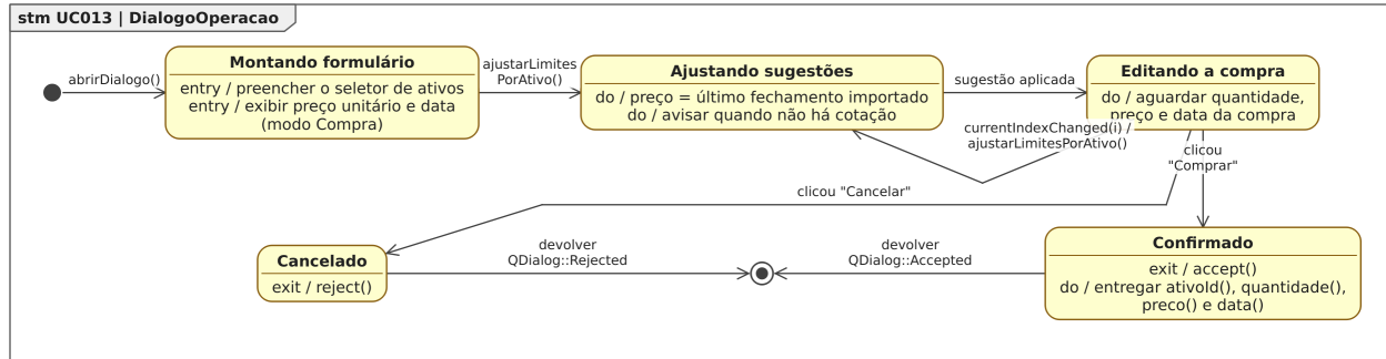
Figura 83. Diagrama de Estados da classe DialogoOperacao para o [UC013].
