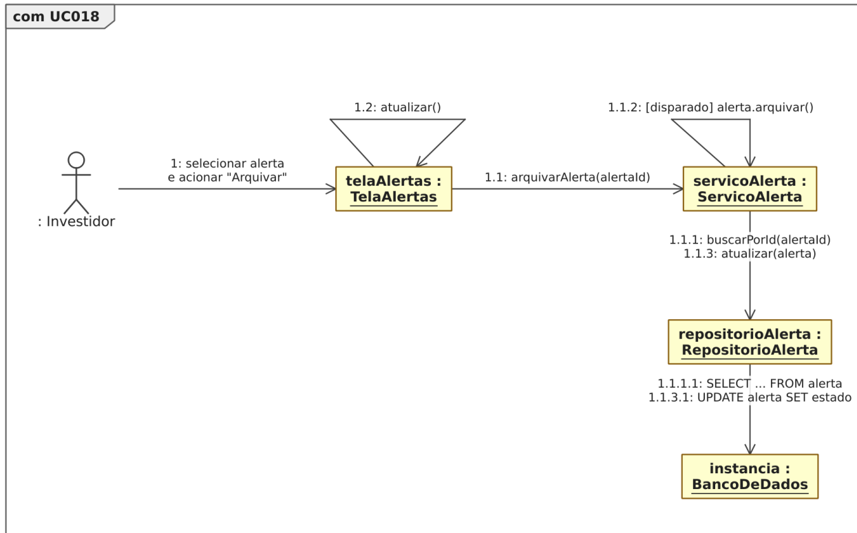
Figura 55. Diagrama de comunicação para o [UC018].
