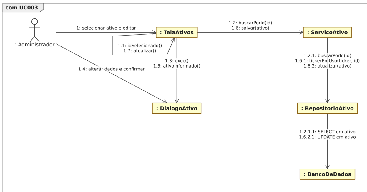
Figura 40. Diagrama de comunicação para o [UC003].
