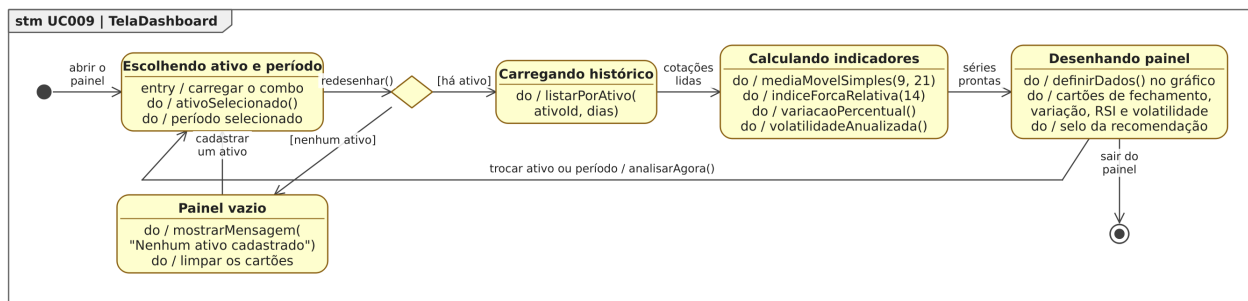
Figura 74. Diagrama de Estados da classe TelaDashboard para o [UC009].
