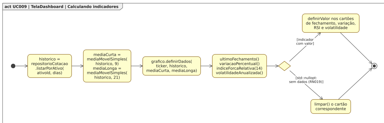
Figura 114. Diagrama de Atividades para o estado “Calculando indicadores”, dentro do Diagrama de Estados para a classe TelaDashboard em [UC009].
