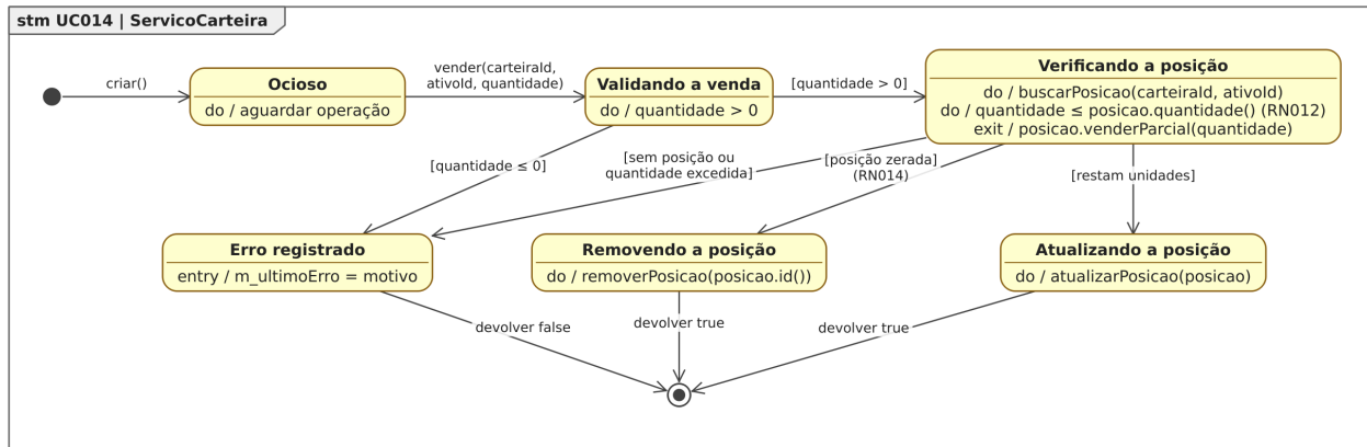
Figura 86. Diagrama de Estados da classe ServicoCarteira para o [UC014].
