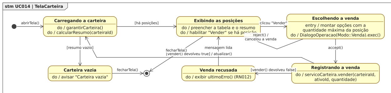
Figura 85. Diagrama de Estados da classe TelaCarteira para o [UC014].
