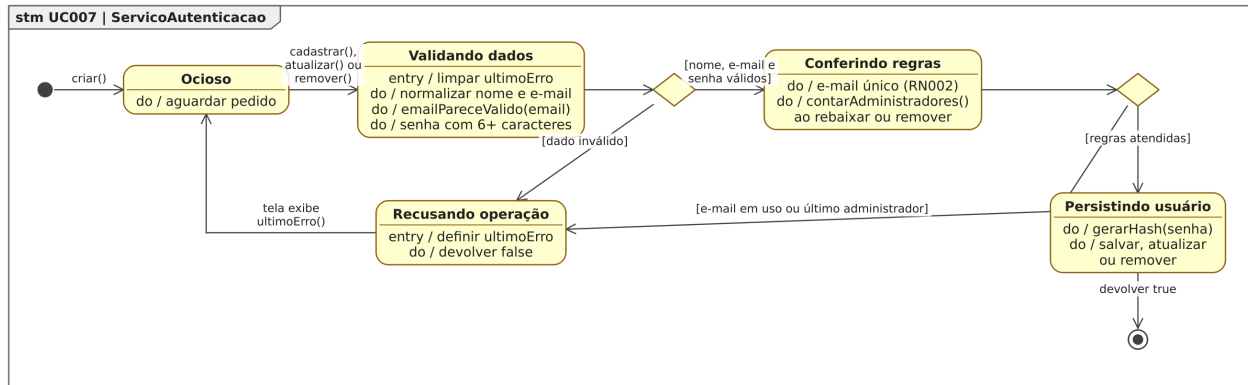
Figura 71. Diagrama de Estados da classe ServicoAutenticacao para o [UC007].
