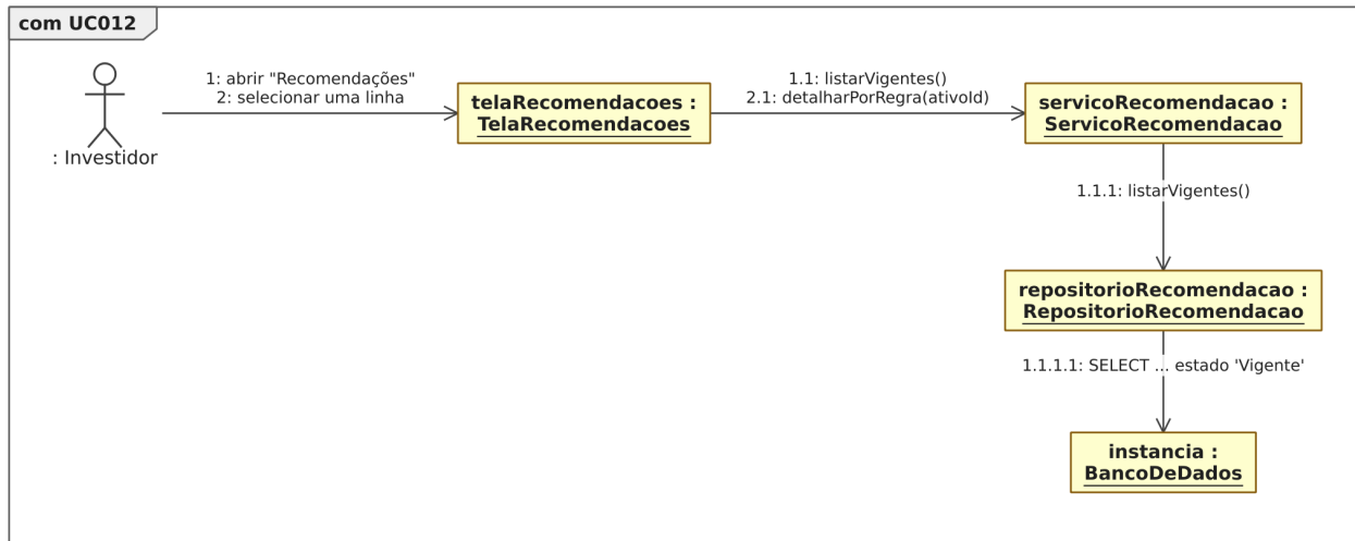
Figura 49. Diagrama de comunicação para o [UC012].
