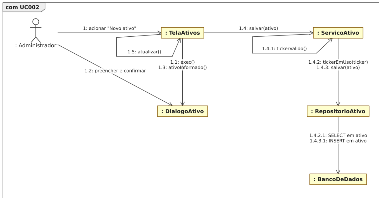
Figura 39. Diagrama de comunicação para o [UC002].
