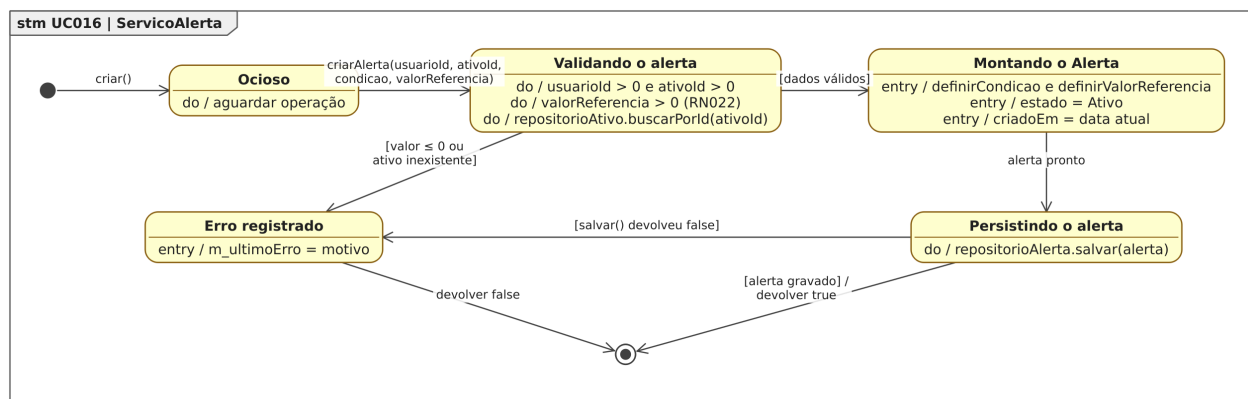
Figura 91. Diagrama de Estados da classe ServicoAlerta para o [UC016].
