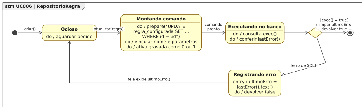
Figura 69. Diagrama de Estados da classe RepositorioRegra para o [UC006].
