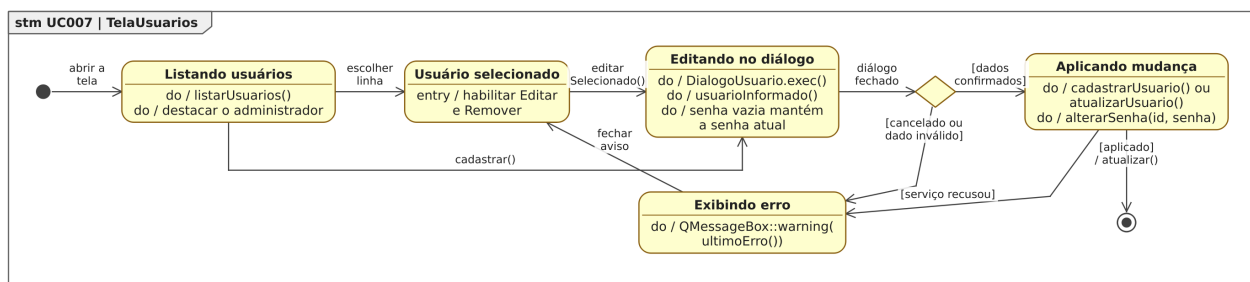
Figura 70. Diagrama de Estados da classe TelaUsuarios para o [UC007].
