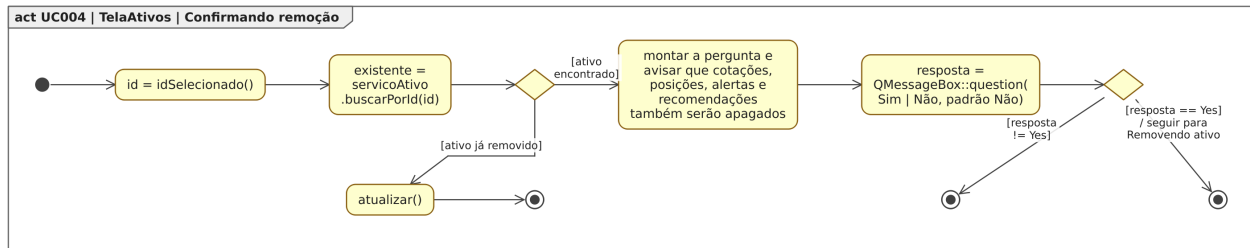
Figura 103. Diagrama de Atividades para o estado “Confirmando remoção”, dentro do Diagrama de Estados para a classe TelaAtivos em [UC004].
