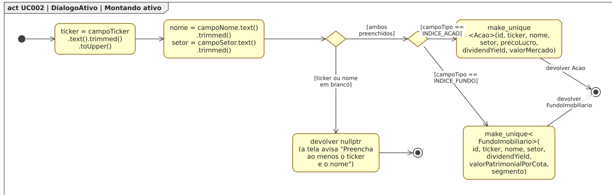
Figura 99. Diagrama de Atividades para o estado “Montando ativo”, dentro do Diagrama de Estados para a classe DialogoAtivo em [UC002].
