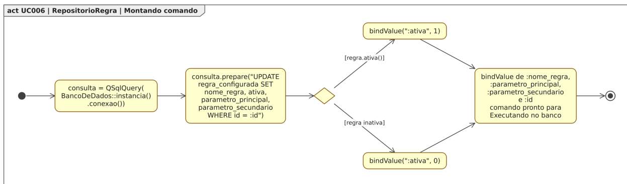
Figura 109. Diagrama de Atividades para o estado “Montando comando”, dentro do Diagrama de Estados para a classe RepositorioRegra em [UC006].
