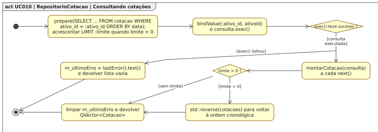
Figura 117. Diagrama de Atividades para o estado “Consultando cotações”, dentro do Diagrama de Estados para a classe RepositorioCotacao em [UC010].
