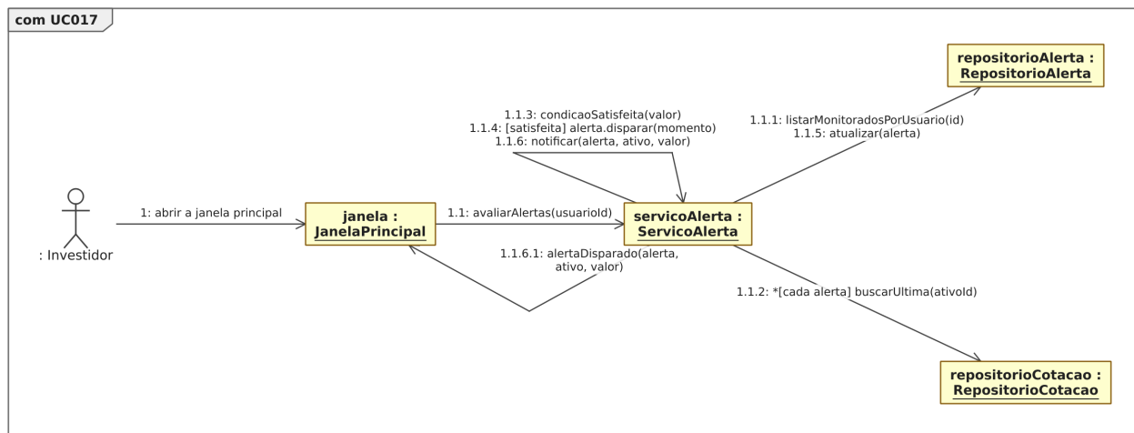
Figura 54. Diagrama de comunicação para o [UC017].
