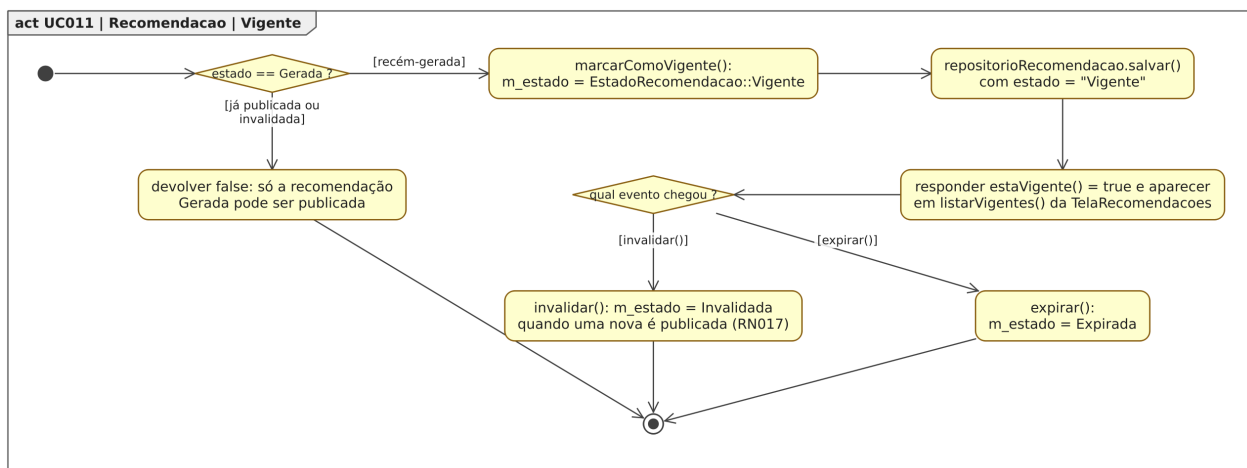
Figura 120. Diagrama de Atividades para o estado “Vigente”, dentro do Diagrama de Estados para a classe Recomendacao em [UC011].
