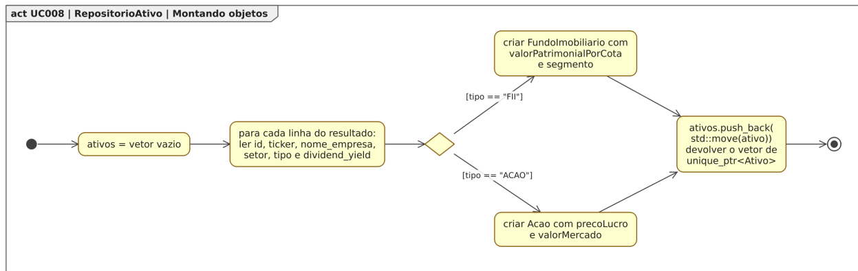
Figura 113. Diagrama de Atividades para o estado “Montando objetos”, dentro do Diagrama de Estados para a classe RepositorioAtivo em [UC008].
