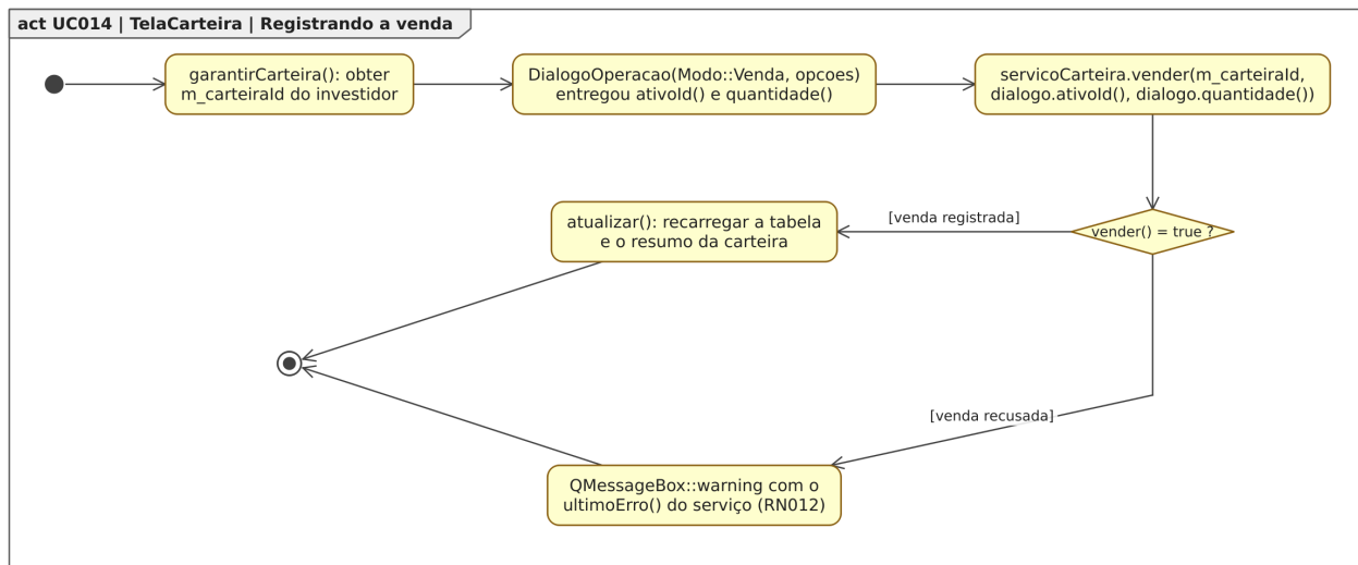
Figura 125. Diagrama de Atividades para o estado “Registrando a venda”, dentro do Diagrama de Estados para a classe TelaCarteira em [UC014].
