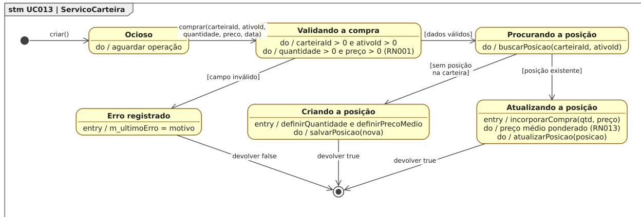
Figura 84. Diagrama de Estados da classe ServicoCarteira para o [UC013].
