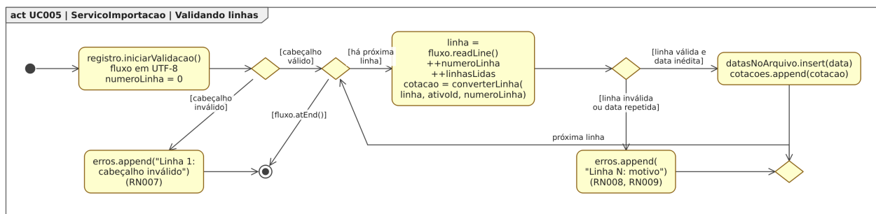
Figura 106. Diagrama de Atividades para o estado “Validando linhas”, dentro do Diagrama de Estados para a classe ServicoImportacao em [UC005].
