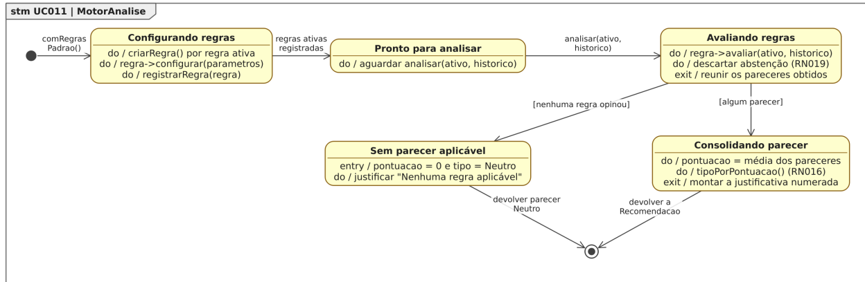
Figura 79. Diagrama de Estados da classe MotorAnalise para o [UC011].
