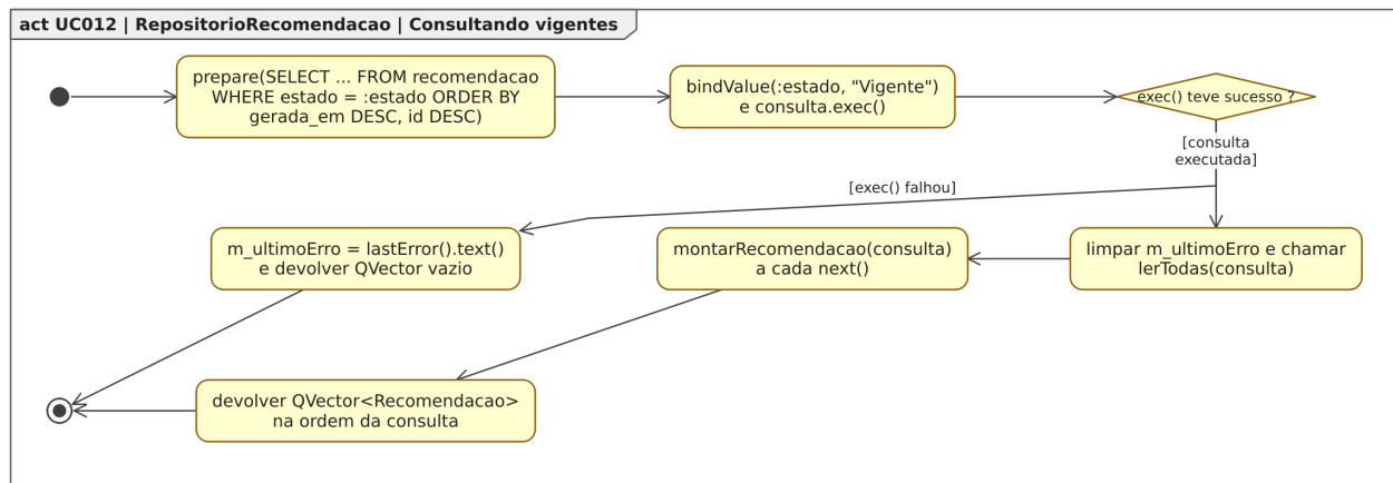
Figura 122. Diagrama de Atividades para o estado “Consultando vigentes”, dentro do Diagrama de Estados para a classe RepositorioRecomendacao em [UC012].
