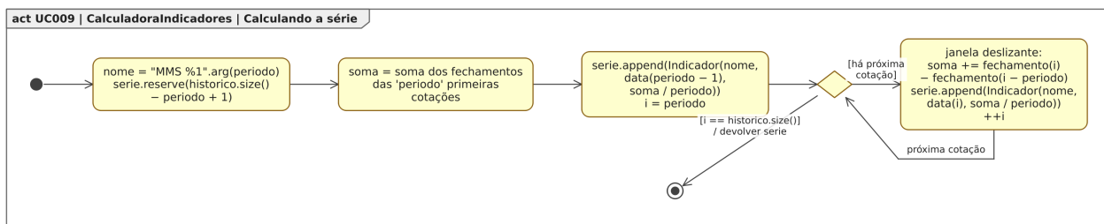
Figura 115. Diagrama de Atividades para o estado “Calculando a série”, dentro do Diagrama de Estados para a classe CalculadoraIndicadores em [UC009].
