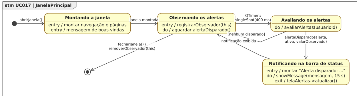
Figura 92. Diagrama de Estados da classe JanelaPrincipal para o [UC017].
