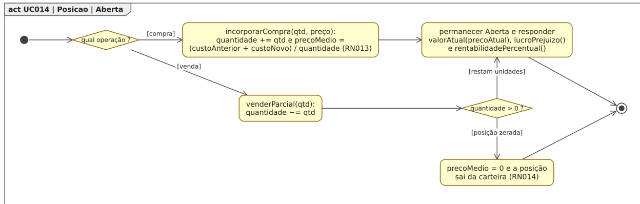
Figura 127. Diagrama de Atividades para o estado “Aberta”, dentro do Diagrama de Estados para a classe Posicao em [UC014].
