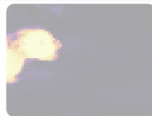
DINOv3
