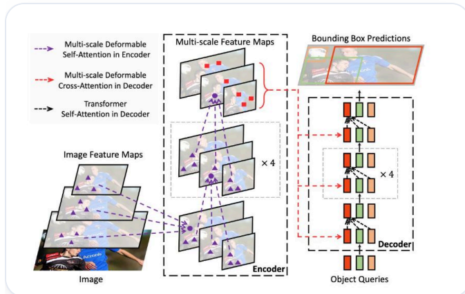
Figura de Deformable DETR (Zhu et al., 2021). RF-DETR conserva el decoder de la derecha y sustituye el encoder.
