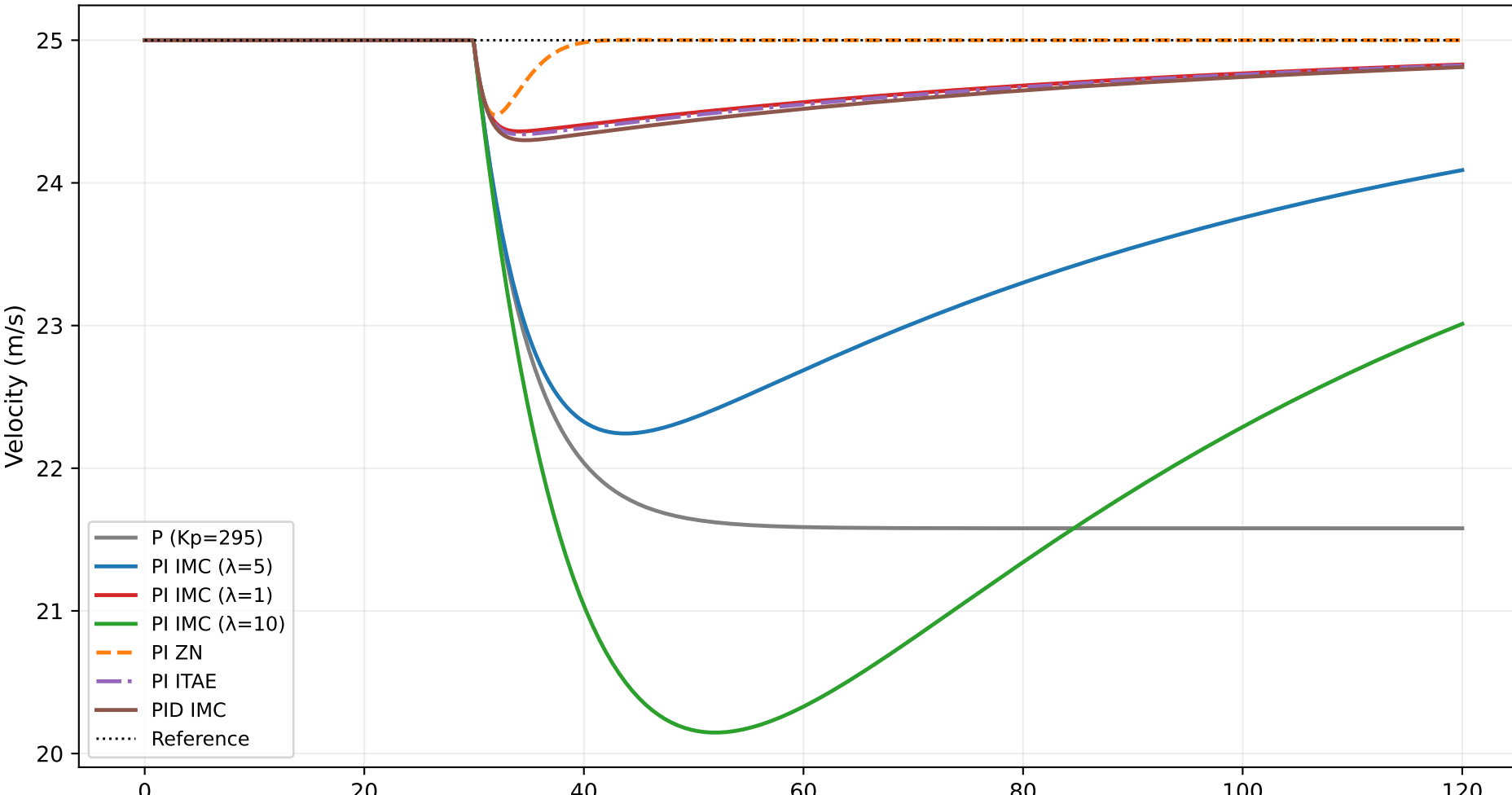
D1 disturbance rejection (linear)
