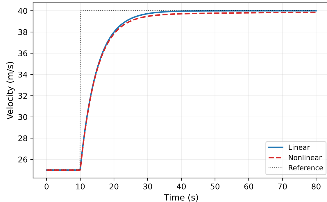
Step +15 m/s
