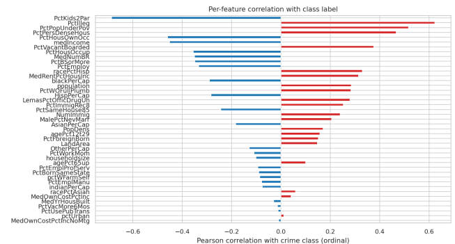
FIGURE 5. 43 özelliğin tamamının suç sınıfı (ordinal) ile özellik-başına Pearson korelasyonu, sıralanmış halde. Kırmızı çubuklar yüksek suç düzeyleriyle pozitif korelasyonu, mavi çubuklar negatif (koruyucu) korelasyonu gösterir.
