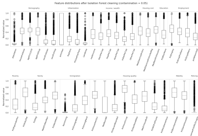
FIGURE 3. Isolation Forest temizliği (kirlilik = 0.05) sonrası kutu grafikleri. Her dağılımın ana gövdesi korunur, ancak marjinal aykırı değer noktaları (bıyıkların ötesindeki daireler) hâlâ görünürdü – detektörün özellikle-başına uç değerleri değil birleşik anomalileri kaldırdığını doğrudan görsel kanıtı.
