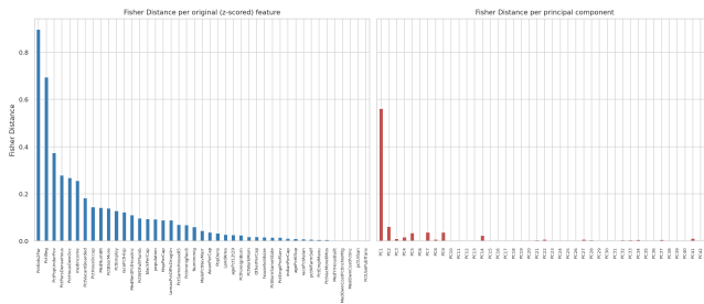
FIGURE 8. Z-skorlanmış orijinal özellik-başına (sol) ve temel bileşen-başına (sağ) Fisher Uzaklığı, ortak dikey ölçekte. Özellik-başına sinyal birkaç değişkene yayılırken, PC-başına sinyal neredeyse tamamen PC1'de yoğunlaşmıştır.
