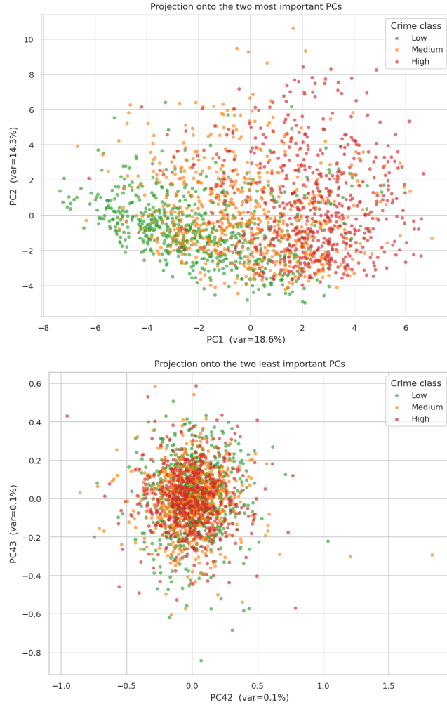
FIGURE 10. Üst: (PC1, PC2) üzerine projeksiyon. Yatay PC1 eksenine boyunca Düşük → Orta → Yüksek monoton bir sıralama belirirken, dikey PC2 eksenine hiçbir ayırım katmaz. Alt: en önemsiz iki PC (PC42, PC43) üzerine projeksiyon; hiçbir sınıf yapısı göstermez.
