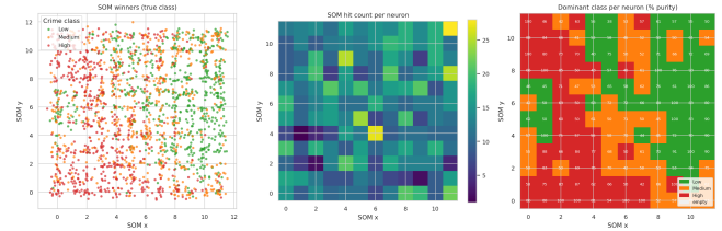
FIGURE 15. Orijinal z-skordanmış veride eğitilmiş 12 \times 12 MiniSom. Sol: kazananların gerçek sınıfa göre saçılımı (görünürlük için titrestirilmiş). Orta: nöron-başına vuruş-sayısı ısı haritası. Sağ: nöron-başına baskın sınıf ve hücre-başına saflık (metin etiketleri, % olarak); boş olmayan hücrelerin ortalama saflığı %67,5'tir.
