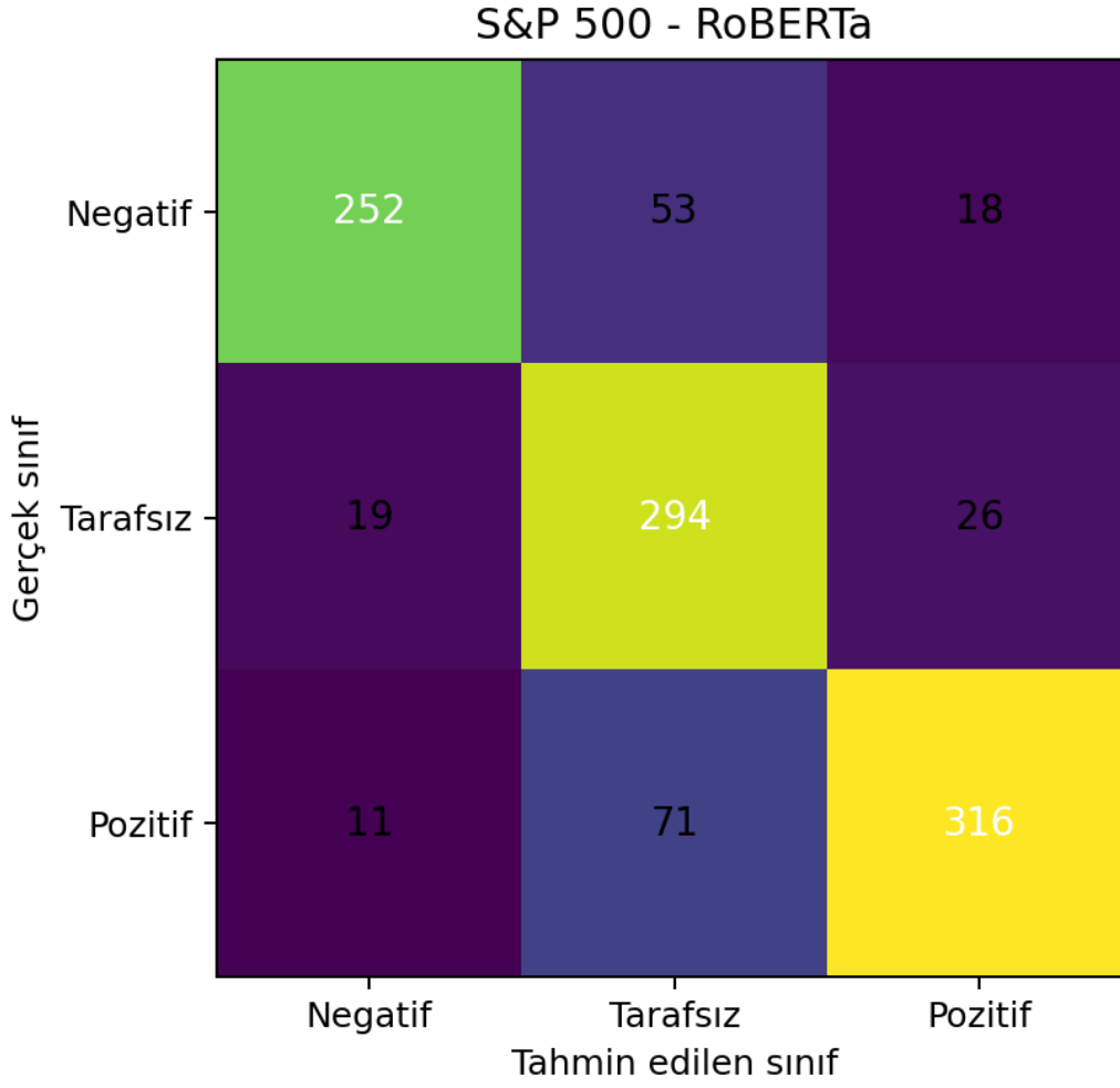
Şekil 5. S&P 500 - RoBERTa karışıklık matrisi
