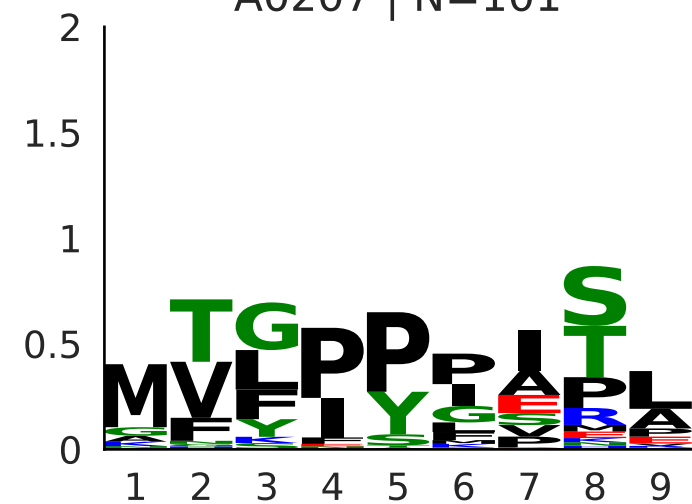
A0207 | N=101
