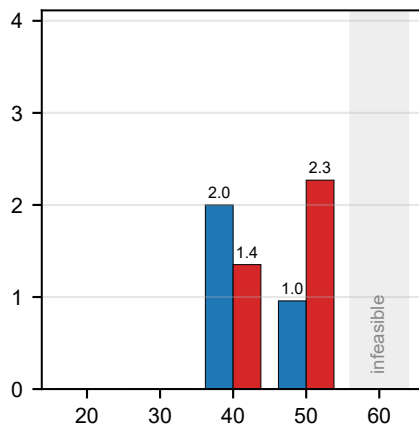
R717/R600
