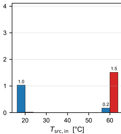
R717/R600
