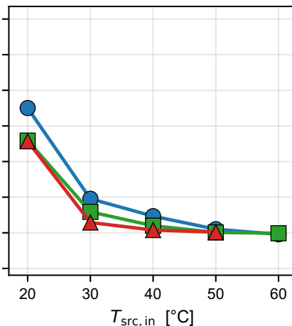
R717/R600
