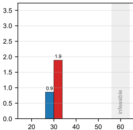
R717/R600
