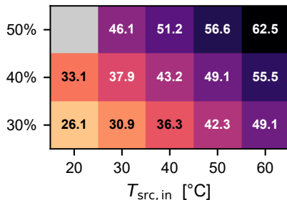
R717/R600
