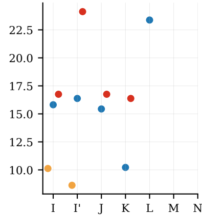
attn-logit max
