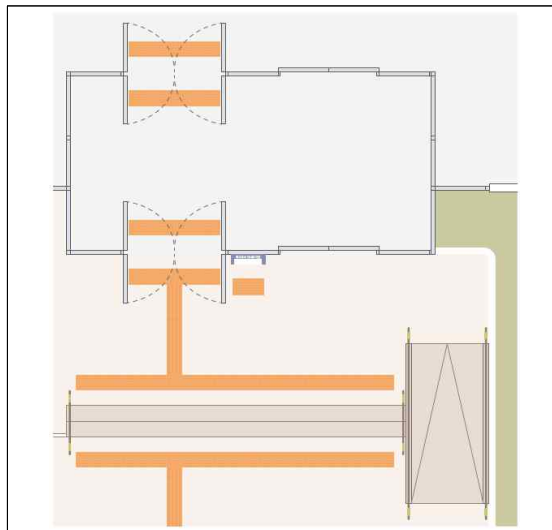
계단과 경사로가 같이 설치된 경우
