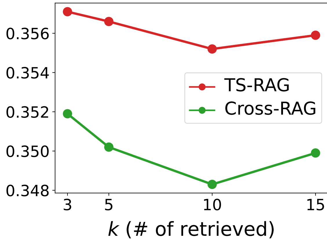
ETTh1
