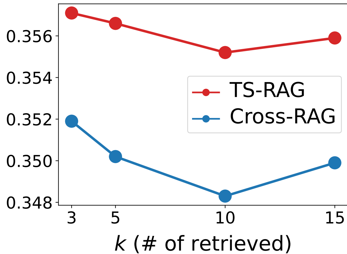
ETTh1
