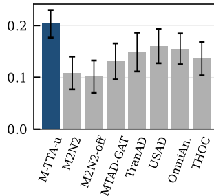
MSL — F1 @ unsupervised \tau
