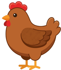
hen
