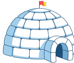
igloo
