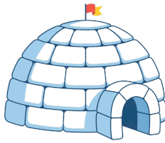
igloo
