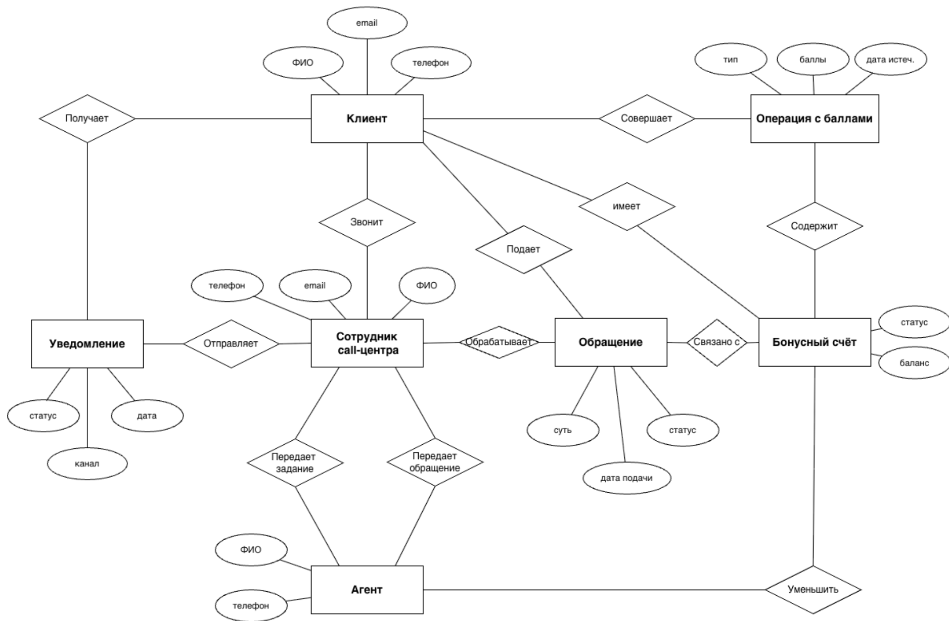
Рис. 1: ER-диаграмма
