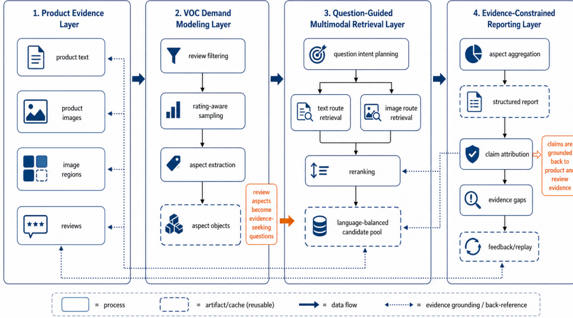
Figure 1: 그림 1. Decathlon VOC Analyzer 의 전체프레임워크. 시스템은상품증거패키지와리뷰측면을중간 표현으로사용하고, 질문계획을통해주관적 VOC 신호를멀티모달상품증거와연결하며, 보고단계에서 claim 수준귀속을수행한다.
