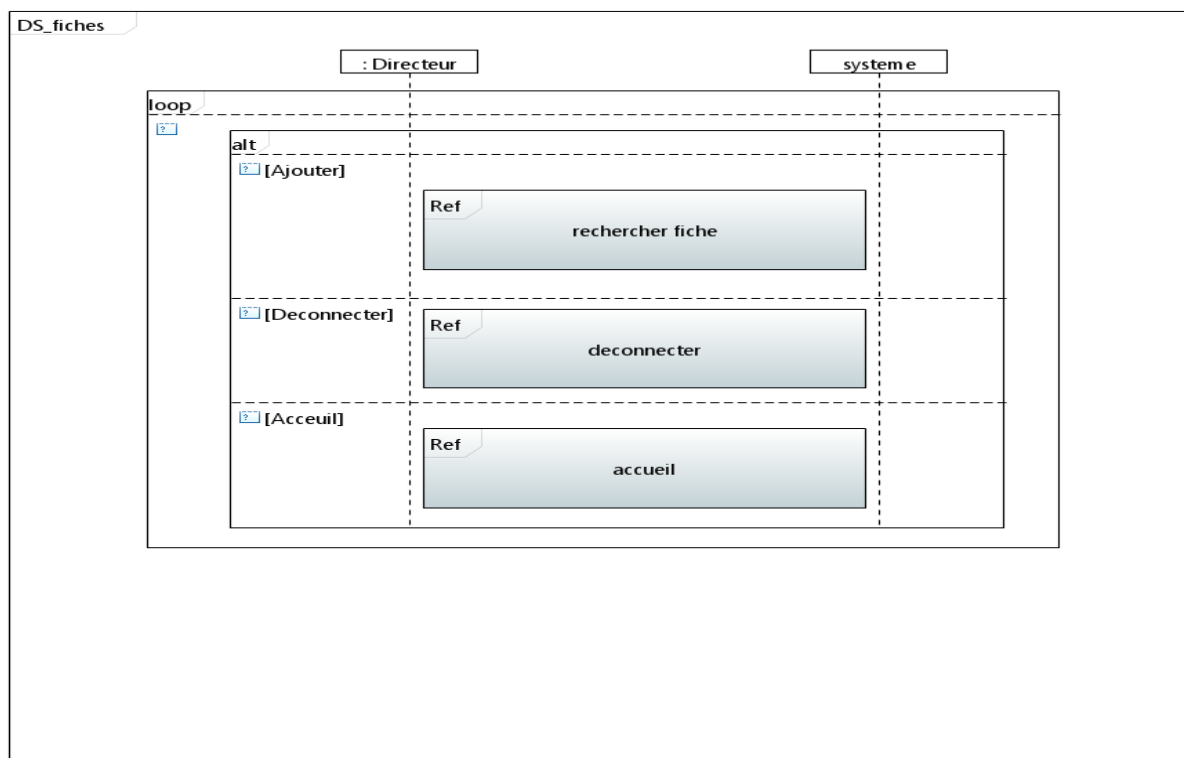
Figure 72 – Diagramme de rechercher fiches.
