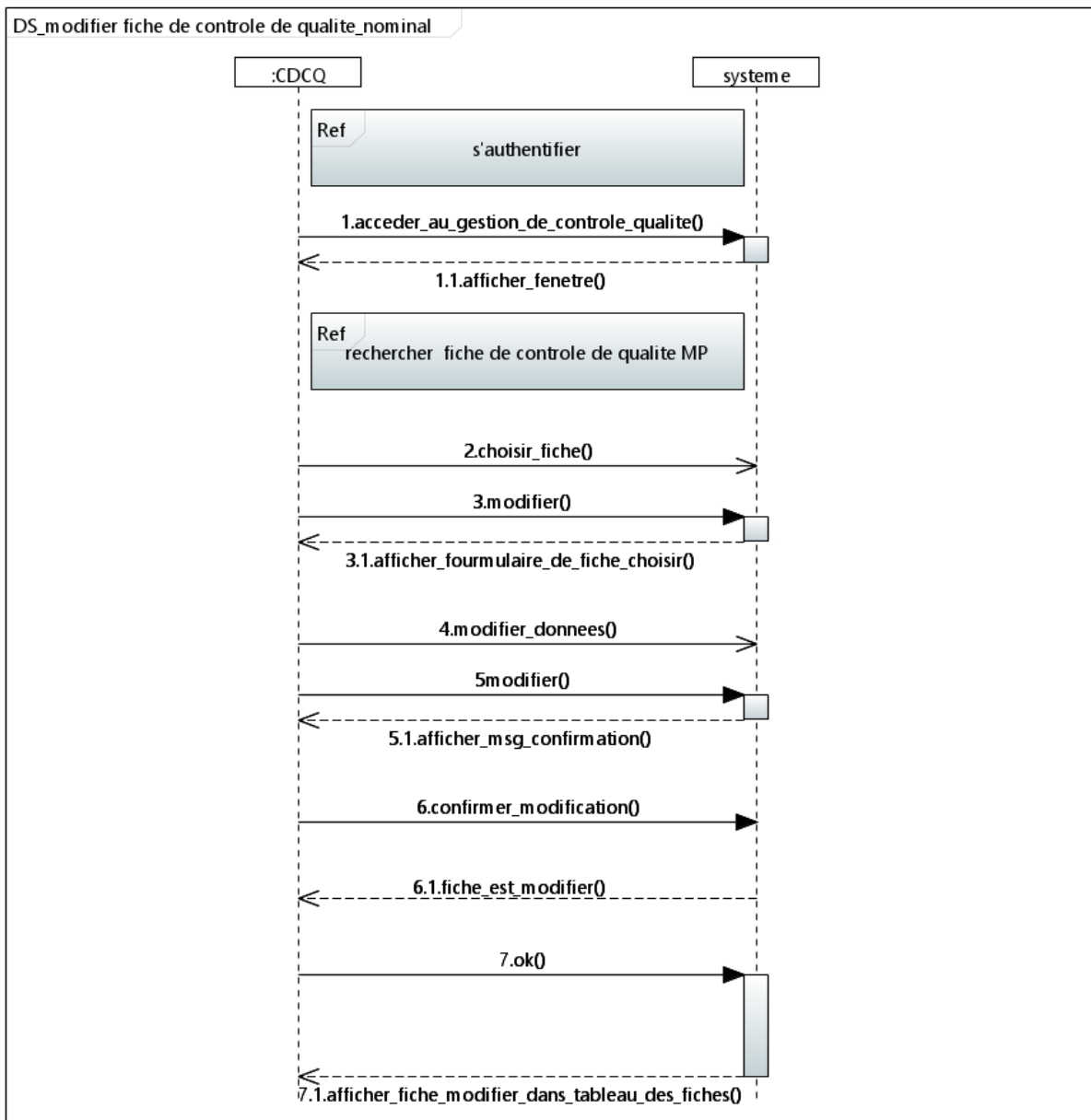
Figure 22 – Diagramme de séquence de modifier la fiche de contrôle des matières premières a la réception scenario nominal.
