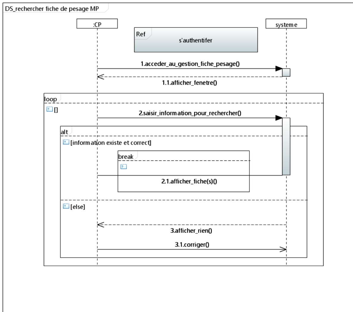
Figure 48 – Diagramme de séquence de rechercher fiche de pesage scenario nominal et alternatif.
