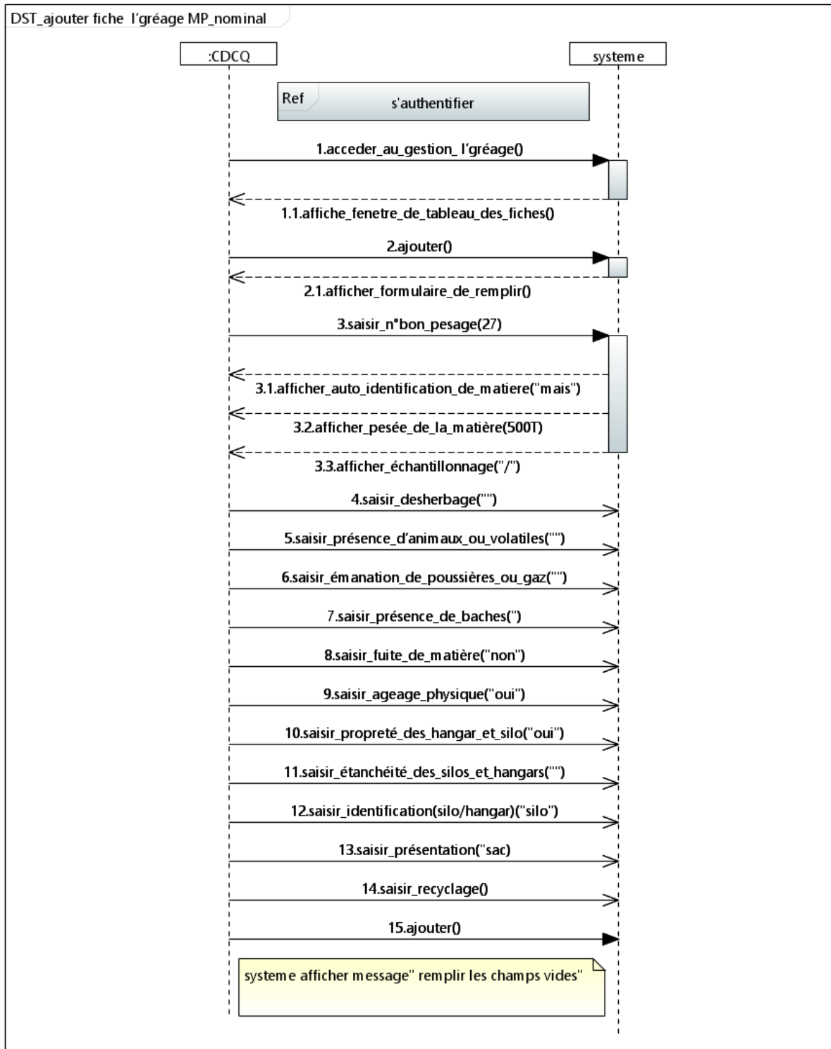
Figure 83- Diagramme de teste de fiche agreage1.
