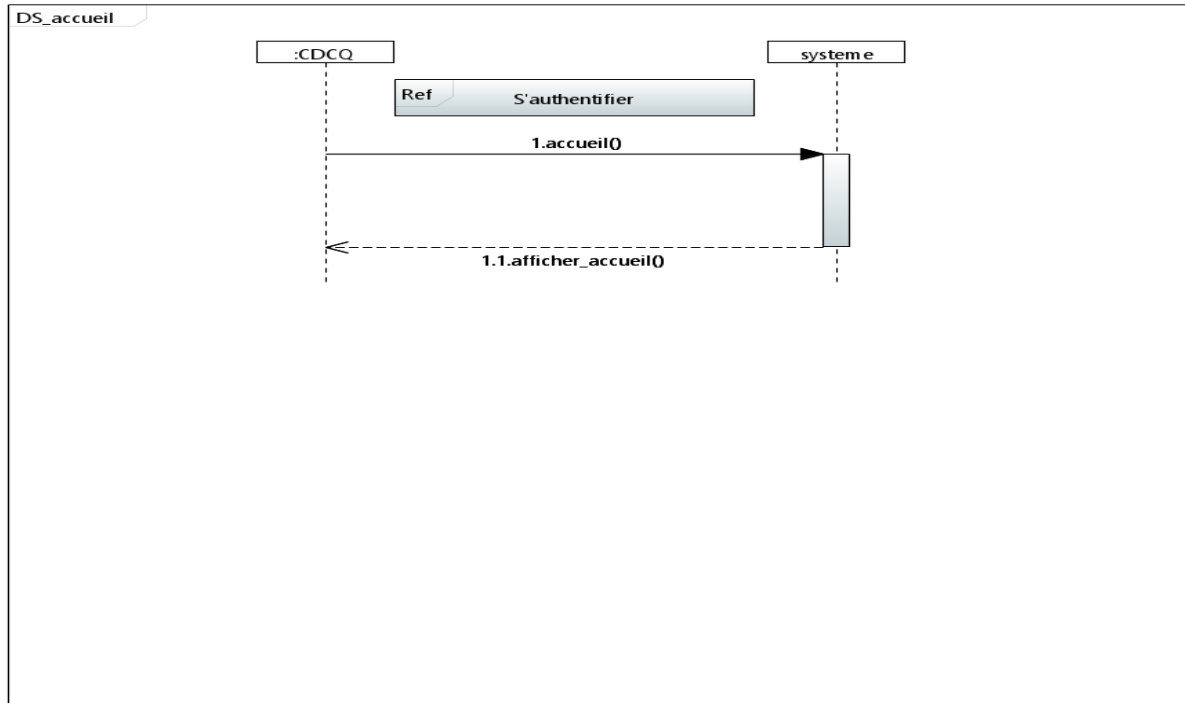
Figure 16 – Diagramme de séquence d'accueil.
