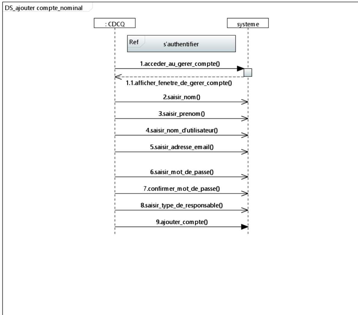
Figure 8 – Diagramme de séquence d’ajouter compte scenario Nominal.
