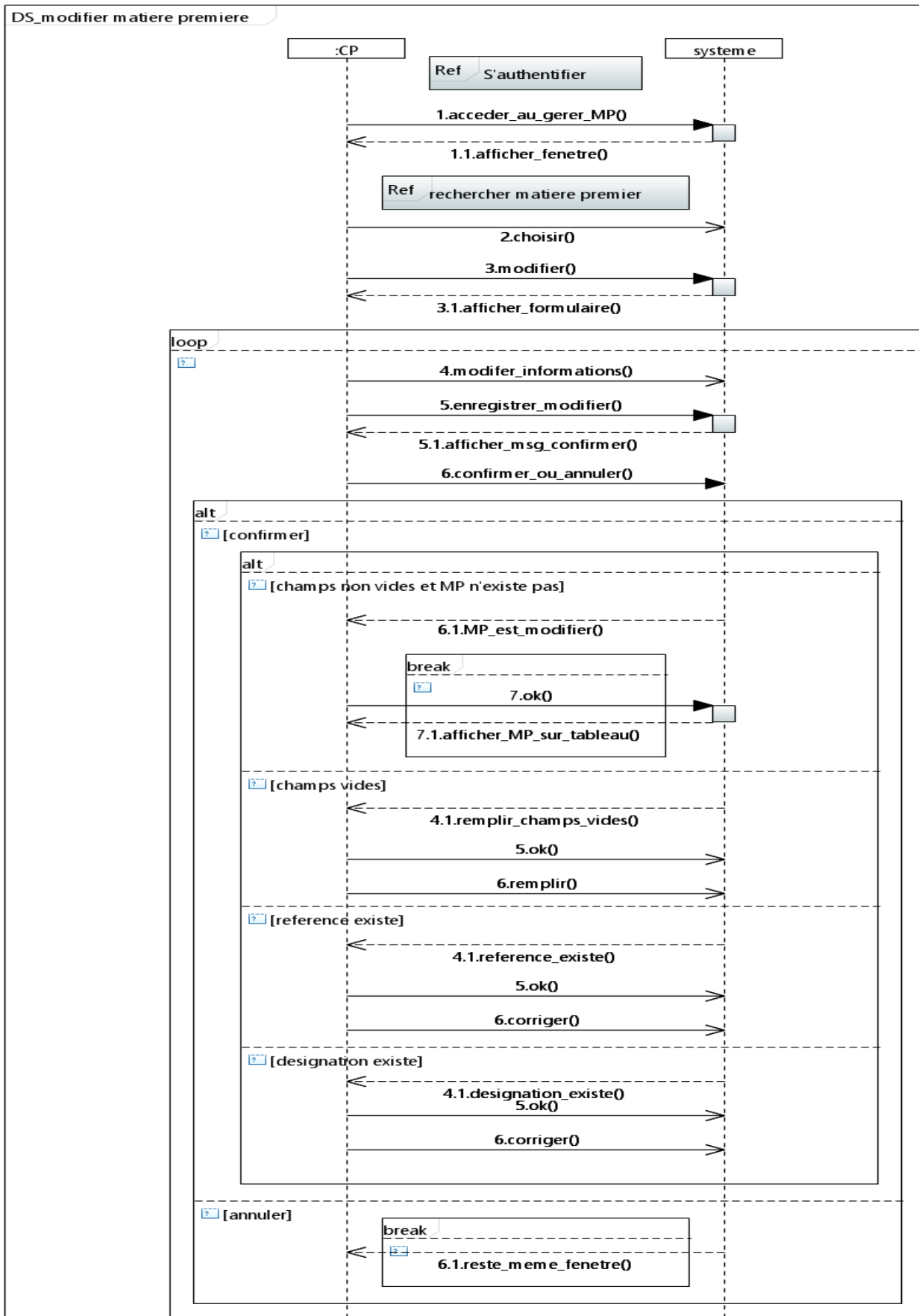
Figure 56 – Diagramme de séquence de modifier matière premier scenario nominal et Alternatif.
