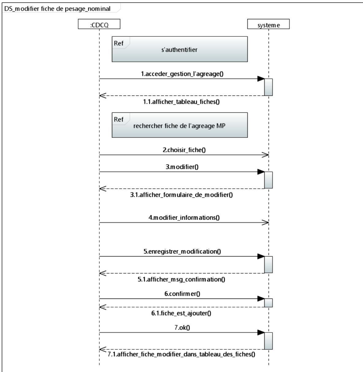
Figure 45 —Diagramme de séquence de modifier fiche de pesage nominal.
