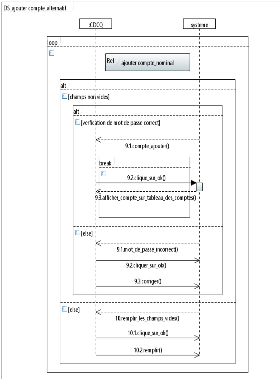
Figure 9 – Diagramme de séquence d'ajouter compte scenario alternatif.
