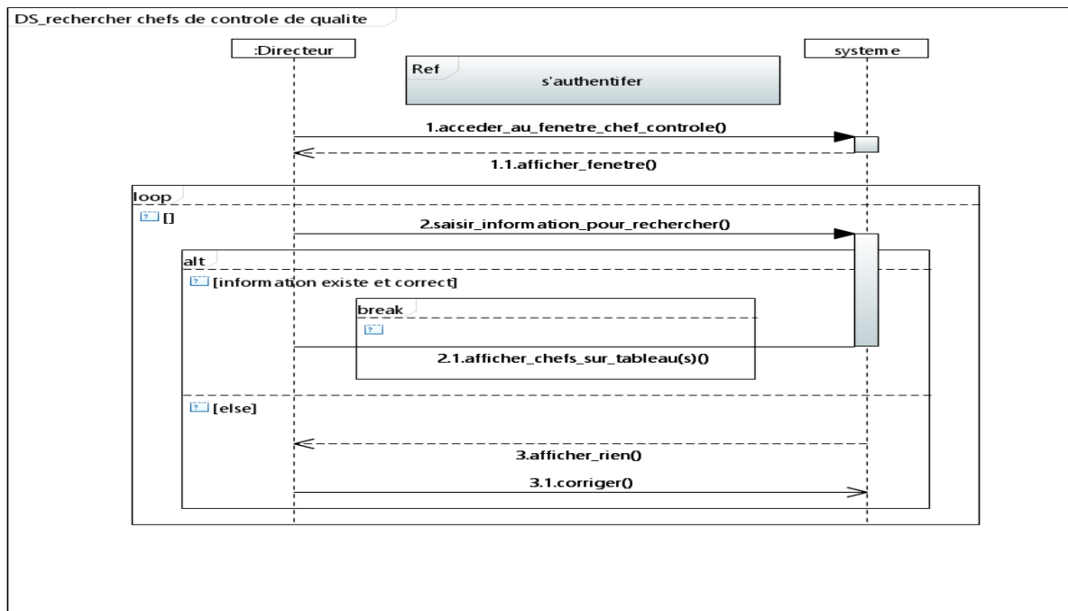
Figure 70 – Diagramme de séquence de chefs contrôle.
