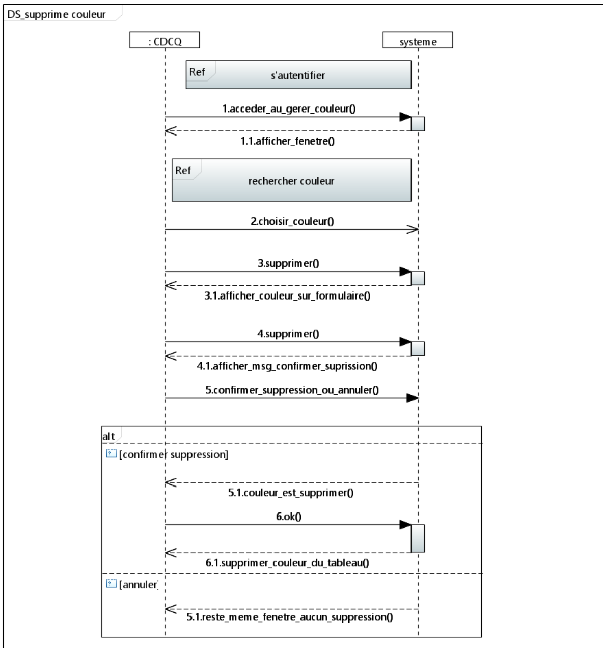
Figure 40 – Diagramme de séquence de supprimer couleur.
