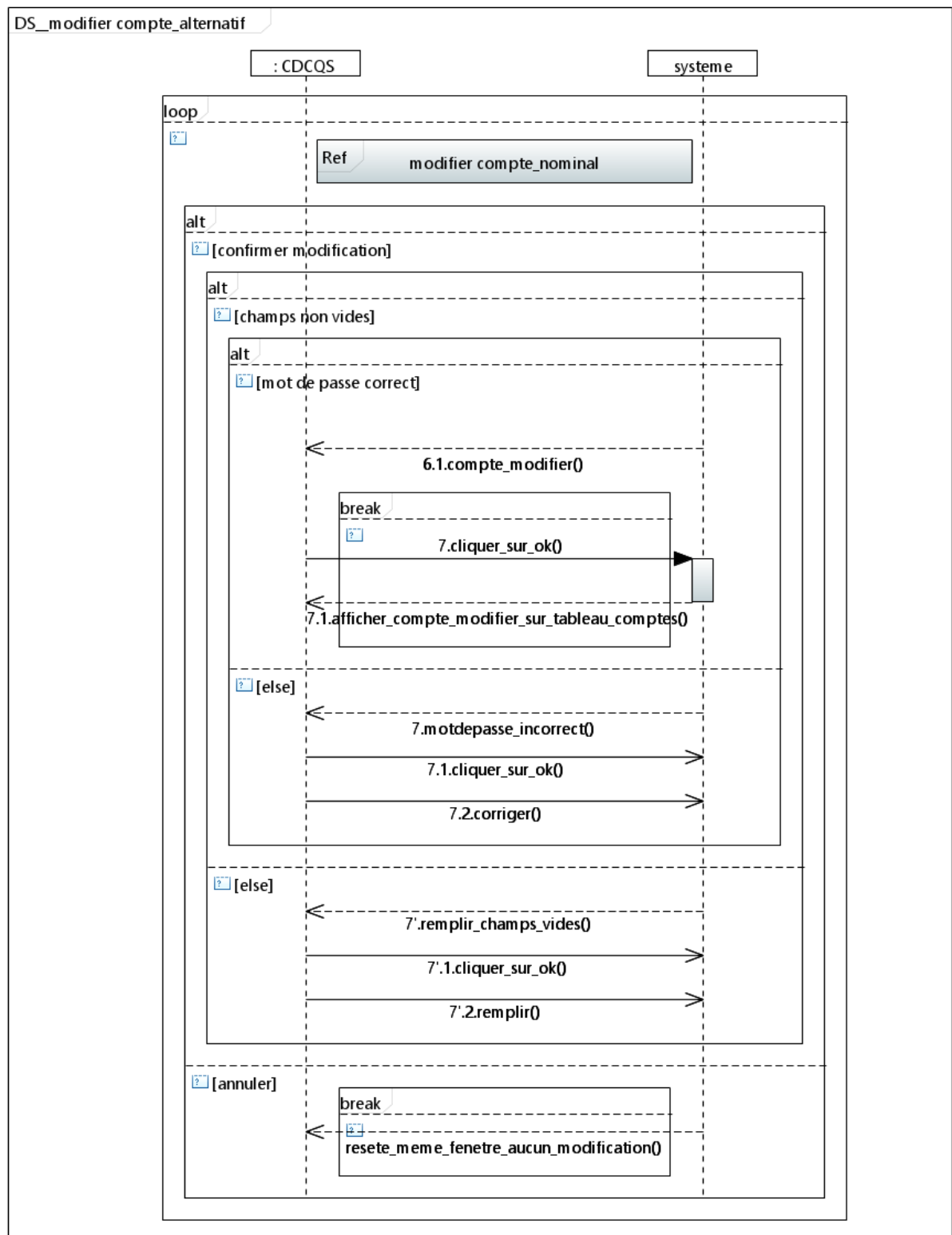
Figure 11 – Diagramme de séquence de modifier compte scenario alternatif.
