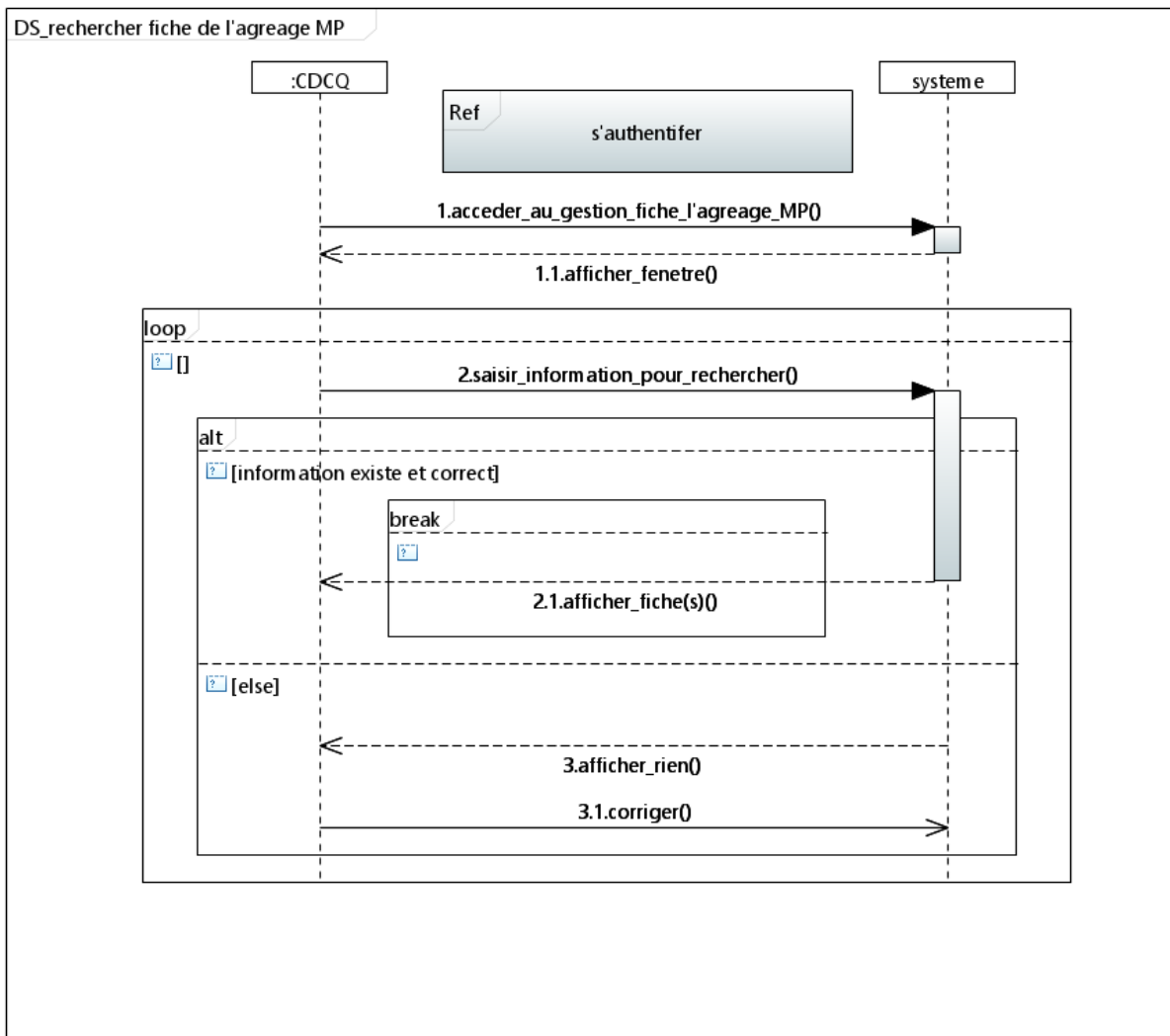
Figure 33 – Diagramme de séquence de recherche fiche de gestion L’agregage des matières premières scenario nominal et alternatif.
