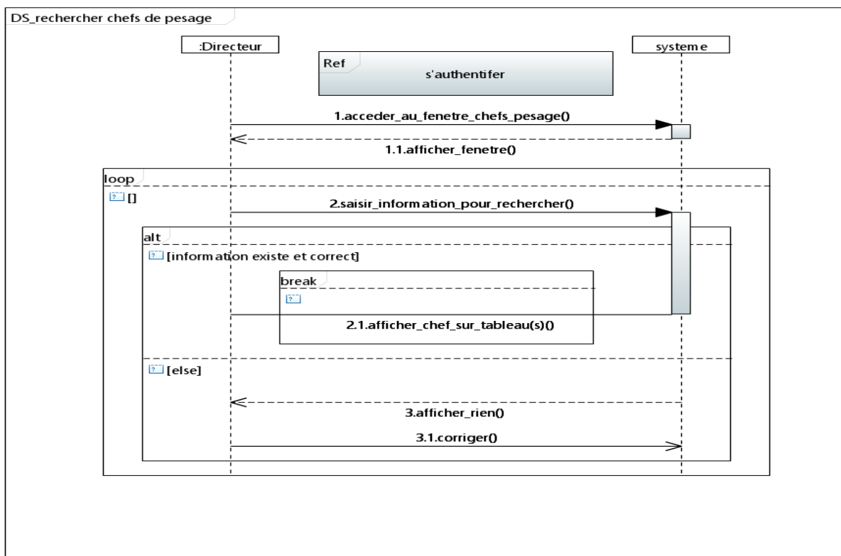
Figure 66 – Diagramme de séquence de chefs de pesage.
