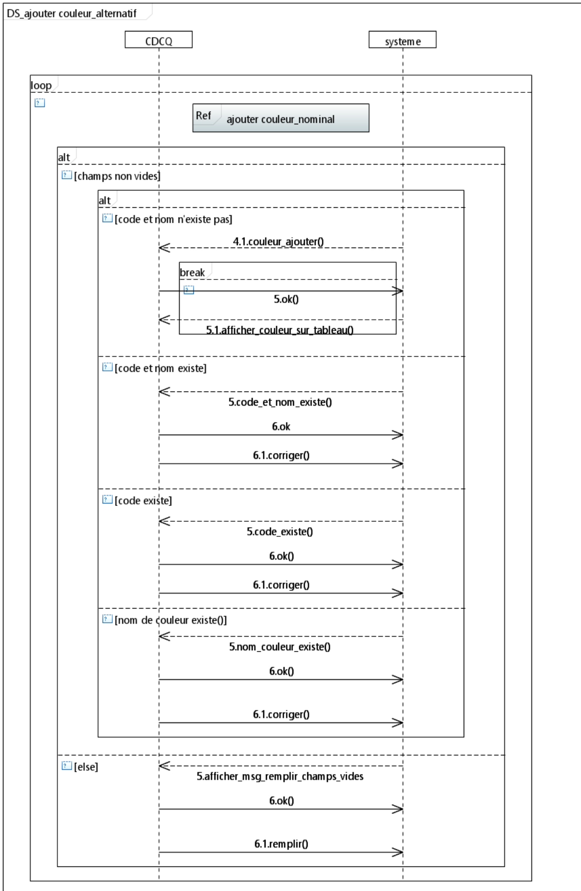
Figure 37 – Diagramme de séquence d'ajouter couleur Scenario Alternatif.
