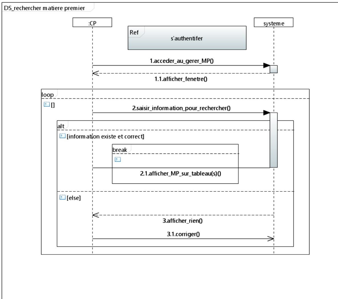
Figure 58 – Diagramme de séquence de rechercher matière première scenario nominal et alternatif.
