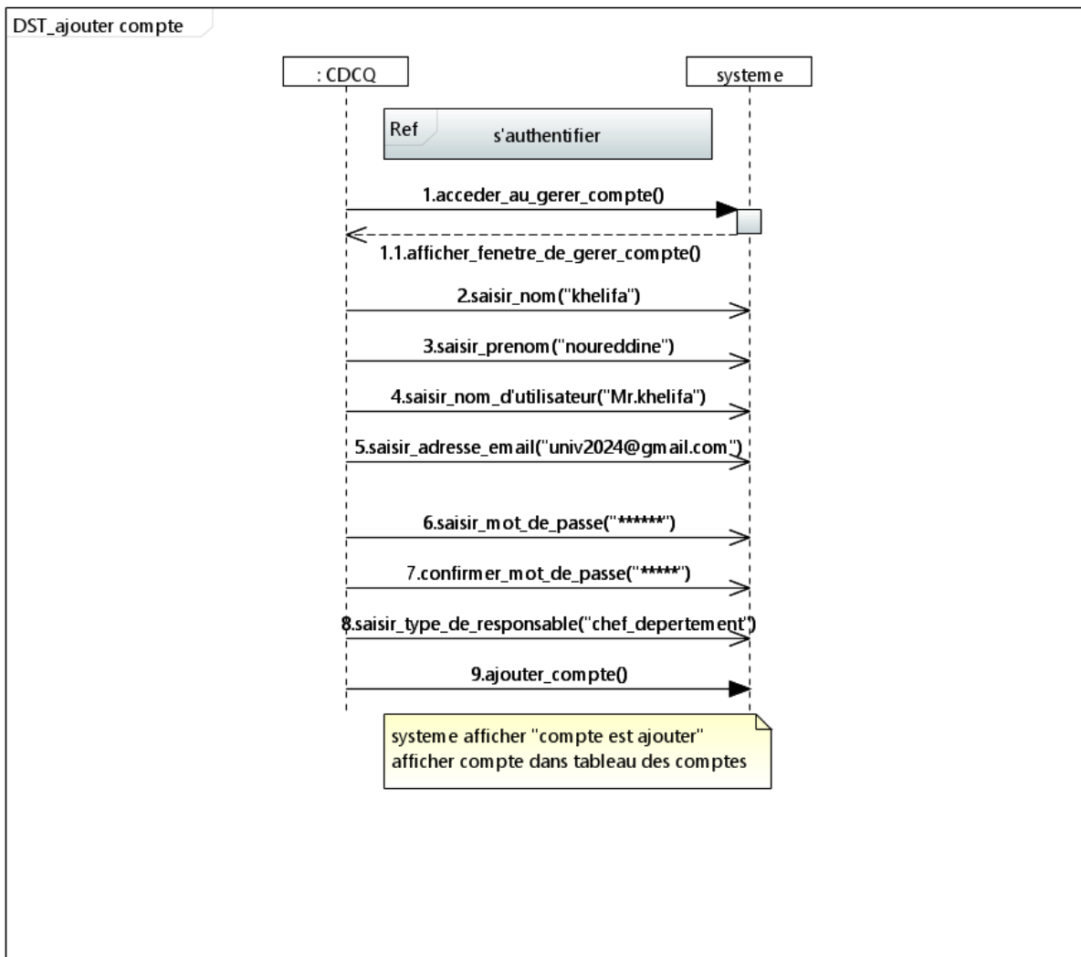
Figure 85 - Diagramme de teste de compte1.
