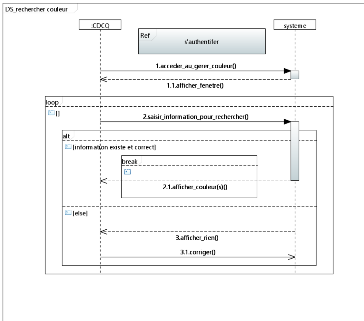
Figure 41 – Diagramme de séquence de rechercher couleur scenario nominal et alternatif.
