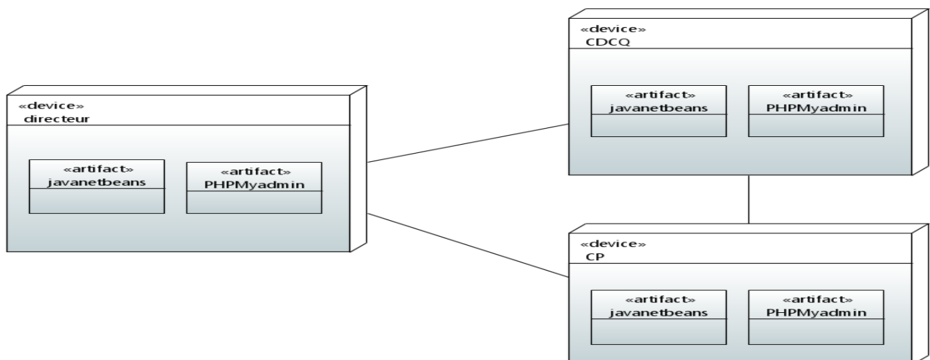
Figure 80 – Diagramme de déploiement.
