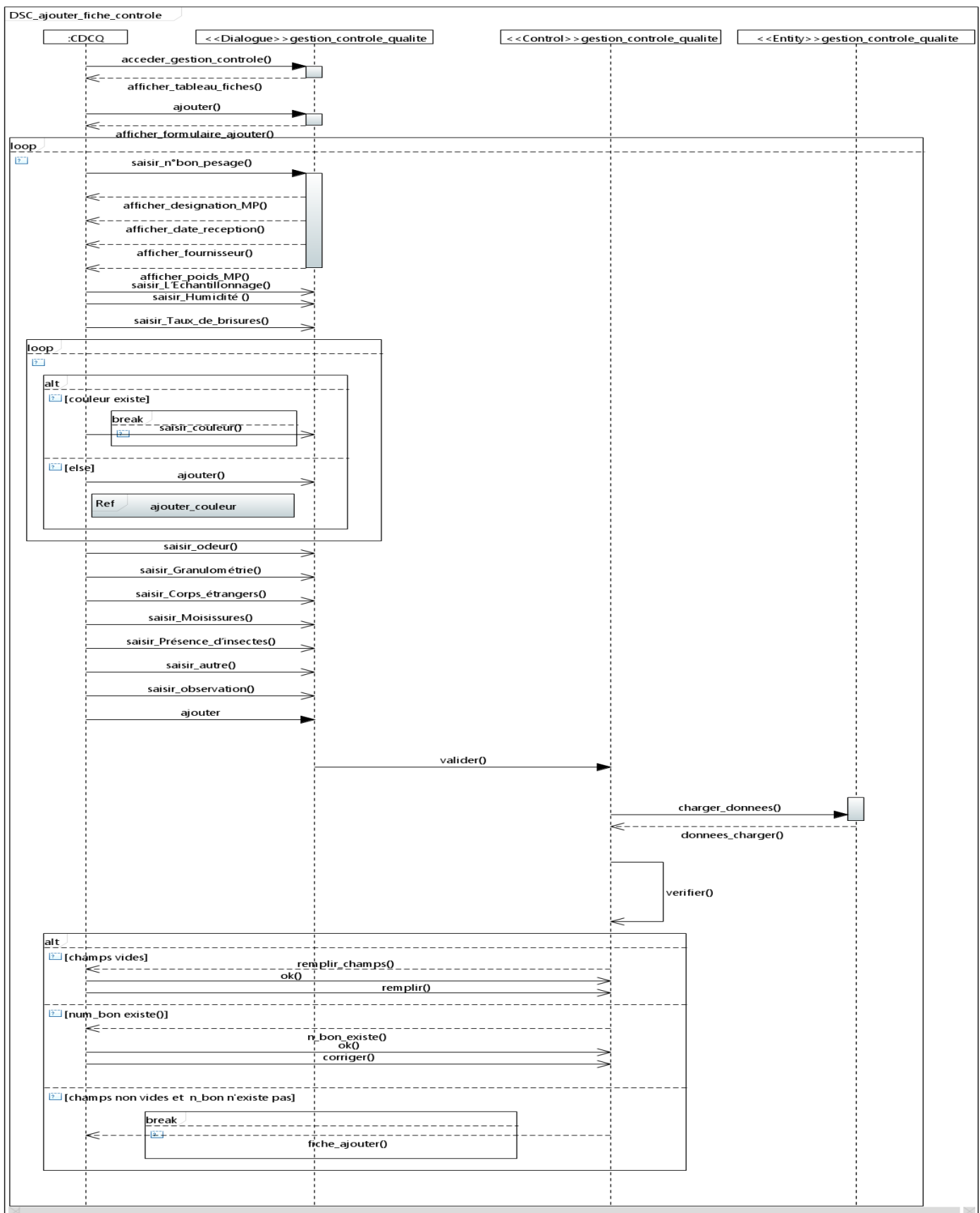
Figure77- Diagramme de séquence de conception d'ajouter fiche de contrôle.
