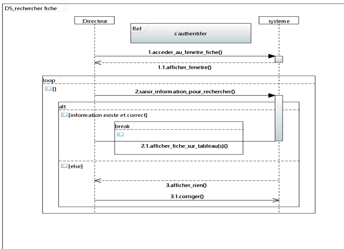
Figure 72 – Diagramme de rechercher fiches.
