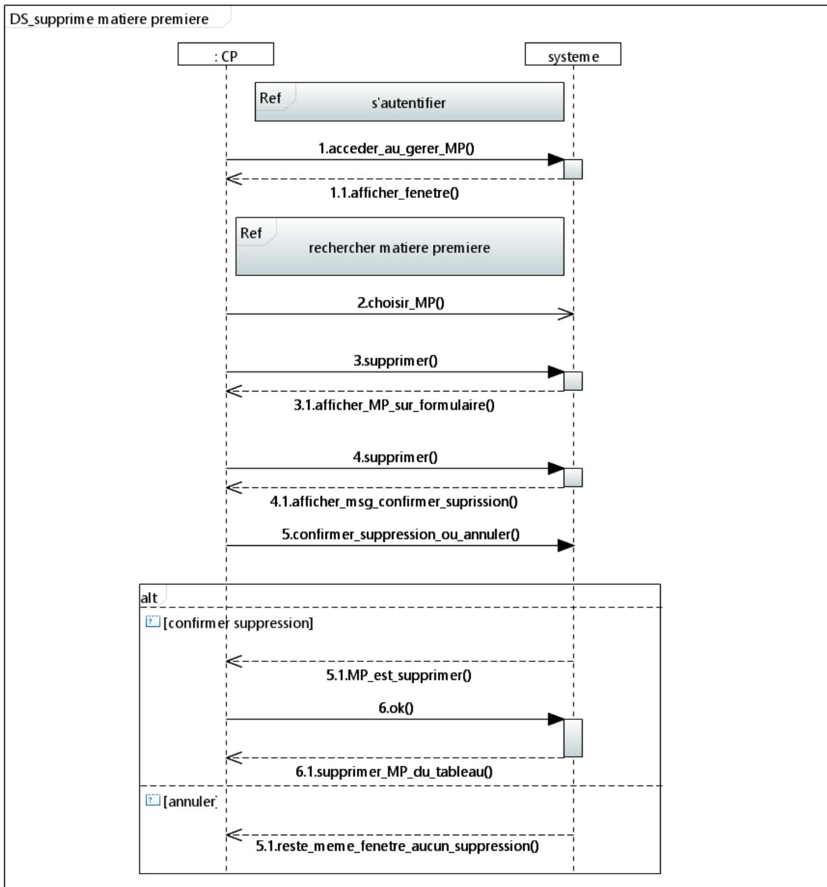
Figure 57 – Diagramme de séquence de supprimer matière première.
