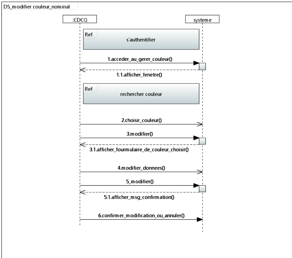
Figure 38 – Diagramme de séquence de modifier couleur scenario nominal.
