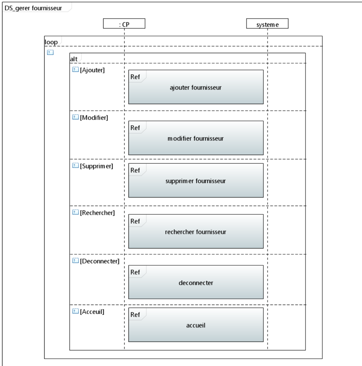
Figure 59 – Diagramme de séquence de gère fournisseur.
