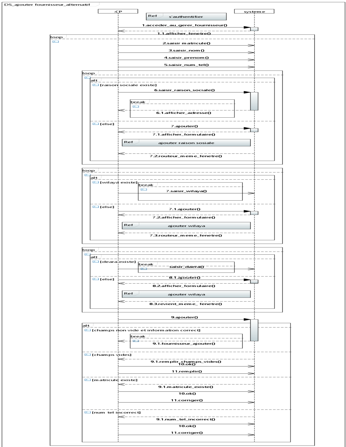
Figure 61– Diagramme de séquence d’ajouter fournisseur Scenario Alternatif.
