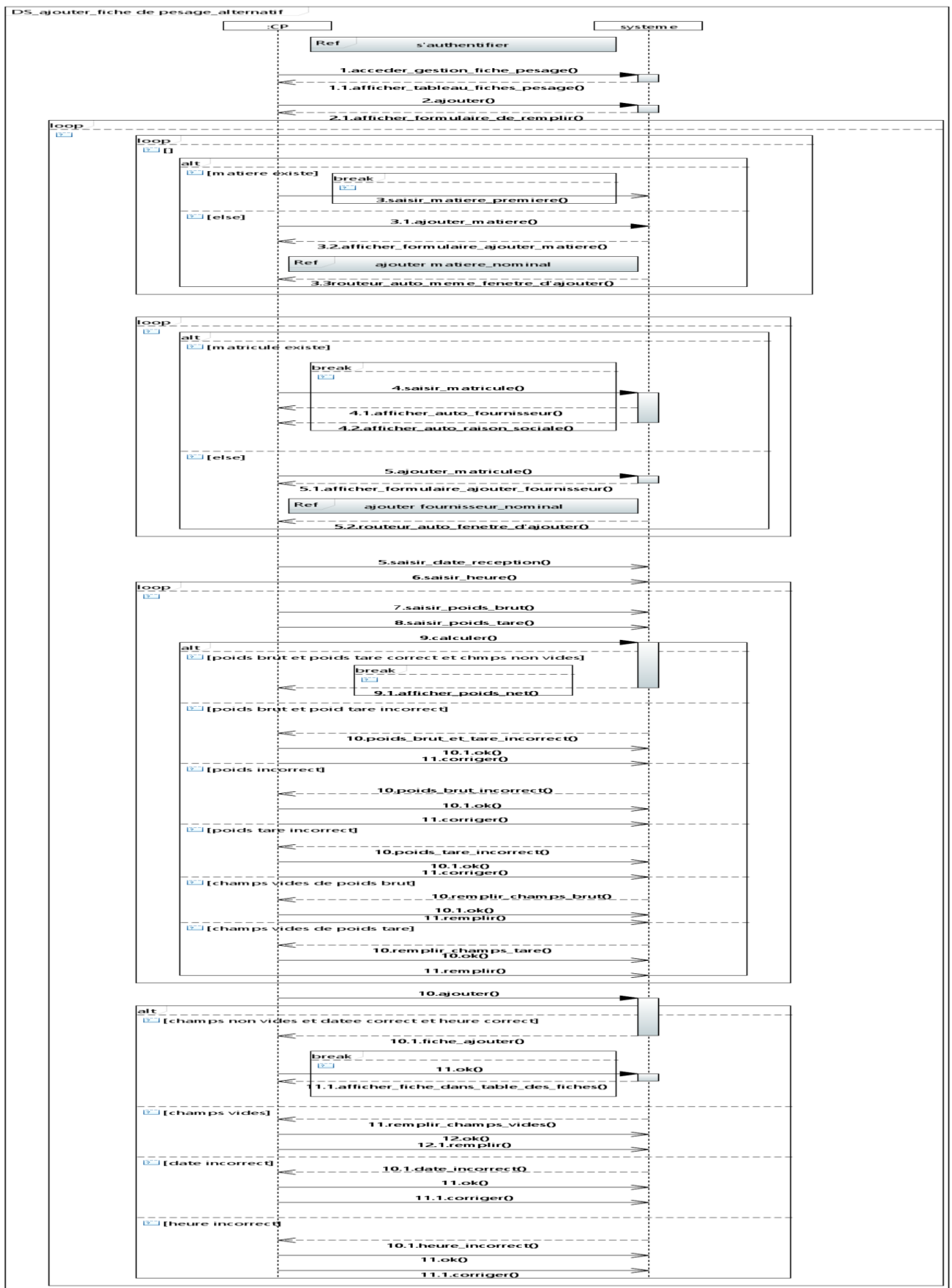
Figure 44–Diagramme de séquence d'ajouter fiche de pesage nominal+ alternatif.
