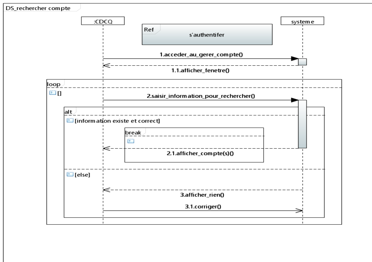
Figure 13 – Diagramme de séquence de rechercher compte scenario Nominal et alternatif.
