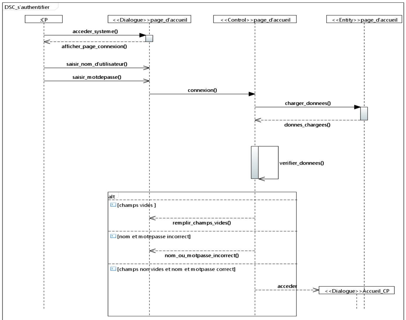
Figure76 - Diagramme de séquence de conception de s'authentifier.
