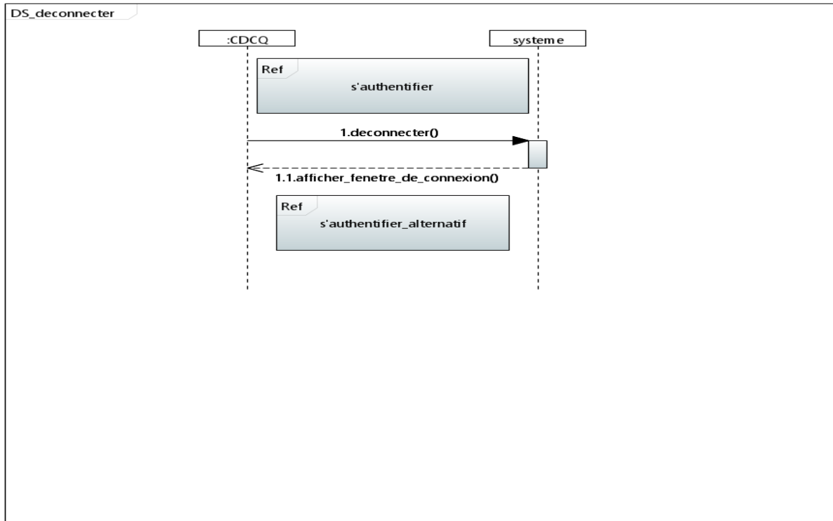
Figure 15 – Diagramme de séquence de déconnecter.
