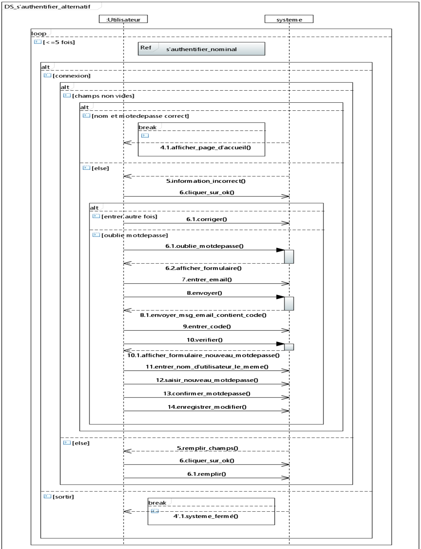
Figure 18– Diagramme de séquence d'Authentification Scenario Alternatif.
