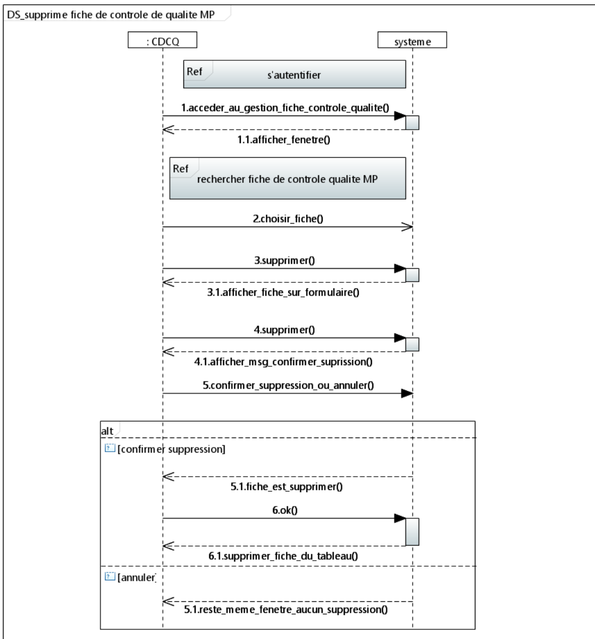
Figure 24 – Diagramme de séquence de supprimer la fiche de contrôle des matières premières a la réception.
