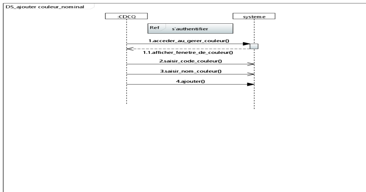
Figure 36 – Diagramme de séquence d'ajouter couleur scenario nominal.
