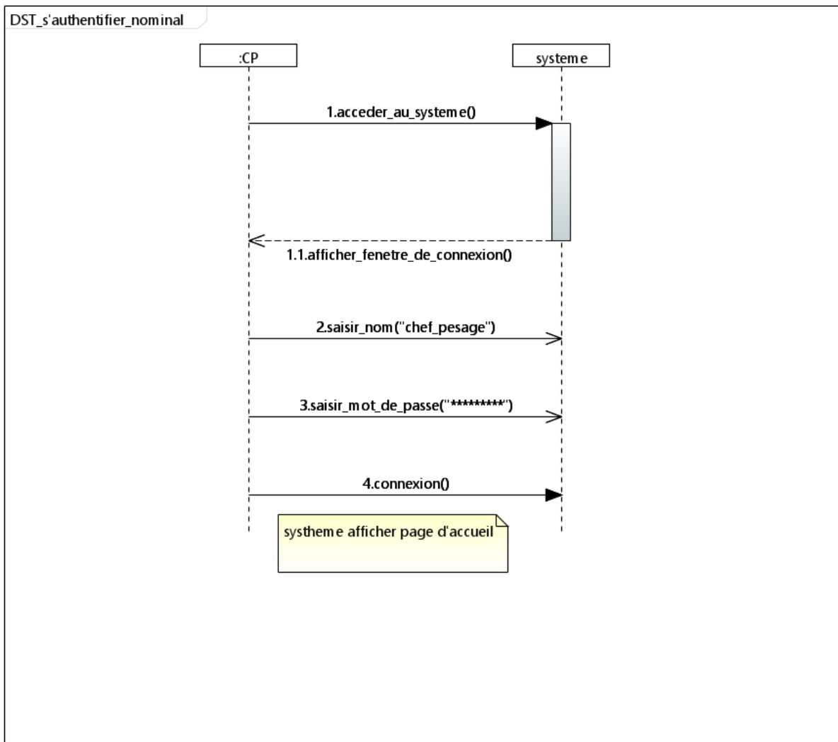
Figure 82 - Diagramme de teste de d'authentification2.
