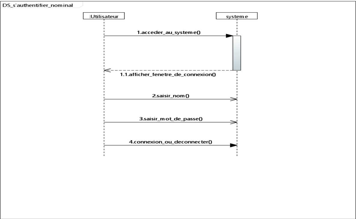
Figure 17 – Diagramme de séquence d'Authentification Scenario nominal.
