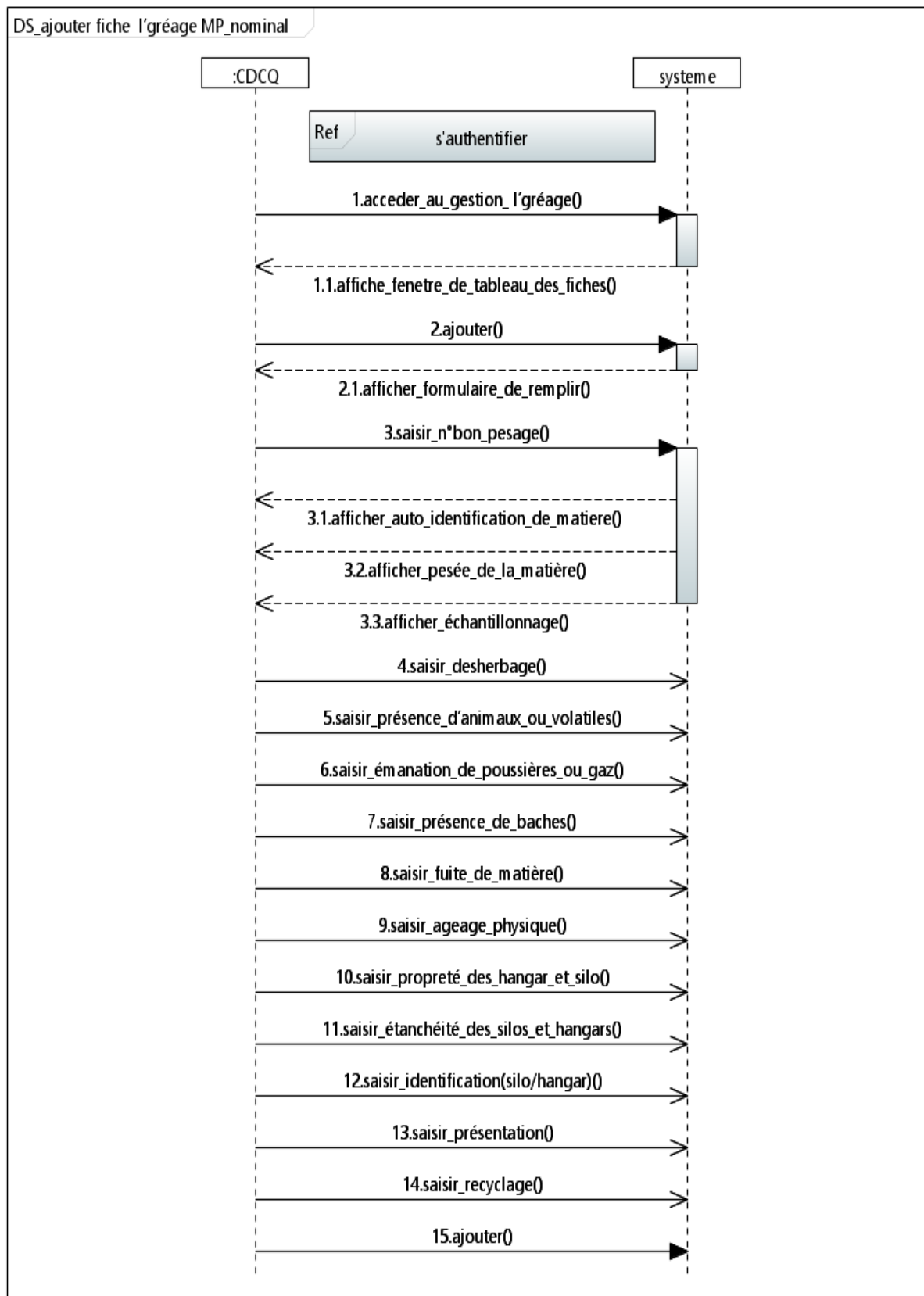
Figure 29 – Diagramme de séquence d'ajouter fiche de gestion L'ageage des matières premières scenario nominal.
