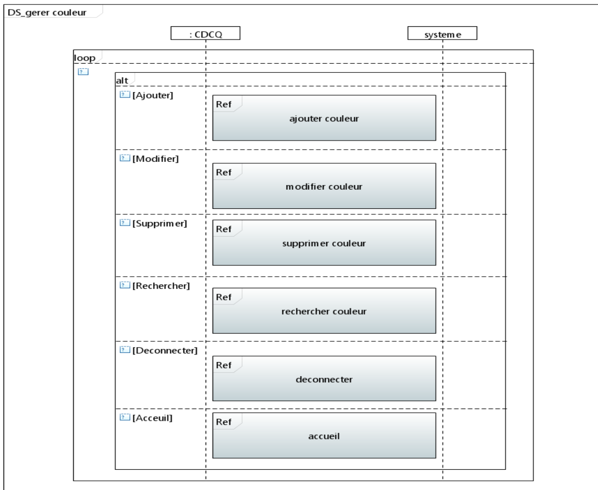
Figure 35 – Diagramme de séquence de gérer couleur.
