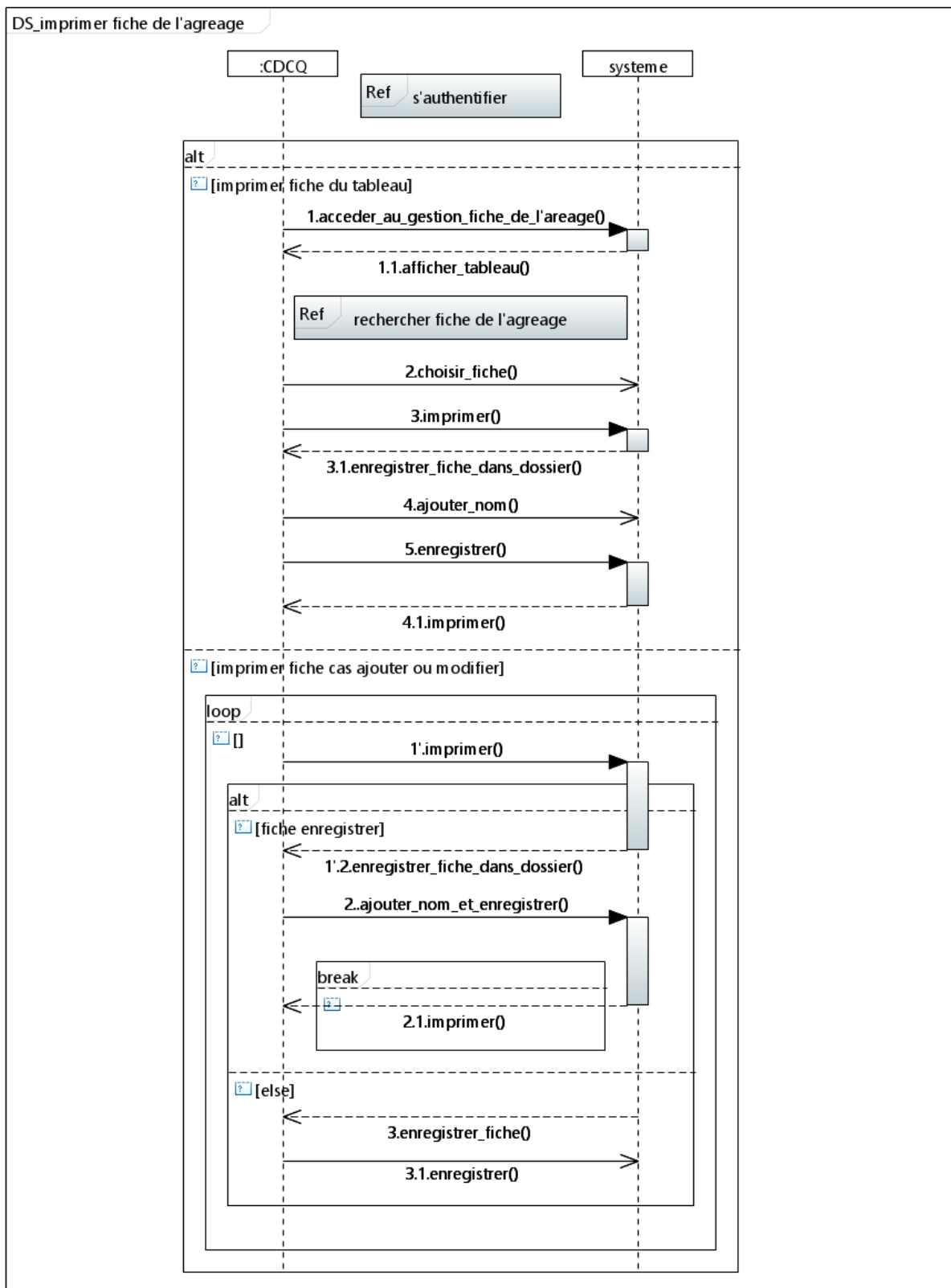
Figure 34 – Diagramme de séquence d'imprimer fiche de gestion L'agreage des matières premières scenario nominal et alternatif.
