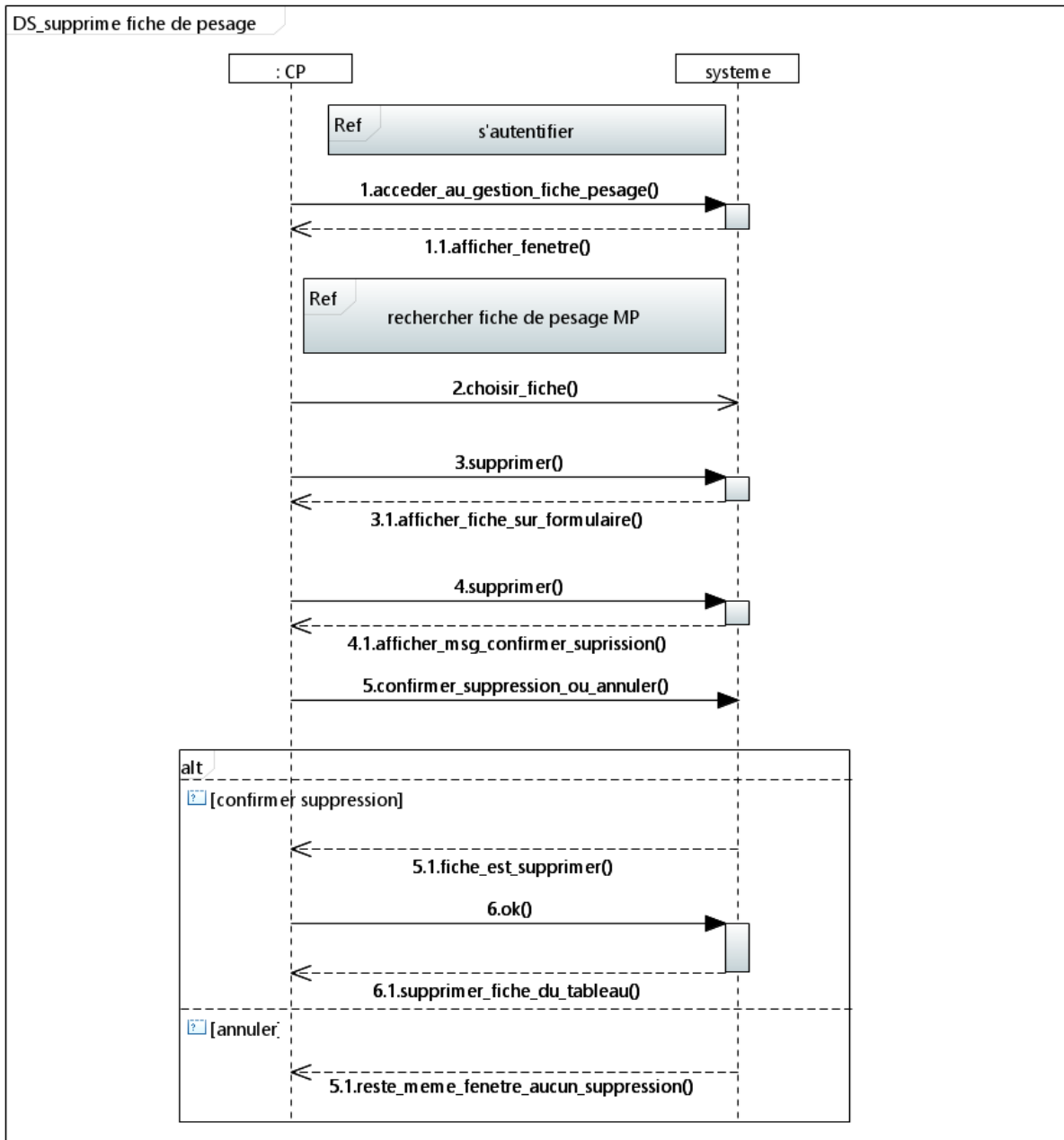
Figure 47 – Diagramme de séquence de supprimer fiche de pesage.
