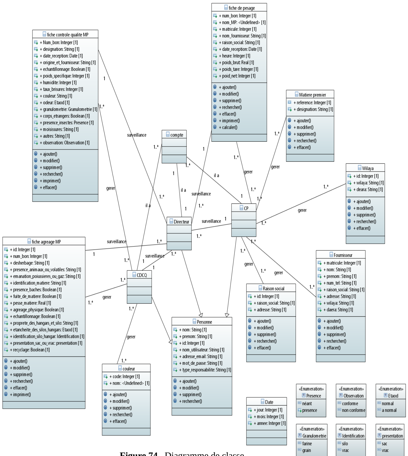
Figure 74– Diagramme de classe.
