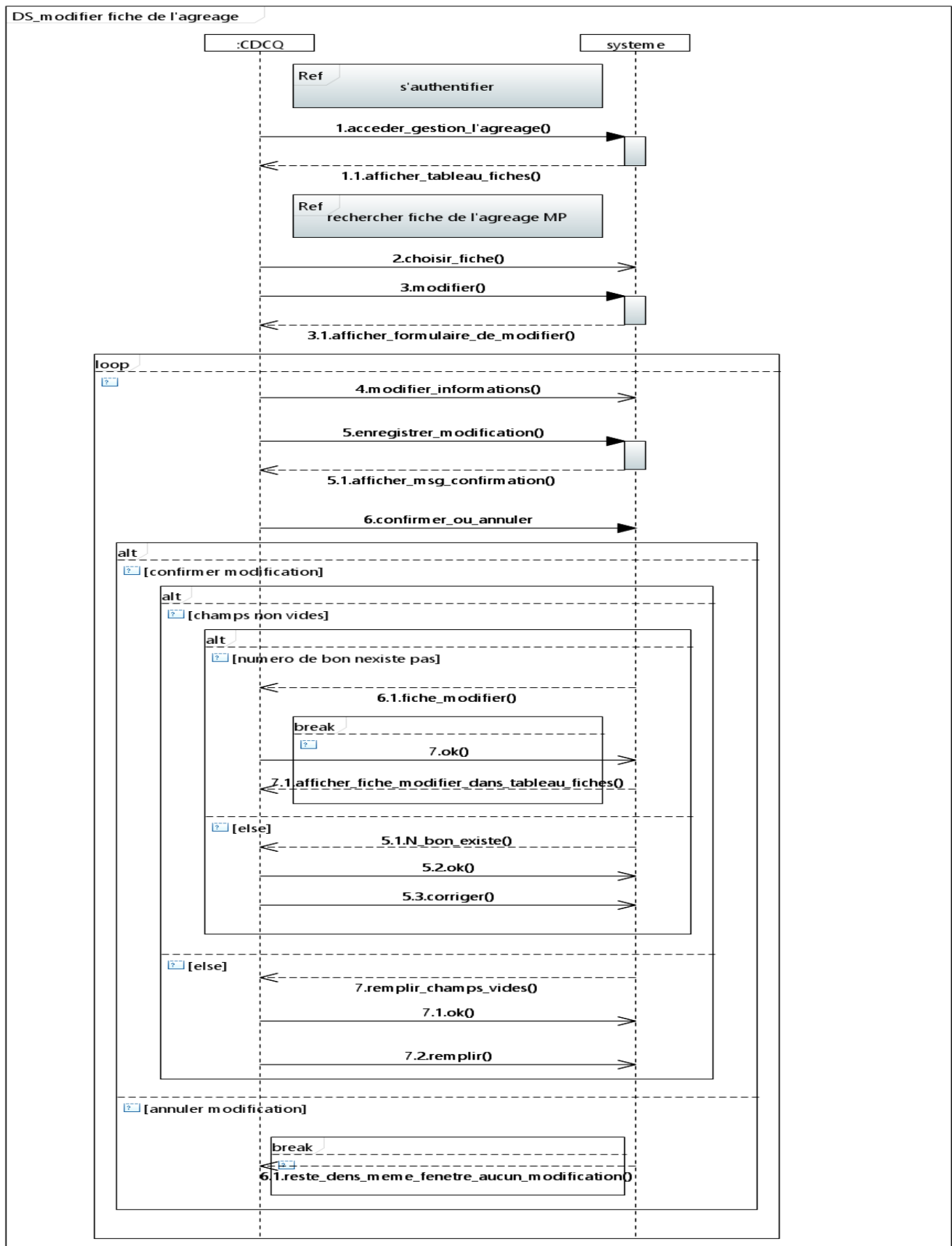
Figure 31 – Diagramme de séquence de modifier la fiche de gestion L'agregage des matières premières scenario nominal et alternatif.
