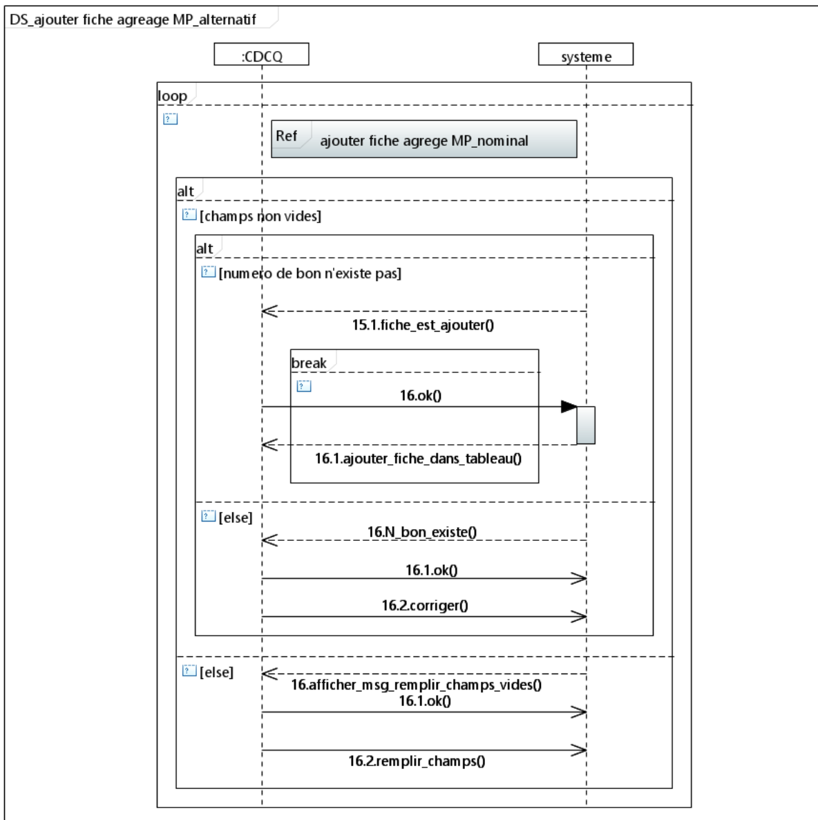
Figure 30 – Diagramme de séquence d’ajouter fiche de gestion L’agreage des matières premières scenario alternatif.
