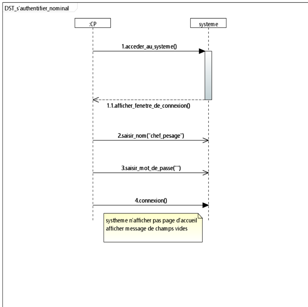
Figure 81 - Diagramme de teste de d'authentification1.
