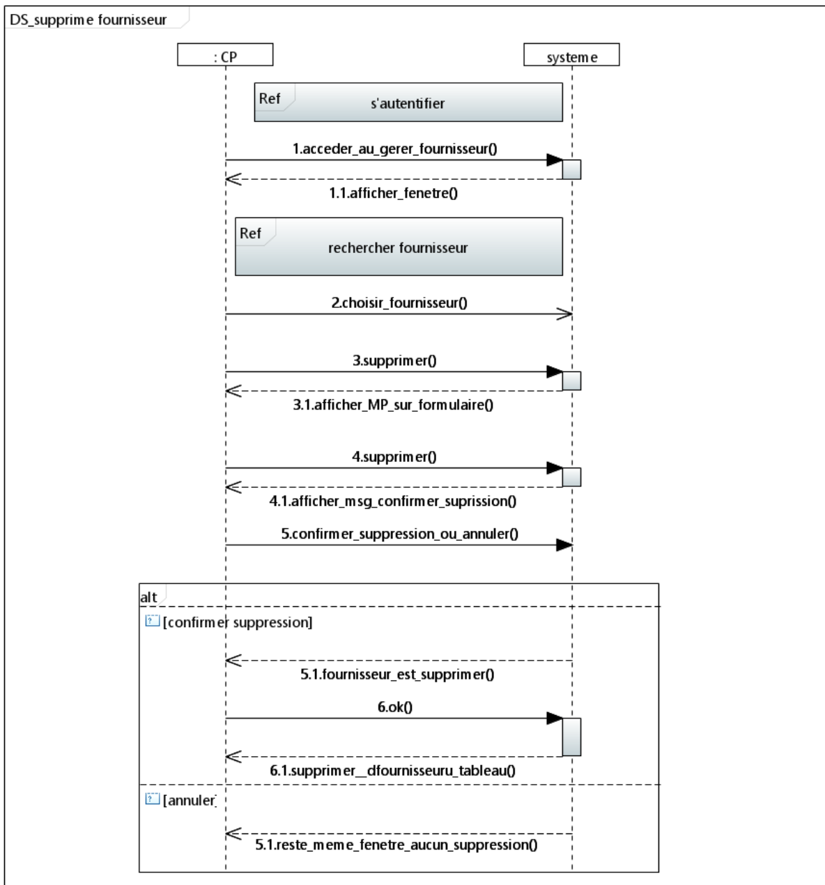
Figure 62 – Diagramme de séquence supprimer fournisseur.
