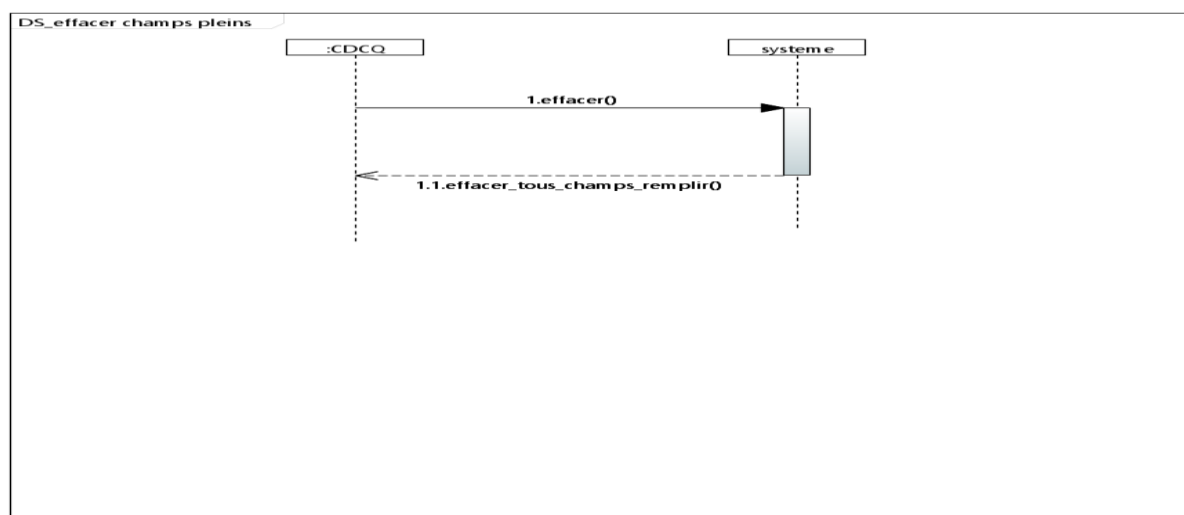
Figure 14 – Diagramme de séquence d’effacer les champs de compte.
