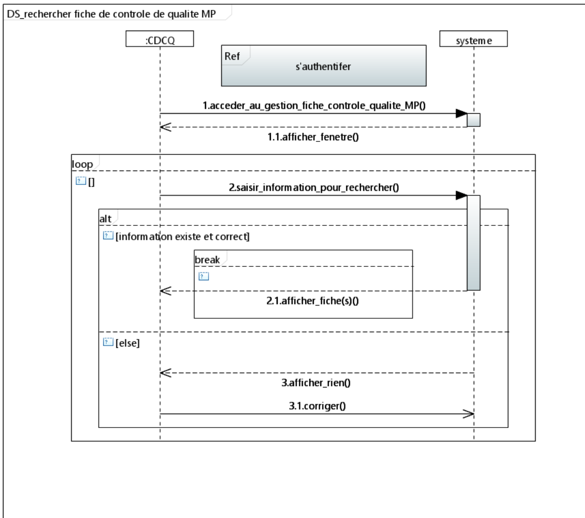
Figure 25 – Diagramme de séquence de rechercher fiche de contrôle des matières premières a la réception Scenario Nominal et alternatif.
