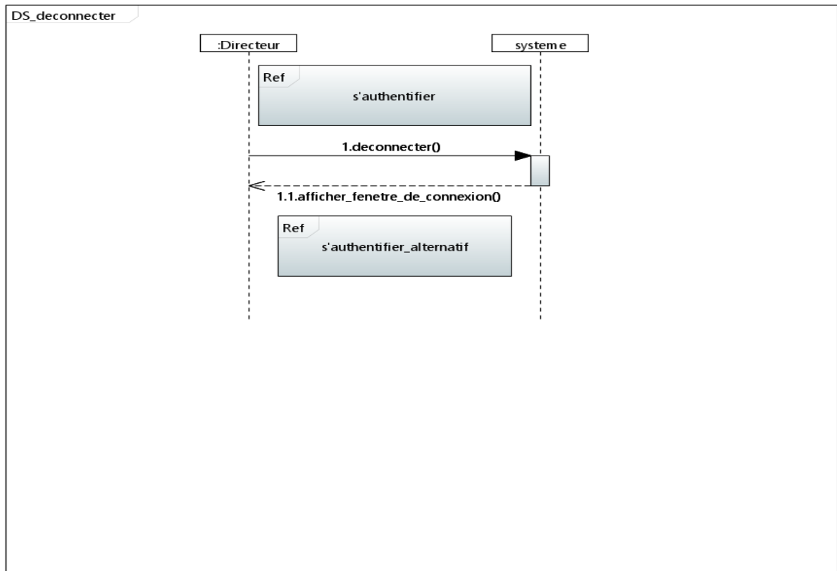
Figure 68 – Diagramme de séquence de déconnecter.
