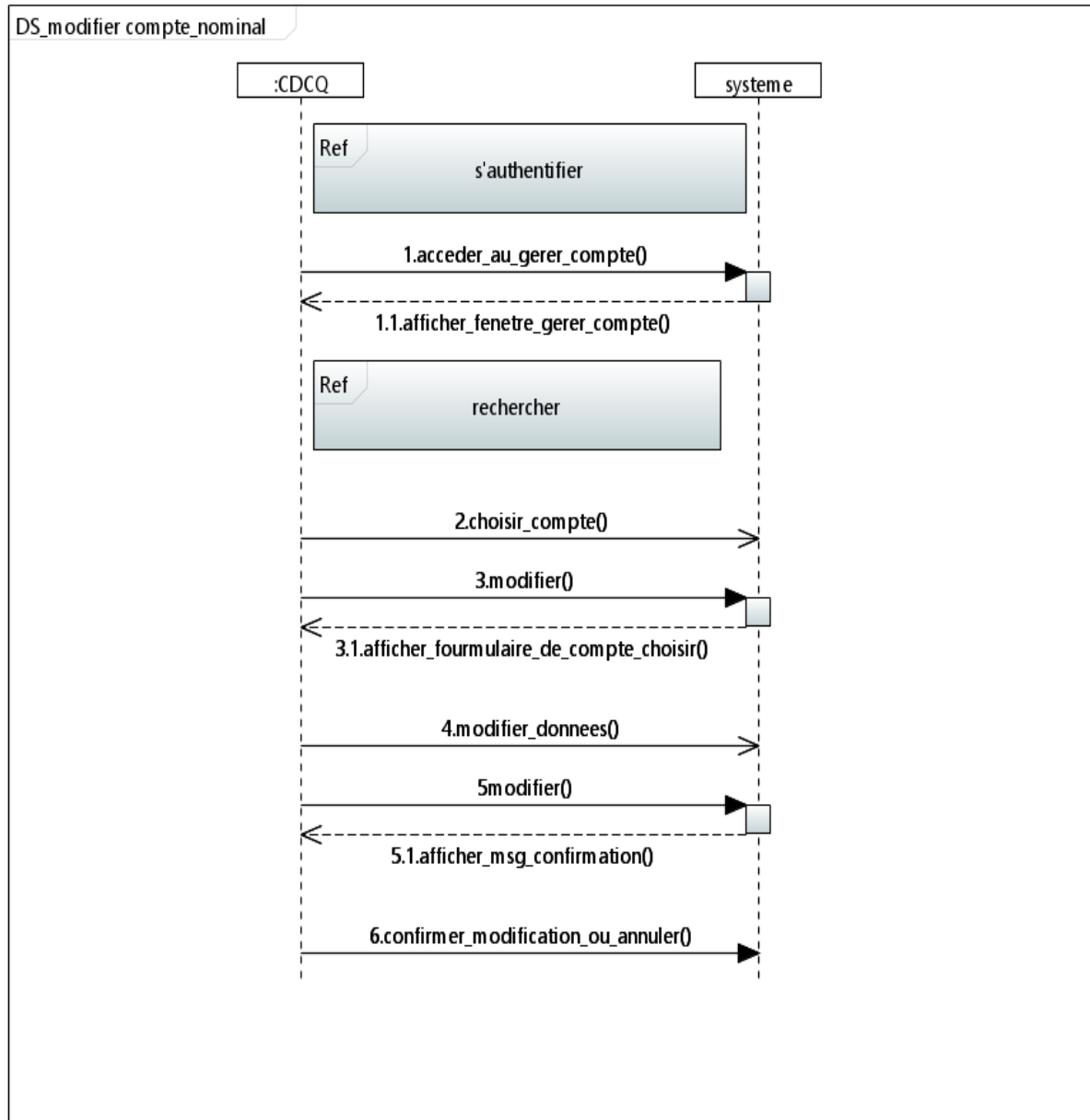
Figure 10 – Diagramme de séquence de modifier compte scenario Nominal.
