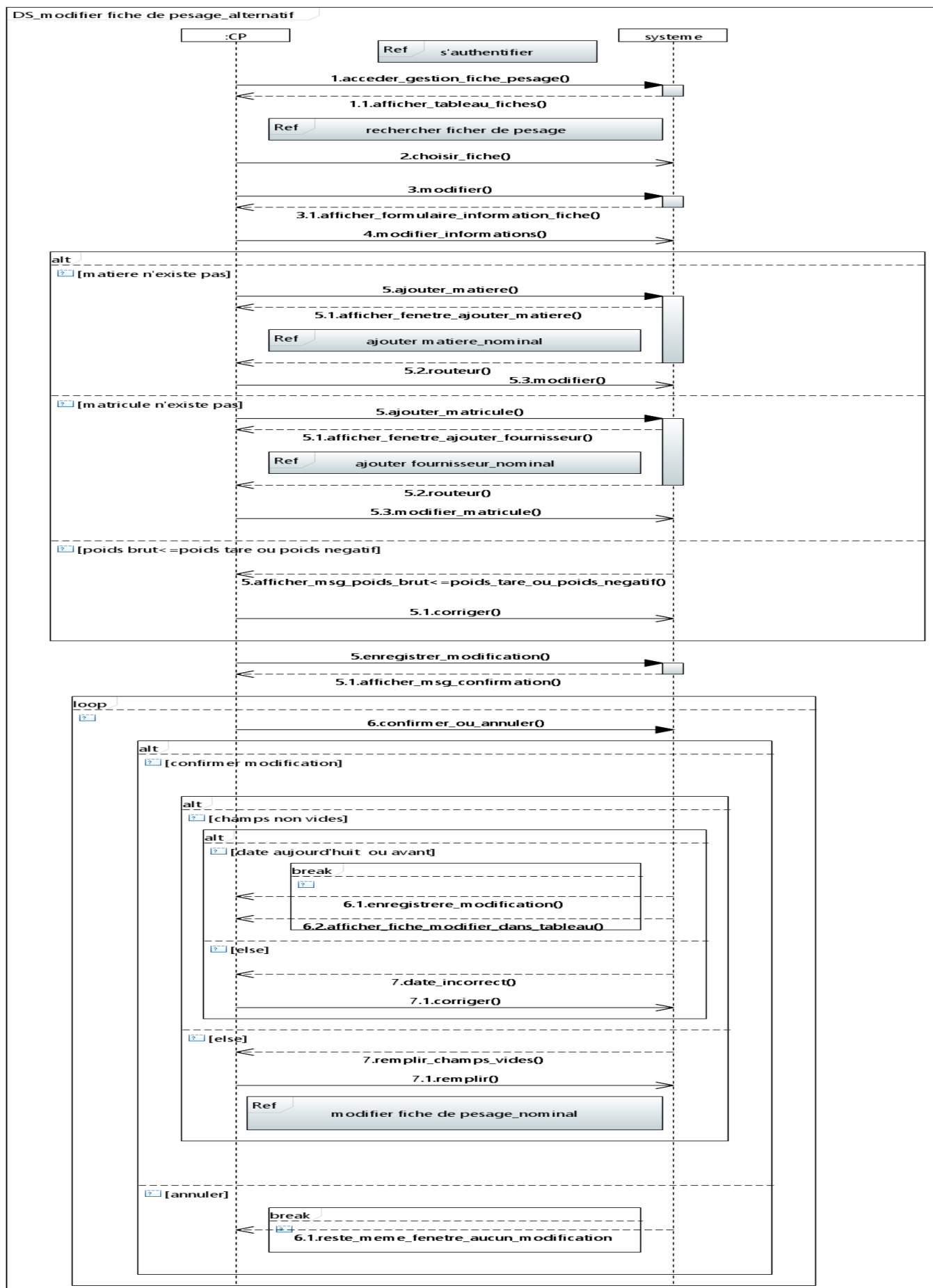
Figure 46–Diagramme de séquence de modifier fiche de pesage alternatif.
