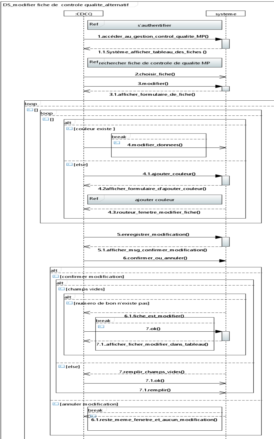
Figure 23 – Diagramme de séquence de modifier la fiche de contrôle des matières premières a la réception Scenario Alternatif.
