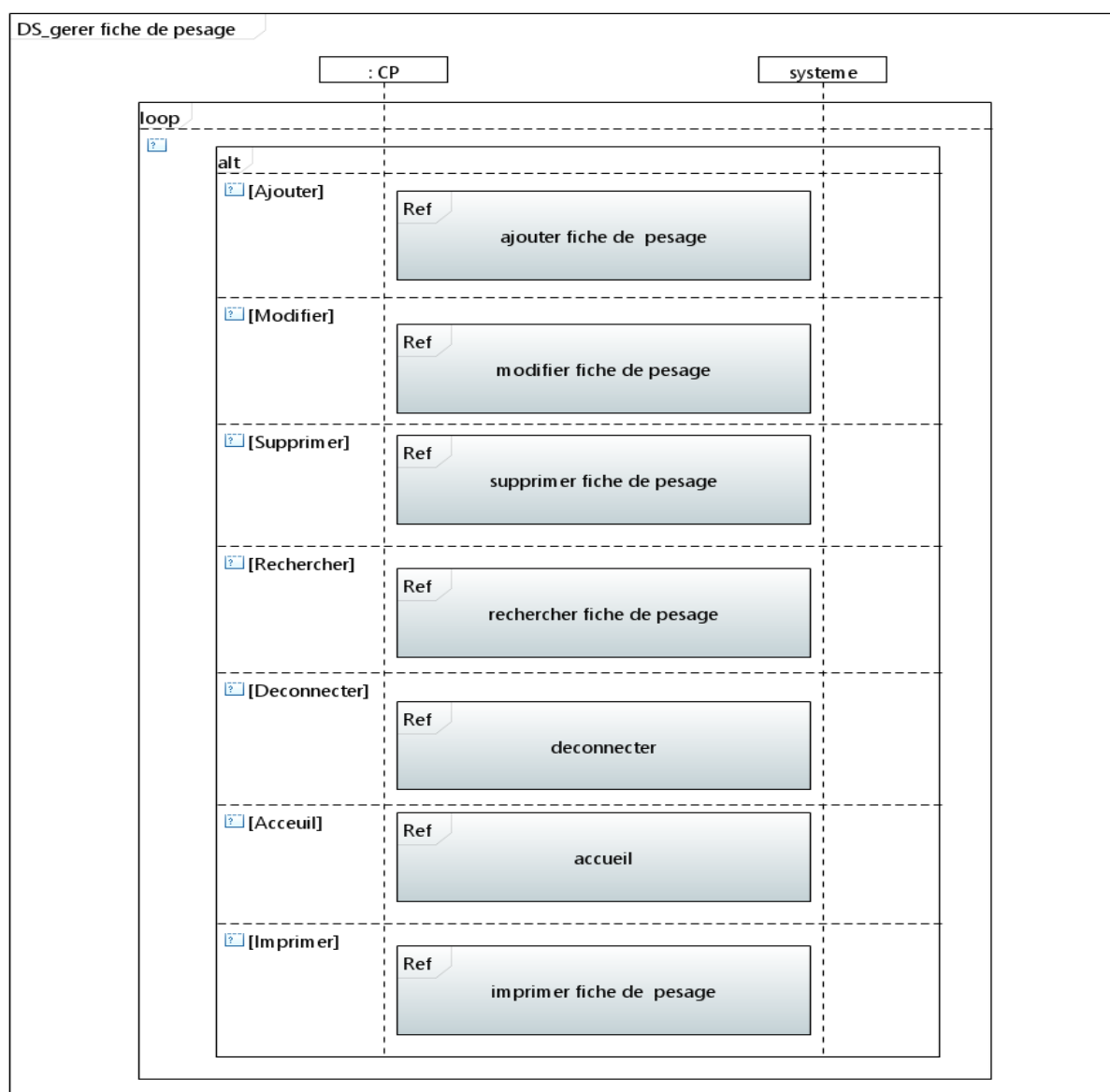
Figure 42–Diagramme de séquence de gestion des operation de pesage.
