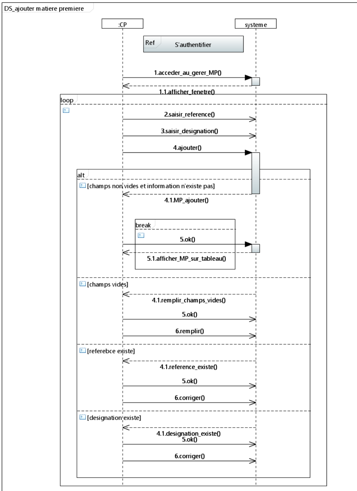
Figure 55 – Diagramme de séquence d'ajouter matière premier scenario nominal et Alternatif.
