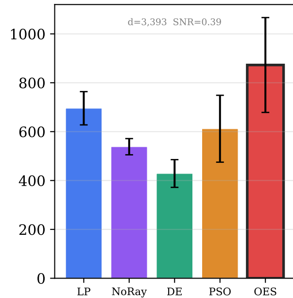
CartpoleSwingup
