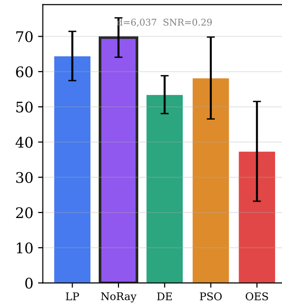
HumanoidWalk
