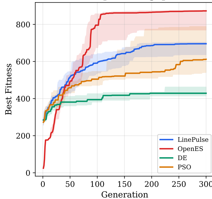
CartpoleSwingup
