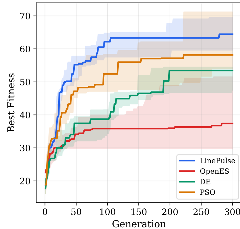
HumanoidWalk
