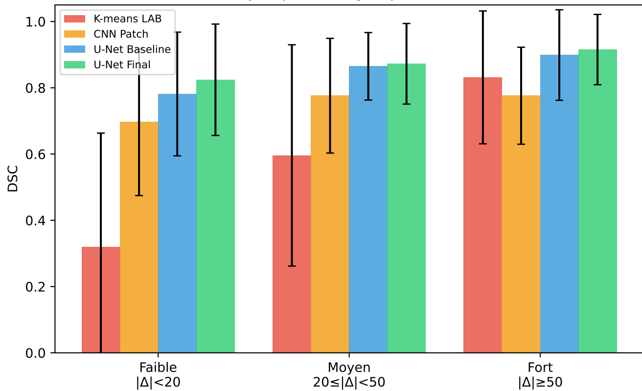
DSC moyen par sous-groupe de contraste
