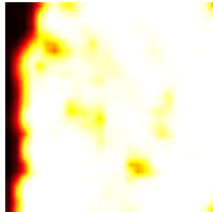
Prob. CNN
