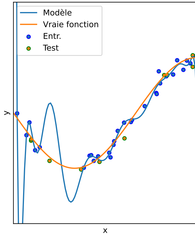
Degré 15 Erreur = 1.8\text{e+}08 (+/- 5.4\text{e+}08 )
