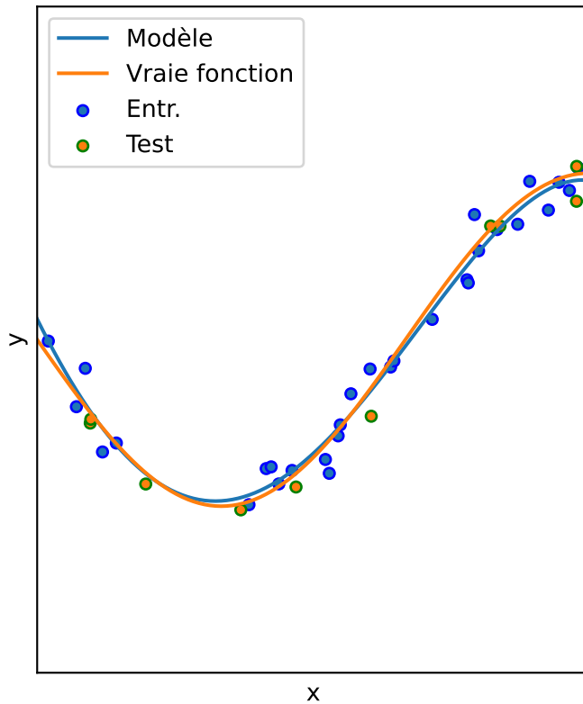
Degré 4 Erreur = 2.3\text{e-}02 (+/- 1.9\text{e-}02 )
