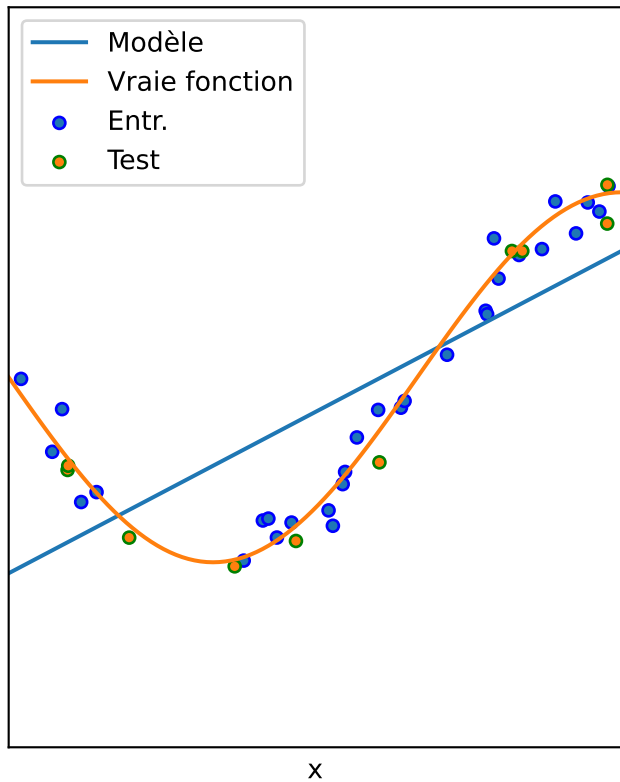
Degré 1 Erreur = 3.6\text{e-}01 (+/- 5.4\text{e-}01 )
