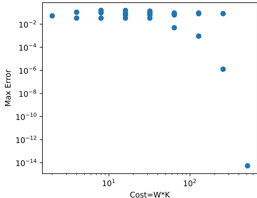
nu=1e-01 stable=25/25
