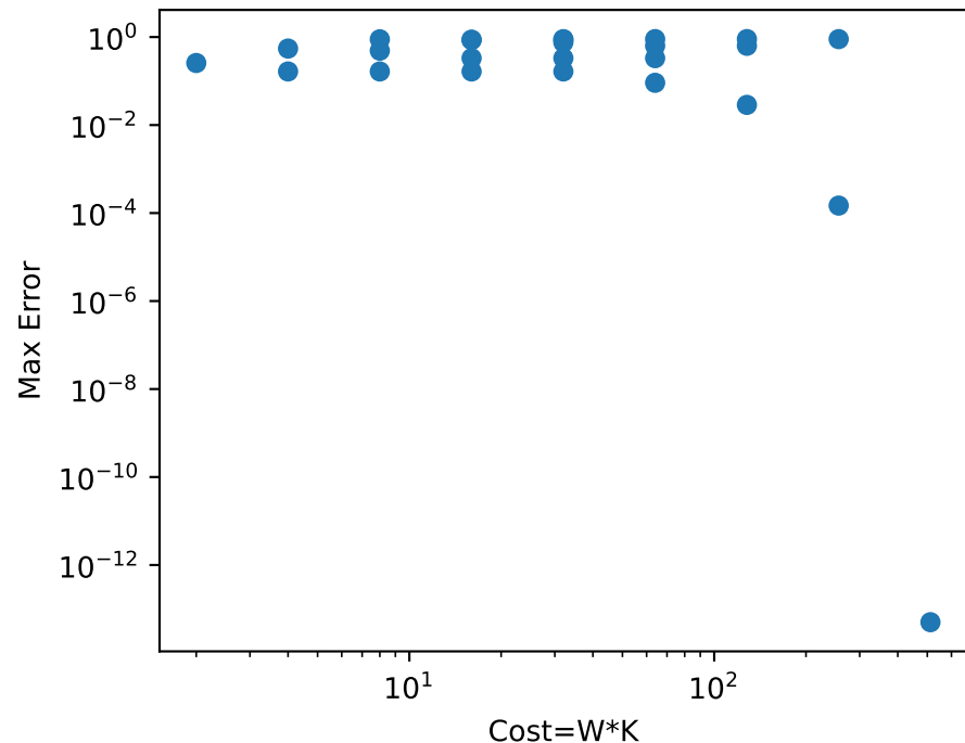
nu=1e-02 stable=25/25
