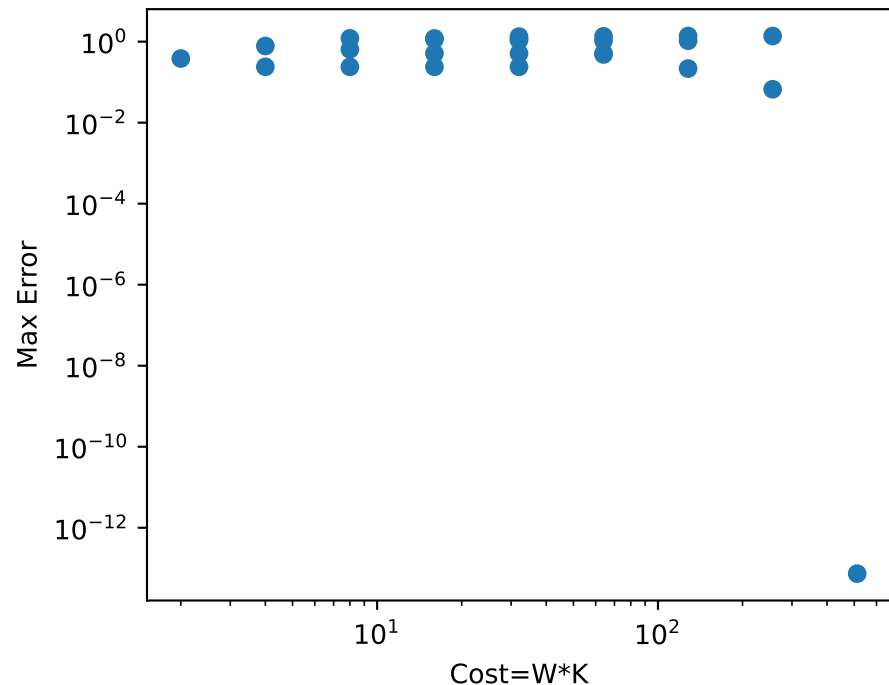
nu=1e-03 stable=25/25
