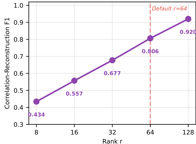
(d) LowRankGNN Rank Sensitivity ( d=500 )
