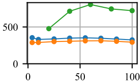
Ycsb
