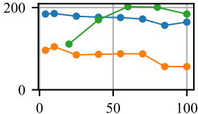
Utxo
