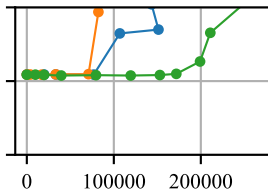
Wan - Utxo
