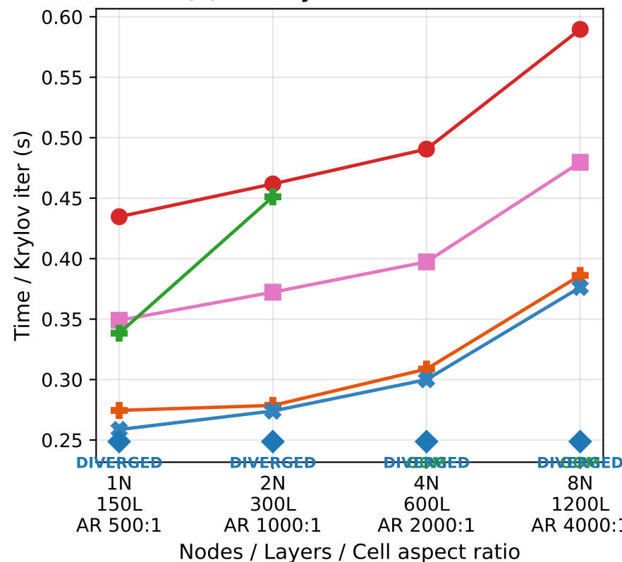
(d) Per-Krylov-iteration cost
