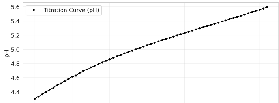
Titration Curve
