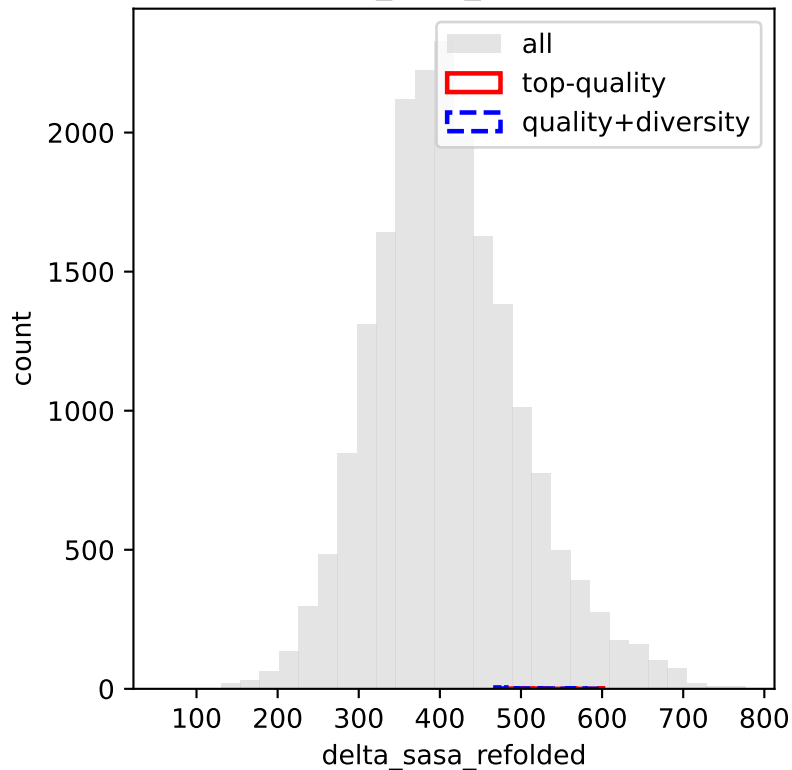
delta_sasa_refolded
