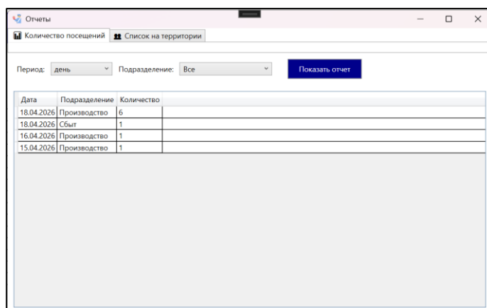
Рисунок 23 – Составление отчетов
