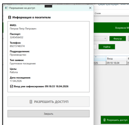
Рисунок 30 – Разрешение доступа
