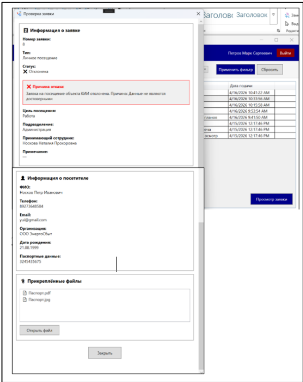
Рисунок 22 – Просмотр заявки
