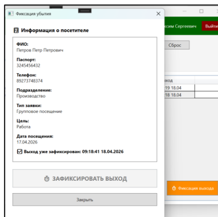
Рисунок 31 – Фиксация выхода
