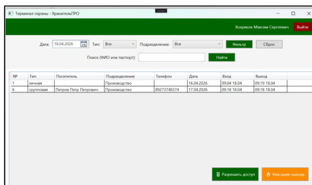
Рисунок 29 – Главное окно
