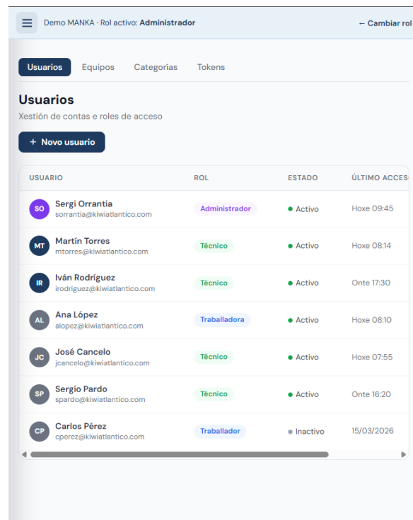
8. Xestión dos usuarios do administrado
