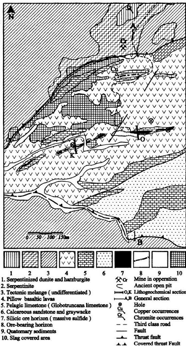
شکل ۳ - نقشه زمین‌شناسی کانسار؛ افق کانه‌دار سیلیسی (ماسیو
