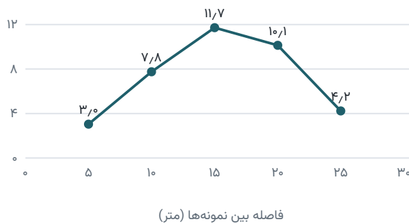
شکل ۱۳ - نیم‌تغییرنمای عیار مس (گام ۵ متر)
