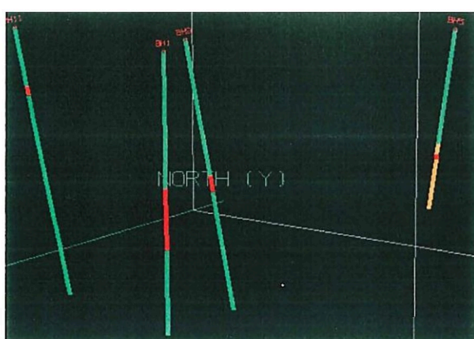
شکل ۴ - موقعیت فضایی گمانه ها (بخش قرمز: ماده معدنی). راست: همه گمانه ها؛ چپ: گمانه های برخوردکننده با ماده معدنی
