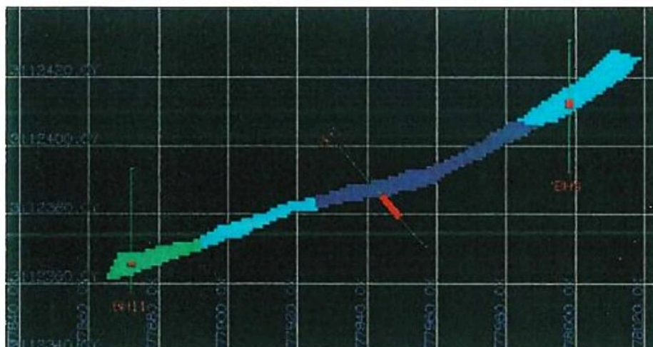
شکل ۷ - بلوک‌بندی کانسار و رنگ‌بندی بلوک‌ها بر اساس عیار مس (BH11 در چپ، BH9 در راست)
