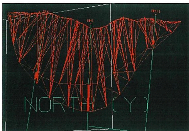
شکل ۶ - مدل سه‌بعدی هندسی کانسار؛ راست: Wireframe، چپ: مدل جامد
