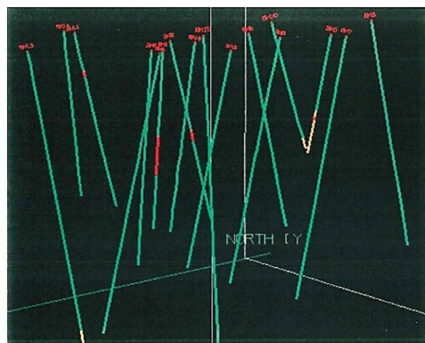
شکل ۴ - موقعیت فضایی گمانه ها (بخش قرمز: ماده معدنی). راست: همه گمانه ها؛ چپ: گمانه های برخوردکننده با ماده معدنی
