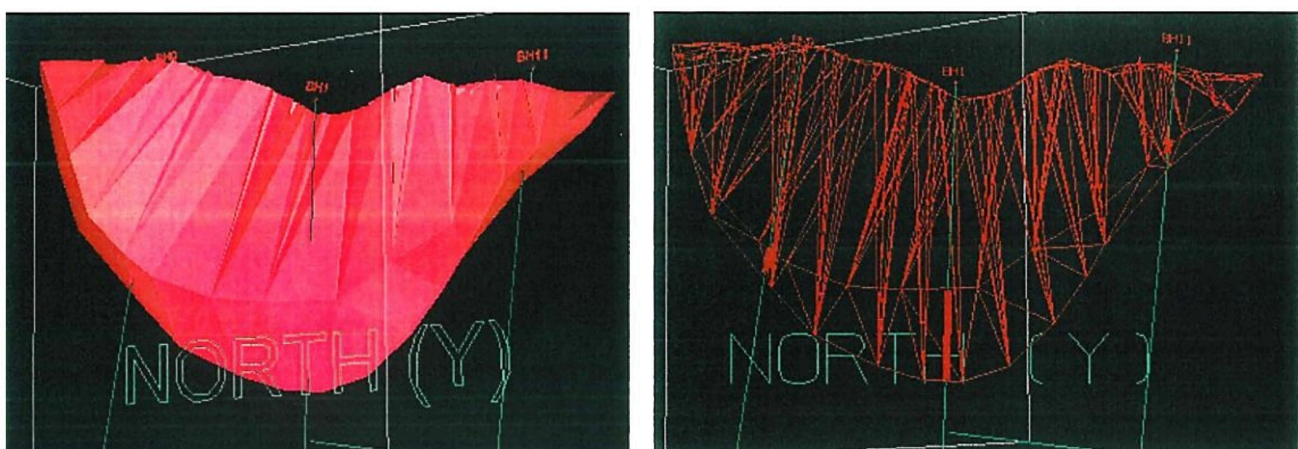
شکل ۱۰ - مدل سه‌بعدی هندسی کانسار؛ راست: Wireframe، چپ: مدل جامد
