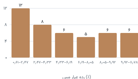
شکل ۸ - توزیع فراوانی عیار مس نمونه‌ها (۴۳ نمونه)
