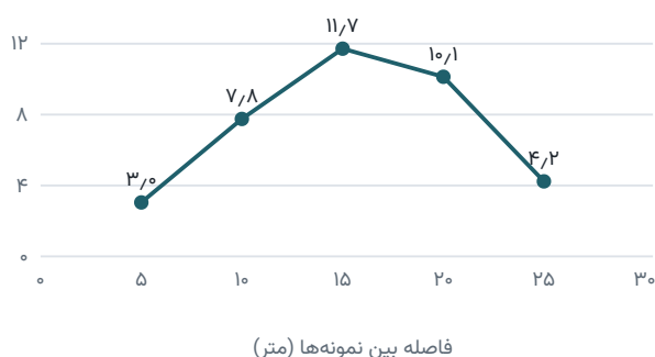
شکل ۹ - نیم‌تغییرنمای عیار مس (گام ۵ متر)
