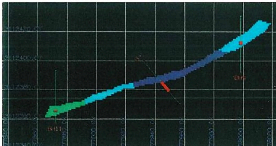
شکل ۷ - بلوک‌بندی کانسار و رنگ‌بندی بلوک‌ها بر اساس عیار مس (BH۱۱ در چپ، BH۹ در راست)
