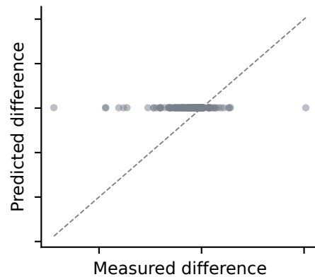
Token CNN
