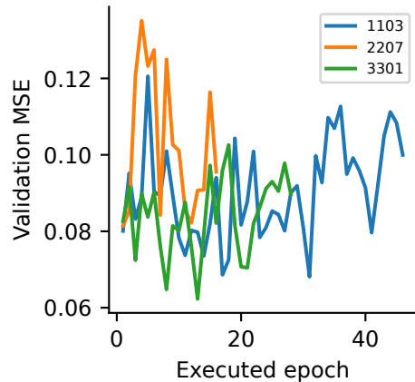
Token CNN
