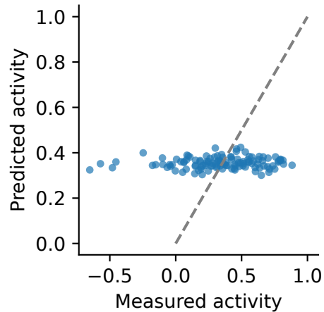
Token CNN
