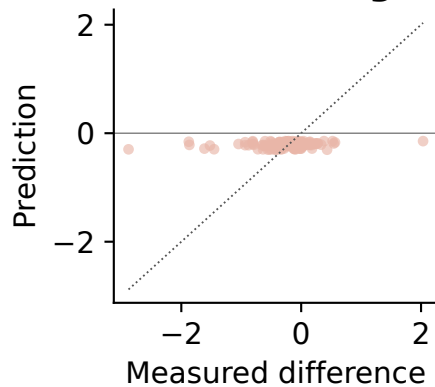
Pair no-msg
