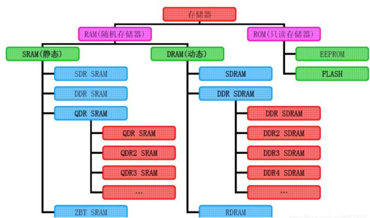
常见存储器分类图示
